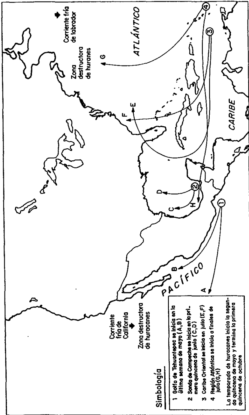
Fig 11 Regiones matrices de huracanes
