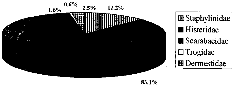
Figura 5. Proporción de las familias de Coleoptera necrófilos registrados a lo largo del año en los tres sitios de recolecta.
