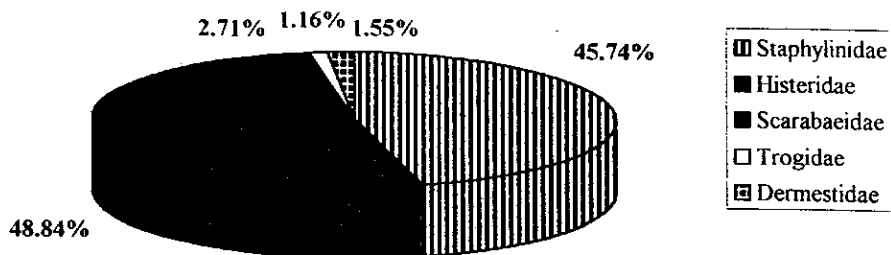
Figura 8. Proporción de Coleoptera necrófilos registrados a lo largo del año en el Espartal.
