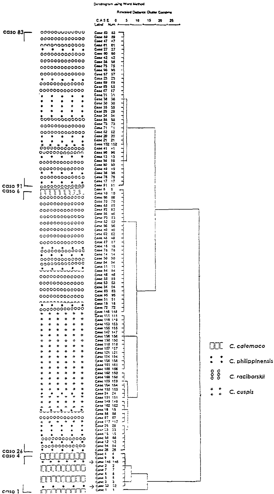
Fig. 5 Análisis de Conglomerados para el lago Chalchoapan considerando sólo caracteres cuantitativos. Los grupos formados por cada una de las especies de Cylindrospermopsis están señalados por patrones acotados en el lado derecho.
