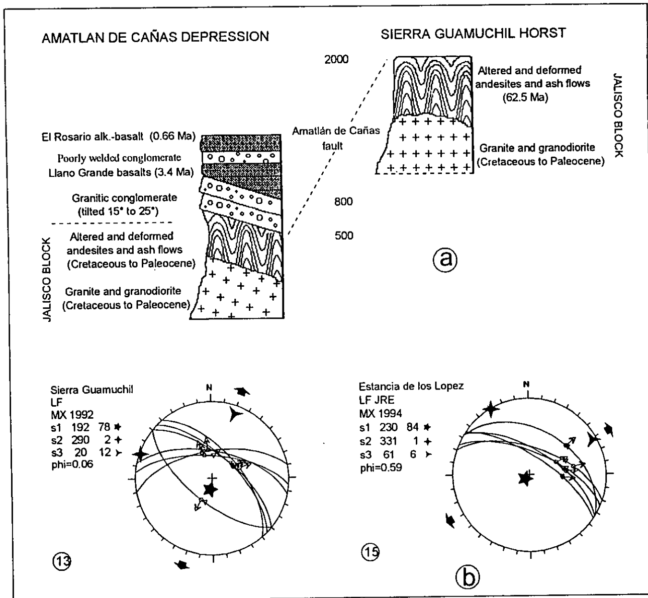
Fig. 4.6 (a) Estratigrafía generalizada del semigraben Amatlán de Cañas con elevaciones en metros (b) Estereogramas de las mesofallas en los sitios a lo largo de la falla Amatlán (ver Fig. 4.3 para la explicación y la figura 10 y Tabla 2 para localización)
