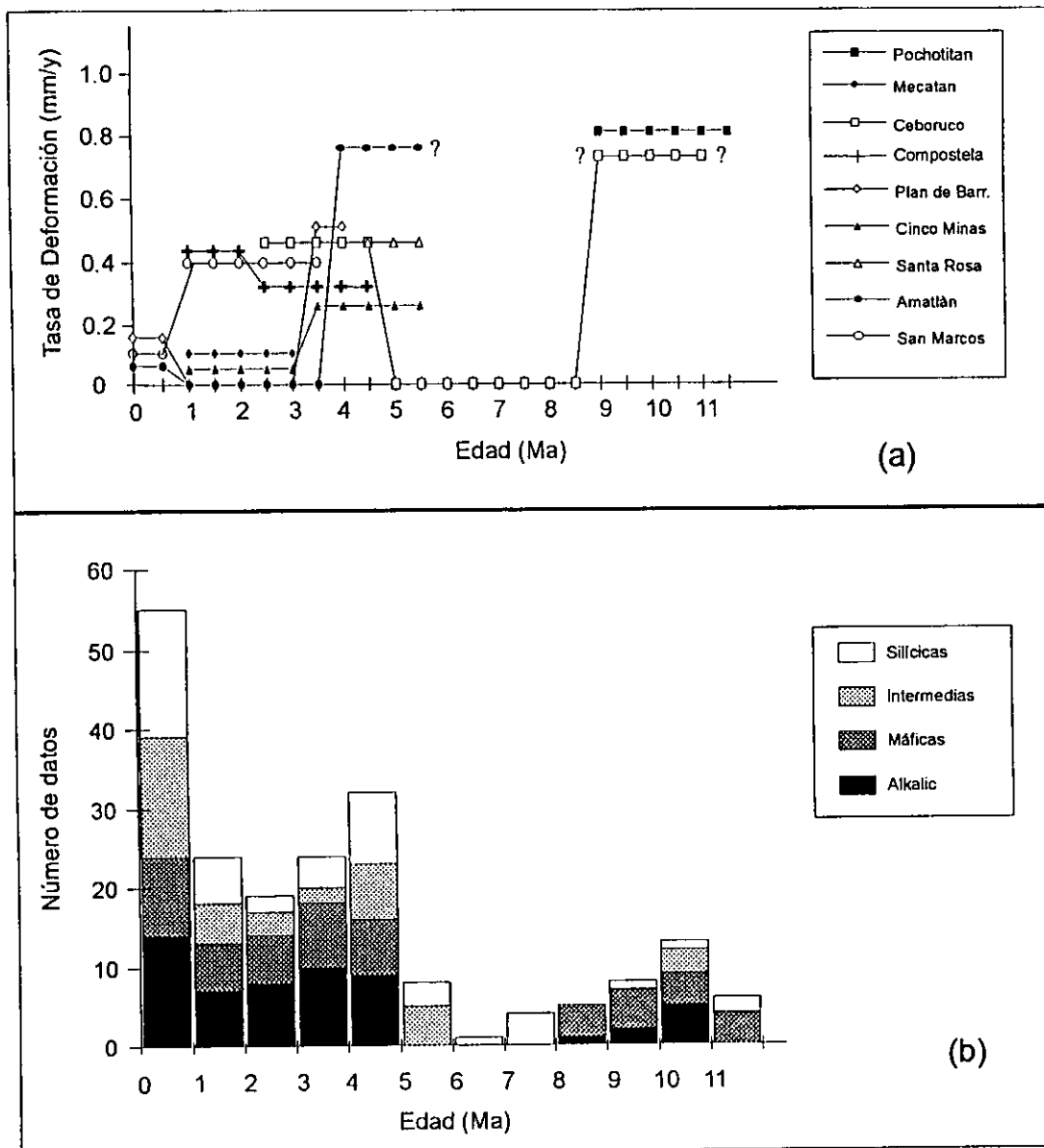
Fig. 4.11 (a) Tasa de deformación mínima para los istemas de fallas del rift Tepic-Zacoalco. Ver Tabla 4.1 para detalles. Los signos de interrogación indican valores solo parcialmente cotejados con datos radiométricos o geológicos. (b) Frecuencia y composición de rocas volcánicas datadas del Mioceno tardío al Presente en el área de estudio (datos de Ferrari et al., en prensa, Tablas 1 y 2). Silícicas=riolitas a dacitas; Intermedias=andesitas; Máfica=basaltos.
