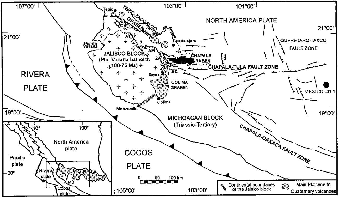
Fig. 2.1 Ambiente geodinámico del occidente de México. El bloque Jalisco está definido por el graben de Colima, la Trinchería Meso-Americana y el sistema Tepic-Zaoalco. Las zonas de falla Chapala-Oaxaca y Chapala-Tula tienen un sentido sinistral. TMVB, Faja Volcánica Trans-Mexicana. Adaptado de Harrison y Johnson (1988) y Rosas-Elguera et al. (1996).
