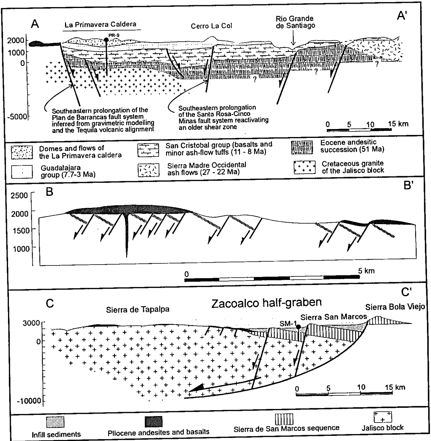
Fig. 3.6 Secciones geológicas de la parte oriental del graben Tepec-Zacoalco. (A) Sistema Plan de Barrancas-Santa Rosa. Observe que la cuenca es llenada por los basaltos San Cristobal y la forma lisica de la pequeña falla del sistema Santa Rosa-Cinco Minas, la cual bascula los depósitos lacustres del Plioceno temprano en la presa de Santa Rosa. (B) Semigraben de Ameca. La línea gruesa representa una ingnimita cretácica que muestra el basculameitno de la sucesión. (C) Interpretación propuesta del semigraber de Zacoalco. Observe la actitud diferente de la sucesión volcánica en el área de Guadalajara la cual no está basculada después del Plioceno tardío. Ver texto para discusión
