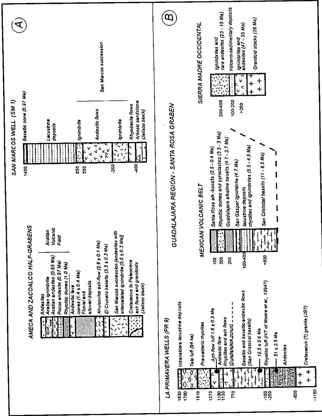
Fig. 3.3 Estratigrafía regional del área de estudio. (A) Estratigrafía simplificada de kis semigrabenes de Ameca y Zacualco El pozo San Marcos no esta a escala. (B) Las columnas estratigráficas a lo largo del río Santiago entre San Cristobal y la presa de Santa Rosa son comparadas con la SMO, al norte, y el pozo Primavera, al sur. En San Cristobal, solo la sucesión de la MVB esta expuesta; ella llena una cuenca (representada por la línea punteada), formada entre la SMO, cuya cima esta expuesta en la presa de Santa Rosa. Los números a la izquierda de las columnas son espesores en metros o elevaciones Las edades absolutas son referidas en el texto. (Ferrari et al., en prensa; este trabajo)
