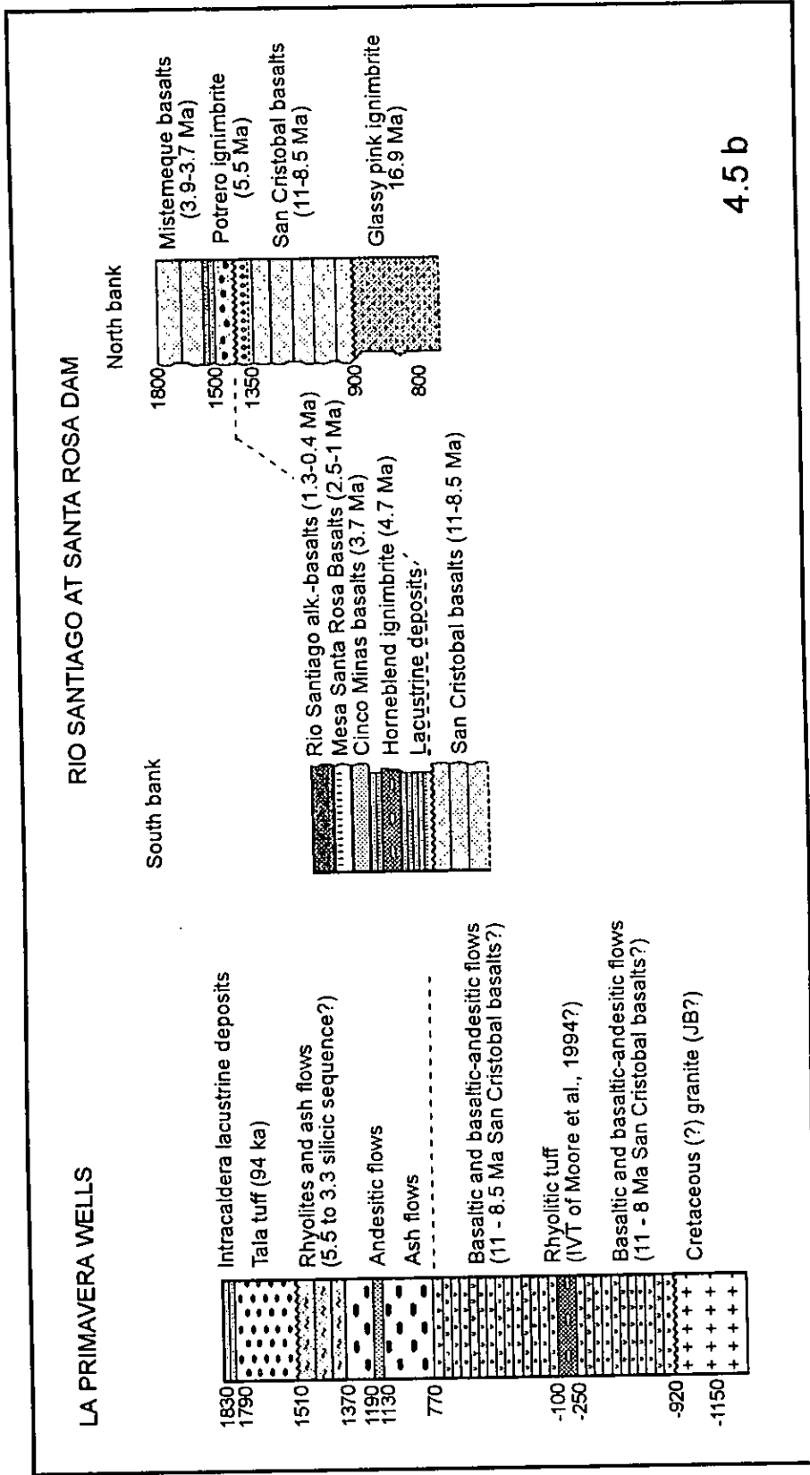
Fig. 4.5 (a) Mapa geoestructural del graben Plan de Barrancas-Santa Rosa. Se infiere que el sistema de fallas Plan de Barrancas continua por debajo del volcán Tequila y sus volcanes monogenéticos asociados, lo cual lo hace paralelo a la falla de Santa Rosa. Las edades están referidas en el texto. Los estereogramas de las mesofallas son como en la figura 4.3. (b) Estratigrafía generalizada de las márgenes norte y sur del Río Santiago a la altura de la presa de Santa Rosa. Elevaciones en metros
