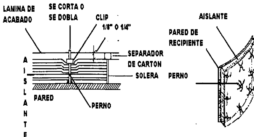
SUSPENSION FIJA DE AISLANTES EN RECIPIENTES
