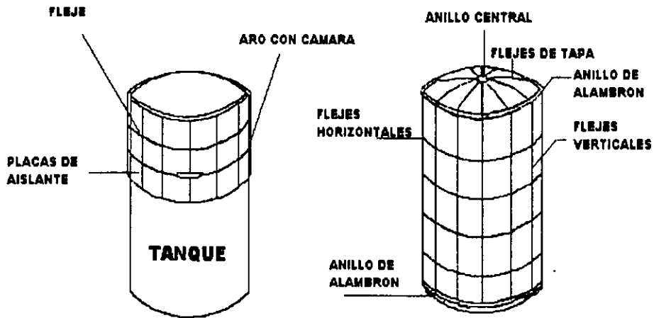
SISTEMA FLOTANTE (JAUJA DE PERICO)
