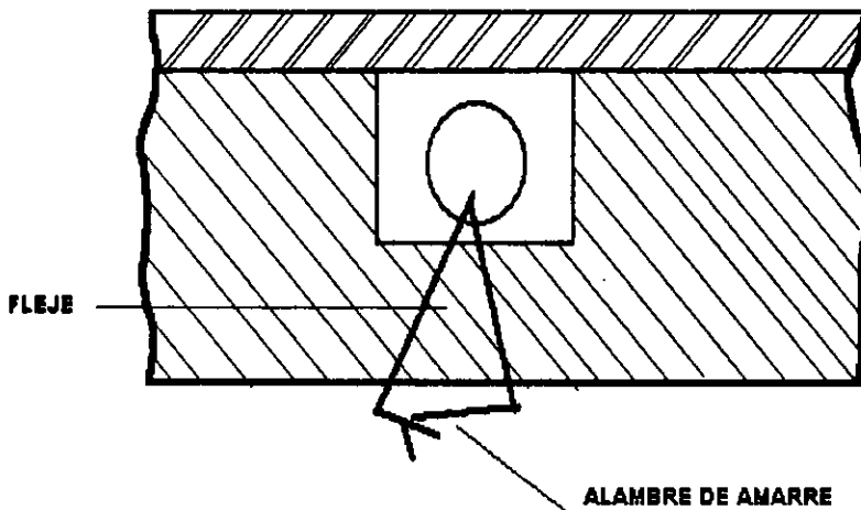
SOPORTE PARA EL AISLAMIENTO DE CABEZAS DE RECIPIENTES VERTICALES Y HORIZONTALES (ALTA TEMPERATURA)
