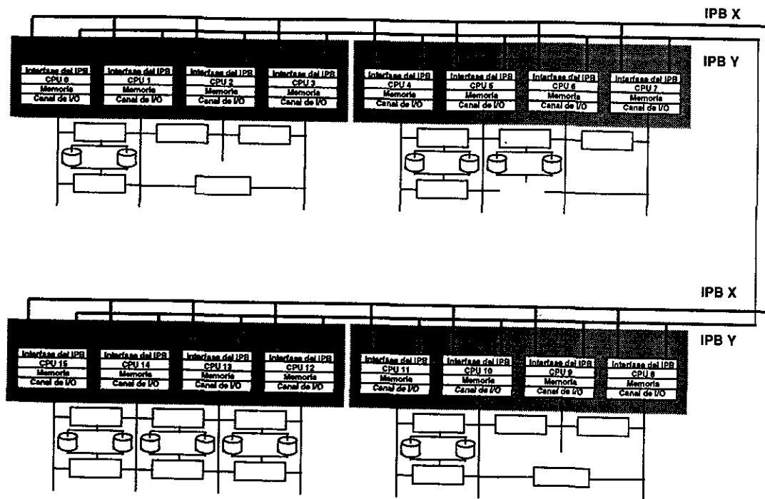
Figura 1-2. Un sistema NonStop de 16 procesadores.
