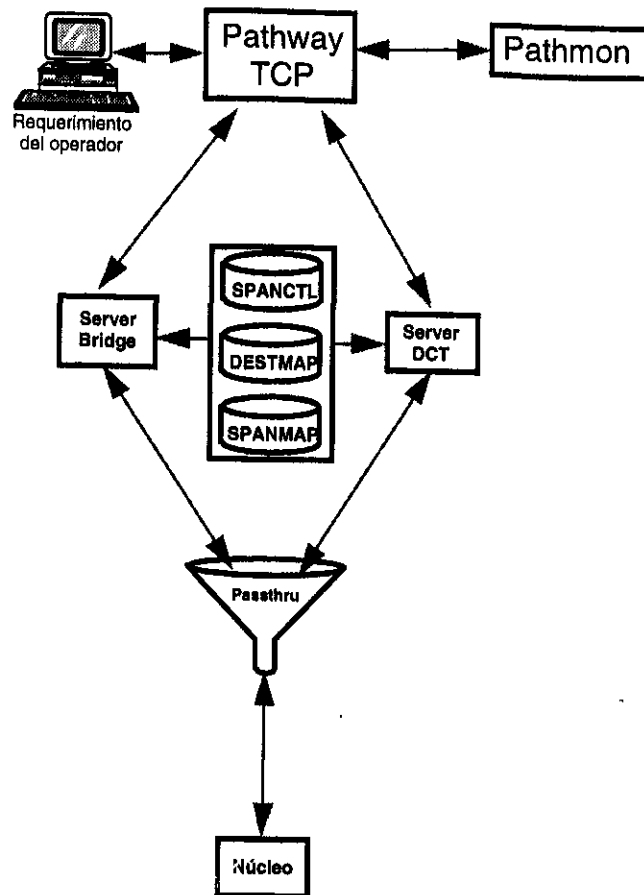
Figura 2-4. Interfase Usuario-BASE24.
