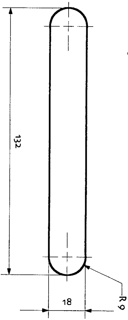
VISTA SUPERIOR
