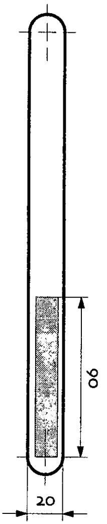
VISTA INFERIOR
