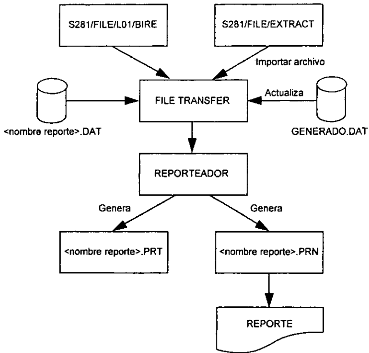
FIGURA 5.23. Flujo del Proceso de Impresión de Reportes.
