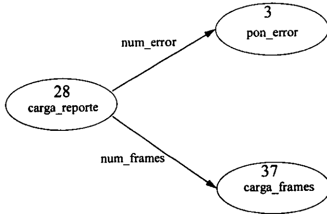
FIGURA 2.4.14. Carga Reporte.
