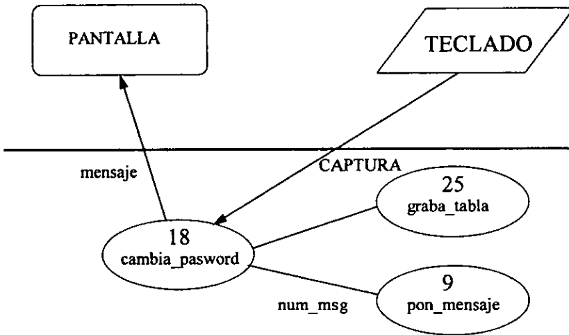
FIGURA 2.4.36. Cambia Password.
