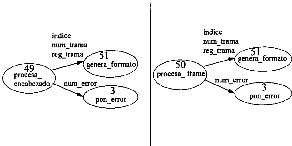
FIGURA 2.4.29. Procesa Reporte.
