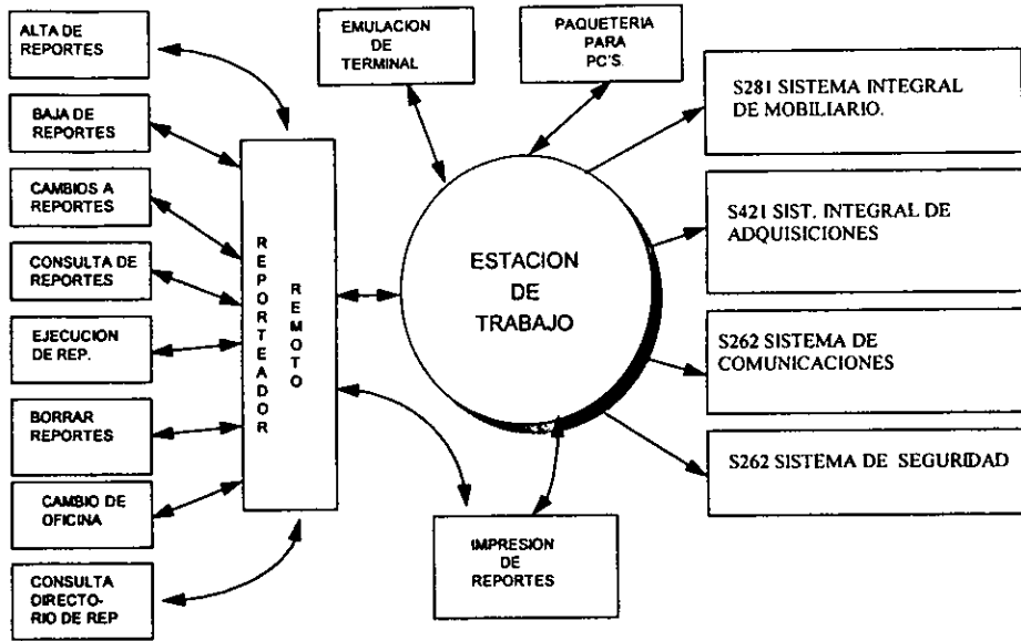
FIGURA 2.4. Esquema de la Estación de Trabajo-Reporteador Remoto.
