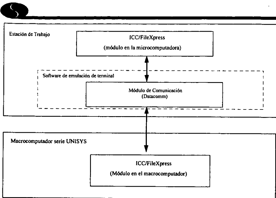
FIGURA 2.2. Relación software y hardware de los elementos de ICC/FileXpress.
