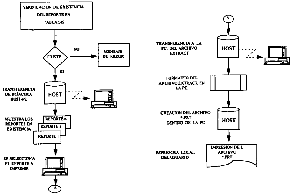
FIGURA 3.5. Proceso efectuado para la Impresión Remota de Reportes.
