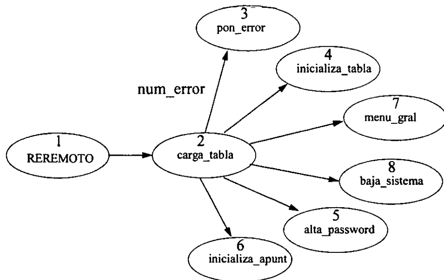
FIGURA 2.4.2. Reporteador Remoto.
