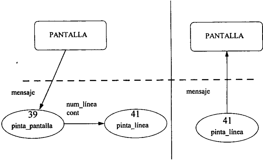
FIGURA 2.4.22. Controla Pantalla.
