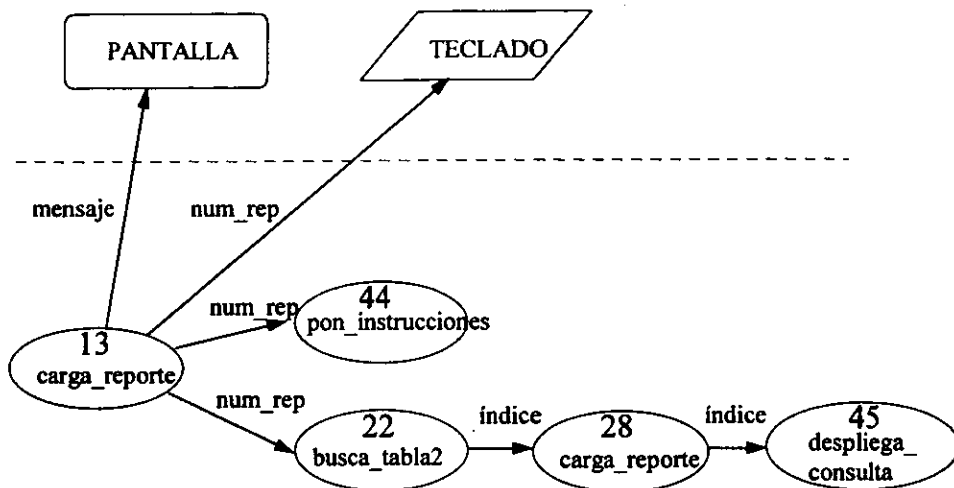
FIGURA 2.4.26. Carga Reporte.
