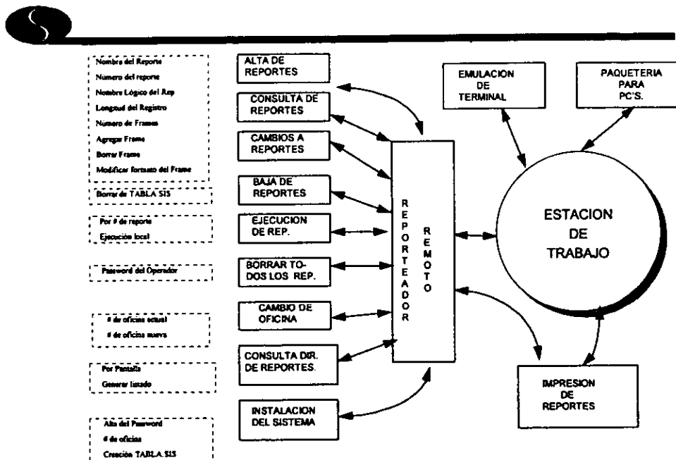
FIGURA 3.1. Esquema de la Estación de trabajo - Reporteador Remoto.
