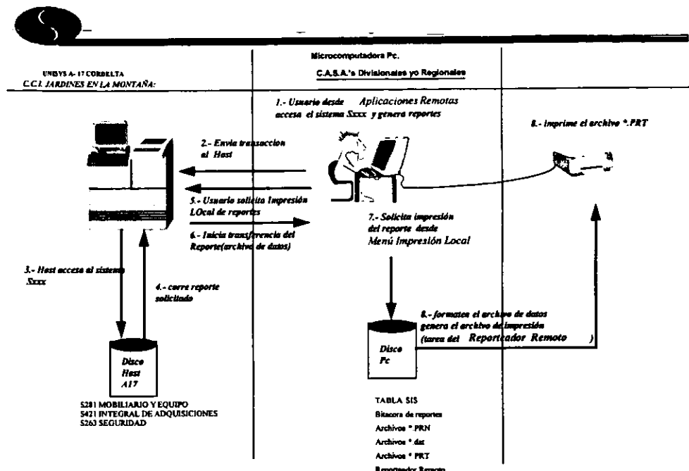
FIGURA 3.3. Diseño del Flujo de Impresión del Reporteador Remoto.
