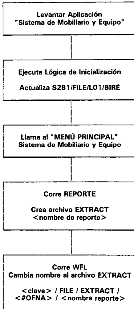
FIGURA 5.12. Diagrama de Bloques del Sistema (Reporteador).
