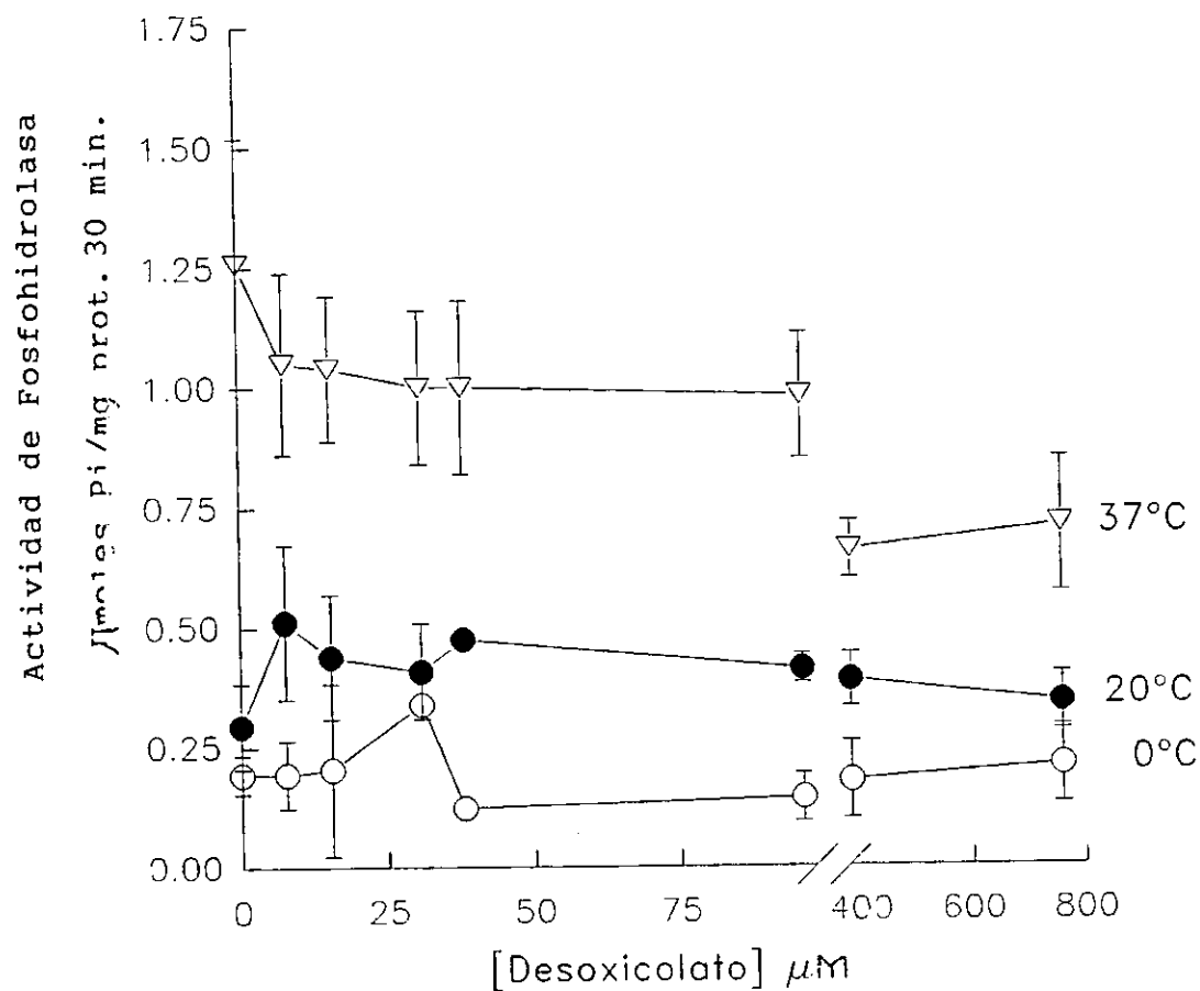
FIGURA 20: EFECTO DE DESOXICOLATO SOBRE LA REACCION DE GLUCOSA-6-FOSFOHIDROLASA A DIFERENTES TEMPERATURAS CON \text{CdI}_2
