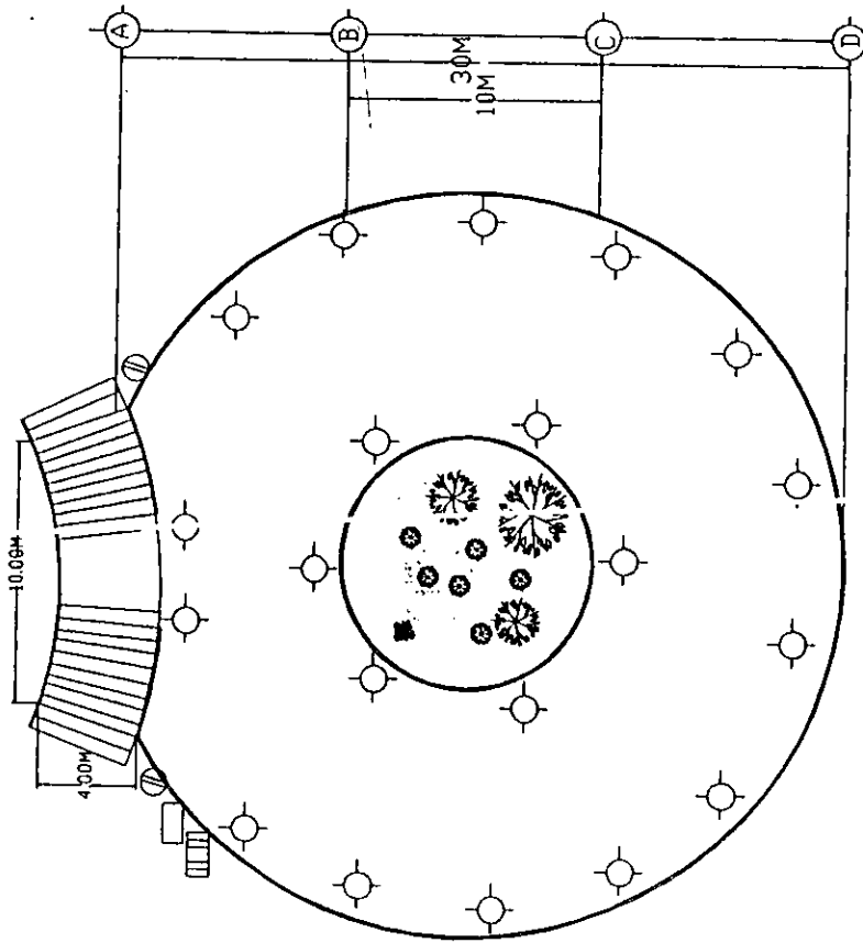
PLANTA DE INSTALACION ELECTRICA DEL COMEDOR
