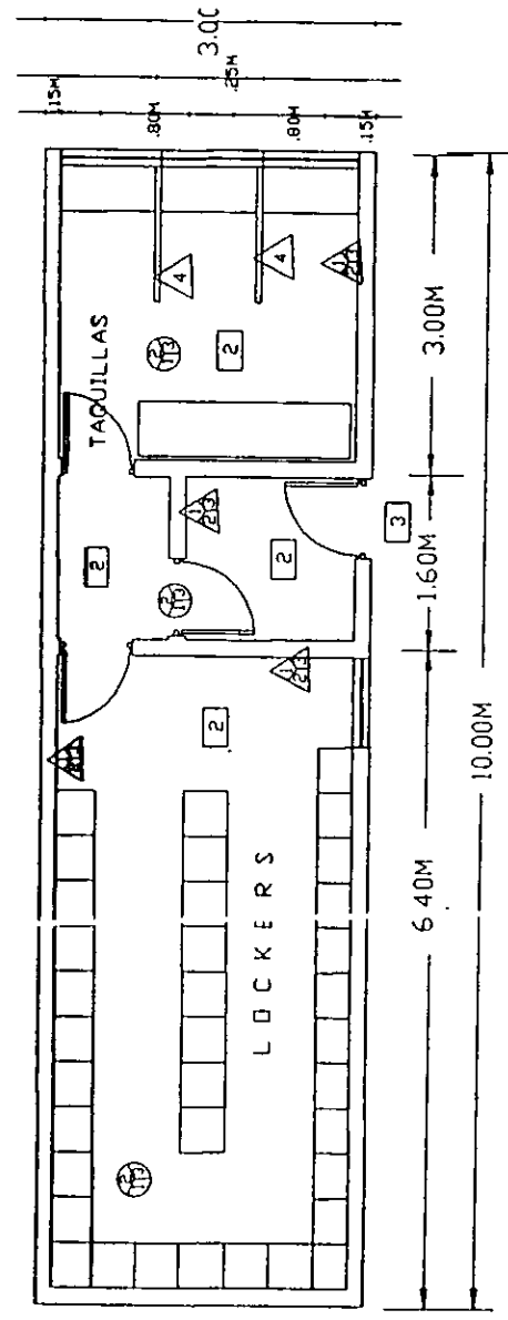
PLANTA DE ACABADOS DE TAQUILLAS Y LOCKERS
