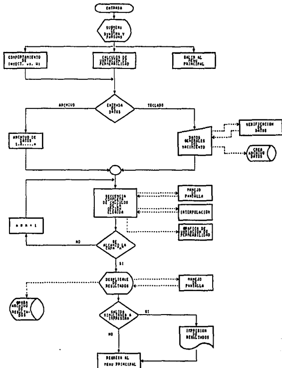
Fig. 4.5. DIAGRAMA DE BLOQUES DEL METODO DE DYKSTRA - PARSONS
