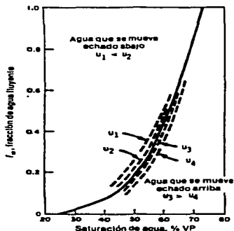
Fig. III.4 Efecto del gasto sobre la curva de flujo fraccional, caso mojado por agua, yacimiento inclinado.
