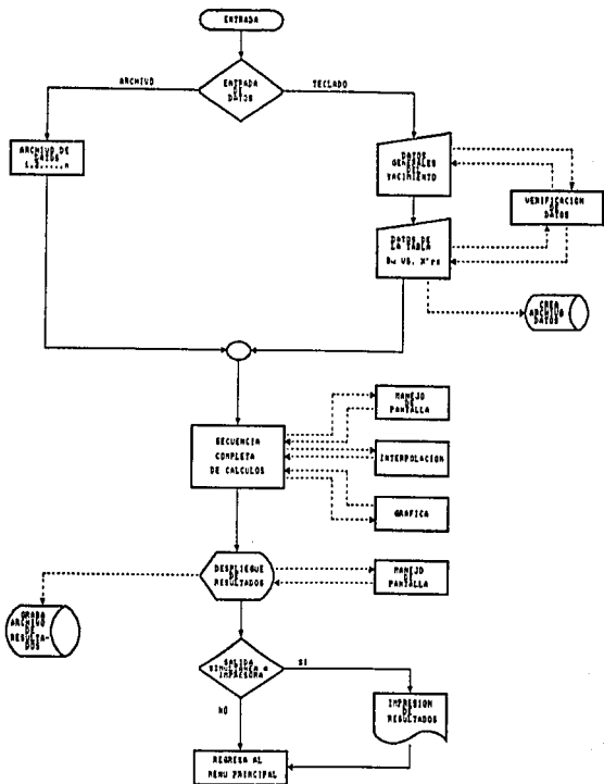
Fig. 4.3. DIAGRAMA DE BLOQUES DEL METODO DE WELGE
