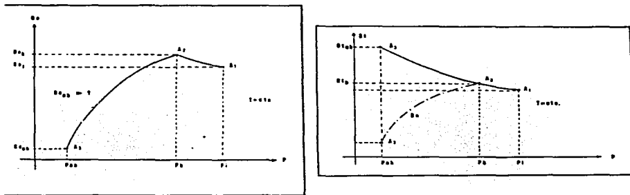
Fig. 1.8.- Comportamiento B_o , B_t vs Presión.
