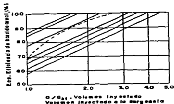
Fig. III.18 INCREMENTO DE LA EFICIENCIA DE BARRIDO AREAL DESPUES DE LA SURGENCIA.
