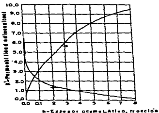
Fig. III.10 Distribución de la permeabilidad y la capacidad
