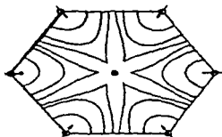
Fig. II.12 BOSQUEJO DE TRES FRENTES DE FLUJO OBSERVADO EN UN ARREGLO DE SIETE POZOS NORMAL, DONDE LOS ELEMENTOS SON OBTENIDOS DE MODELOS ELECTROLITICOS.
