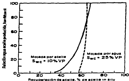
FIG. III.3 EFECTO DE LA MOJABILIDAD DE LA ROCA SOBRE EL COMPORTAMIENTO DE LA RECUPERACION DE ACEITE POR INYECCION DE AGUA.
