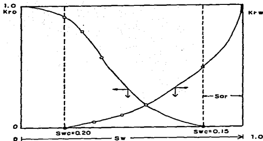
Fig. 1.2.- Gráfica de Permeabilidades Relativas Agua-Aceite.
