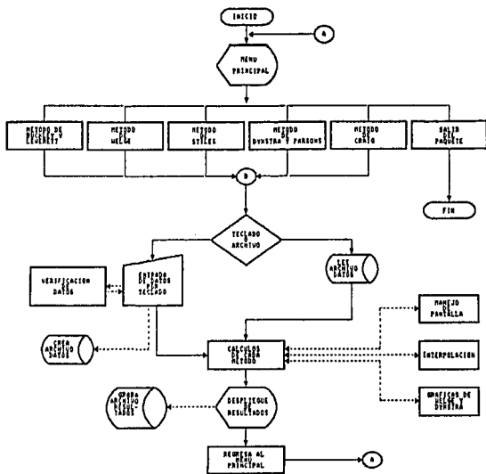
Fig. 4.1. DIAGRAMA DE BLOQUES DEL SISTEMA DE COMPUTO
