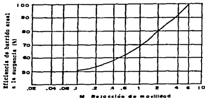
Fig. III.17 EFICIENCIA DE BARRIDO AREAL A LA SURGENCIA, DE UN MODELO DE CINCO POZOS.
