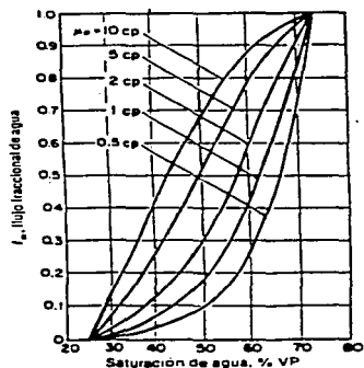
Fig. III.1 EFECTO DE LA VISCOSIDAD DEL ACEITE SOBRE LA CURVA DE FLUJO FRACCIONAL, ROCA FUERTEMENTE MOJADA POR AGUA.
