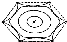
Fig. II.13 BOSQUEJO DE TRES FRENTES DE FLUJO OBSERVADO EN UN ARREGLO DE SIETE POZOS INVERTIDO, DONDE LOS ELEMENTOS SON OBTENIDOS DE MODELOS ELECTROLITICOS.
