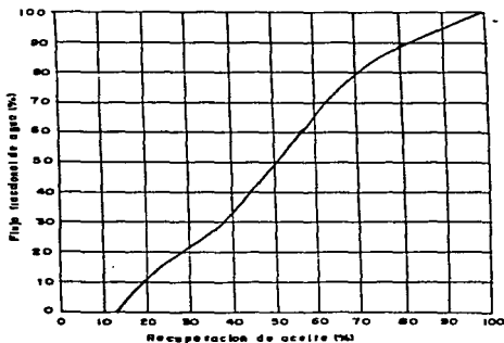
Fig. III.12 FLUJO FRACCIONAL DE AGUA VS. RECUPERACION
