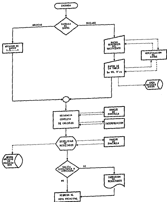
Fig. 4.2. DIAGRAMA DE BLOQUES DEL METODO DE BUCKLEY - LEVERETT
