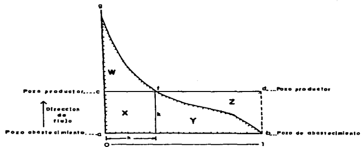
Fig. III.11 Secciones básicas e ilustración esquemática del frente de flujo.
