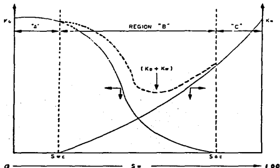
Fig. 1.1.- Permeabilidades Efectivas para un Sistema Aceite-Agua
