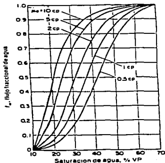
Fig. III.2 EFECTO DE LA VISCOSIDAD DEL ACEITE SOBRE LA CURVA DE FLUJO FRACCIONAL, ROCA FUERTEMENTE MOJADA POR ACEITE.
