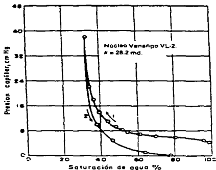
Fig (1.6.a) Características de la Pc durante : (1) drene y (2) imbibición
