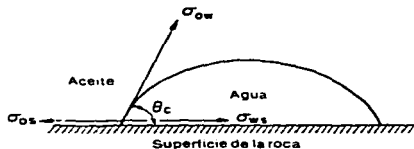
Fig. 1.7 .- Mojabilidad de un sistema aceite-agua-sólido
