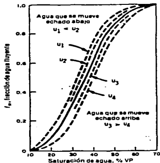
Fig. III.5 Efecto de gasto sobre la curva de flujo fraccional, caso mojado por aceite, yacimiento inclinado.
