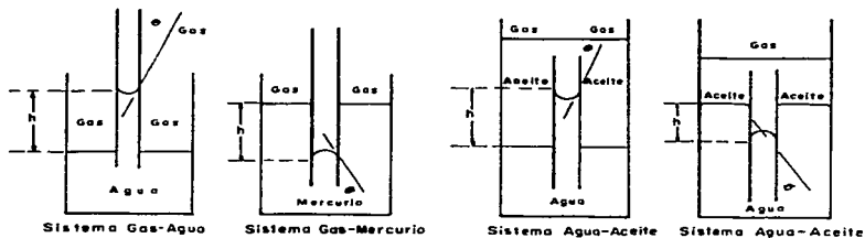
Fig. 1.3 . Ilustración de las fuerzas capilares.
