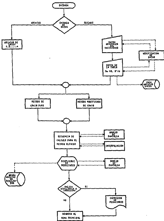
Fig. 4.6. DIAGRAMA DE BLOQUES DEL METODO DE CRAIG
