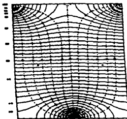
Fig. II.11 DISTRIBUCION DE PRESIONES EN ARREGLO DE POZOS EN LINEA ALTERNA.
