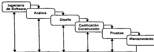
Fig.2.6 Modelo SDLC
