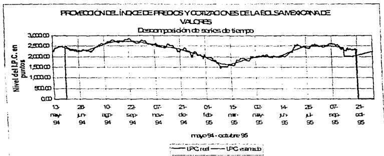
Figura 2.9. Pronóstico del IPC con el método de descomposición de series de tiempo, nov. 95.
