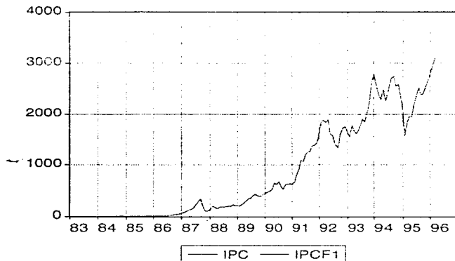
Figura 4.16.: Pronóstico del I.P.C. por el periodo de octubre 1995 - marzo 1996.
