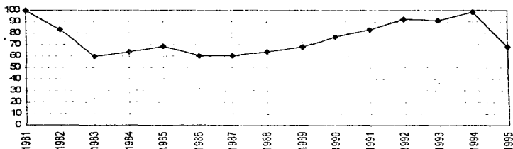
Figura 1.11.: Gráfica de una serie de tiempo cíclica. Serie de la inversión en México.
