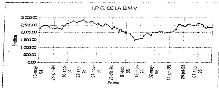
Figura 2.1.: Índice diario de la Bolsa Mexicana de Valores, mayo 94 - octubre 95
