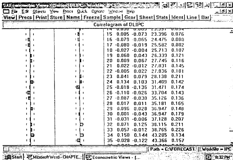
Figura 4.6.: Correlograma de la variable DLIPC con 36 rezagos.
