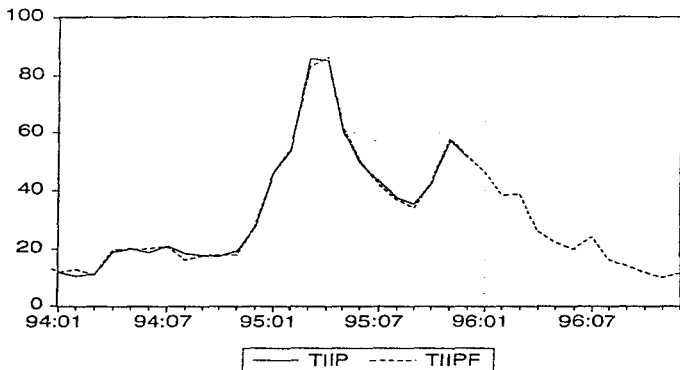
Figura 3.17.: Gráfica del TIIP y la TIIP pronosticada
