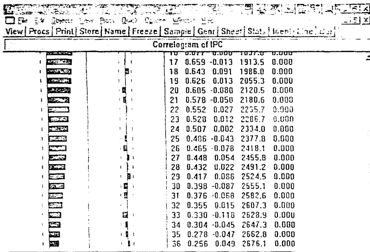
Figura 4.2: Correlograma del I.P.C. de la B.M.V. con 36 rezagos
