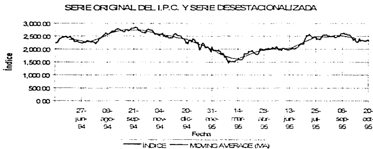
Figura 2.6.: Serie original y desestacionalizada del Índice diario de la Bolsa Mexicana de Valores, mayo 94 - octubre 95
