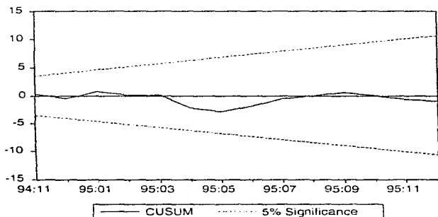
Figura 3 15.. Resultados de la prueba CUSUM
