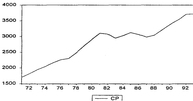
Figura 1.9.: Gráfica de una serie de tiempo con tendencia. Serie del consumo privado en México.
