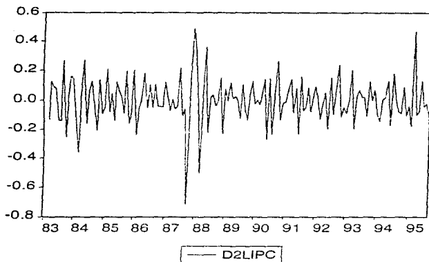
Figura 4.7 : Gráfica de las segundas diferencias de la variable LIPC, (D2LIPC)
