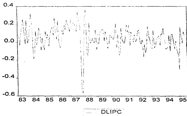
Figura 4.5.: Gráfica de las primeras diferencias de la variable LIPC, (DLIPC).
