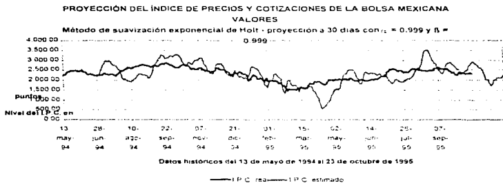
Figura 2.4: Pronóstico del Índice diario de la Bolsa Mexicana de Valores, noviembre 95.
