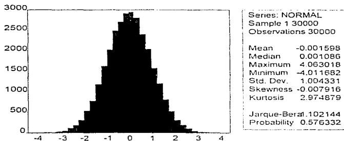
Figura 1.1.: Distribución de números aleatorios con media 0 y varianza 1. Muestra de 30,000 números.
