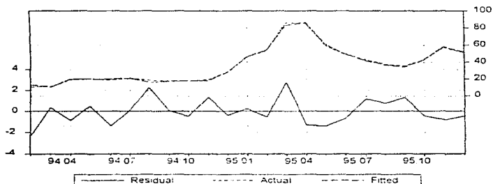
Figura 3.3.: Resultados de la regresión con la TIP
