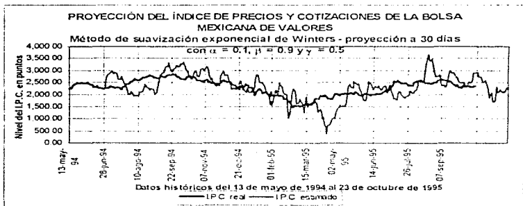
Figura 2.5.: Pronóstico del índice diario de la Bolsa Mexicana de Valores, noviembre 95.
