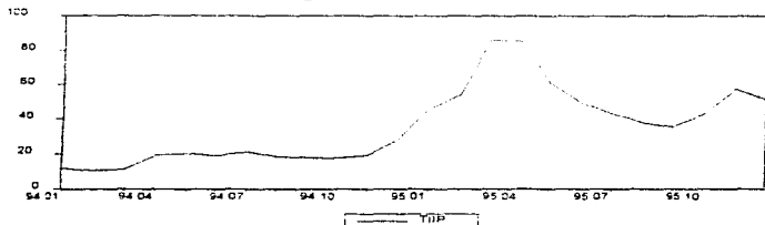
Figura 3.1.: Evolución de la TIIP por el periodo 1994 1995.
