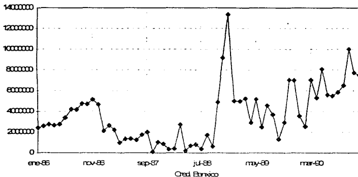
Figura 1.10.: Gráfica de una serie de tiempo con estacionalidad. Serie del crédito vía Banxico.
