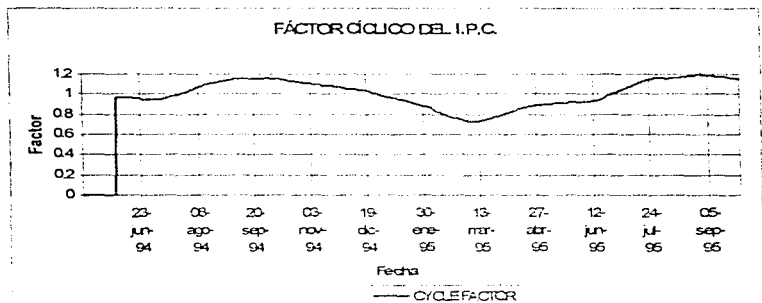
Figura 2.8.: Factor cíclico del Índice diario de la Bolsa Mexicana de Valores, mayo 94 - octubre 95.
