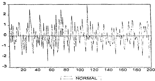
Figura 1.8.: Gráfica de una serie de tiempo estacionaria, con media y varianza constantes. Serie normal con media cero y varianza 1.
