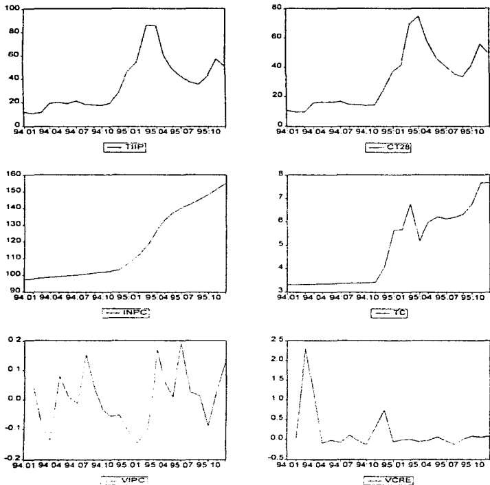
Figura 3.1. Evolución de la TIIP, CETES, INPC, TC, variación del IPC y del CREDITO por el periodo 1994 1995
