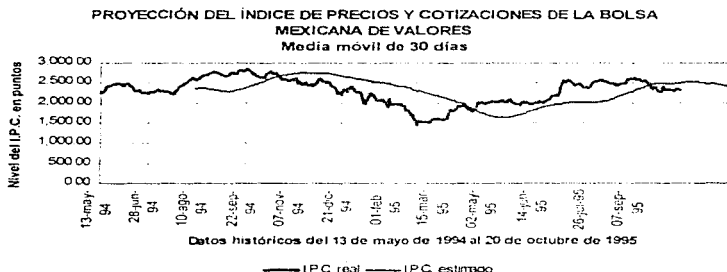
Figura 2.2.: Pronóstico del Índice diario de la Bolsa Mexicana de Valores, noviembre 95.
