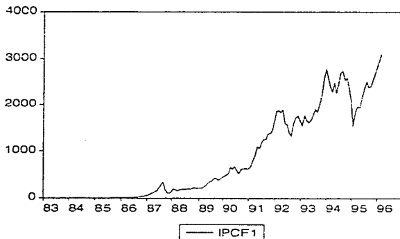
Figura 4.17.: Pronóstico del I.P.C. por el periodo de octubre 1995 - marzo 1996.
