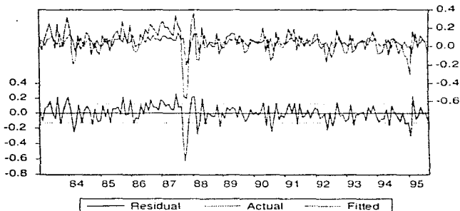
Figura 4.11.: Mapeo de los valores reales, estimados y los residuos de la regresión.
