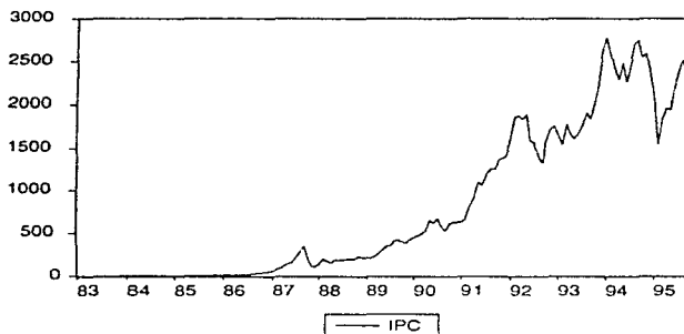
Figura 4.1.: Gráfica del I.P.C. de la B.M.V. Datos mensuales 1983 - 1995.
