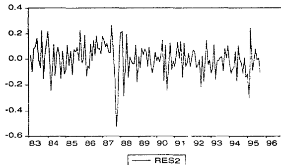
Figura 4.14.: Grafica de los residuos de las regresiones de los modelos C MA(1) I1 y C MA(1) I2. RES1 y RES2, respectivamente.
