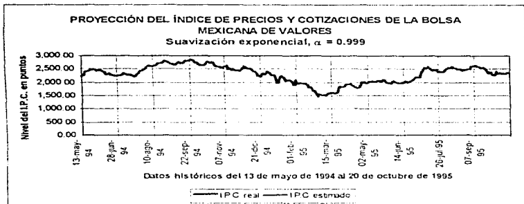
Figura 2.3.: Pronóstico del índice diario de la Bolsa Mexicana de Valores, noviembre 95.
