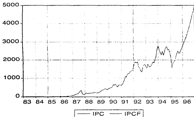
Figura 4.15 · Pronóstico del I.P.C. por el período de octubre 1995 - diciembre 1996.
