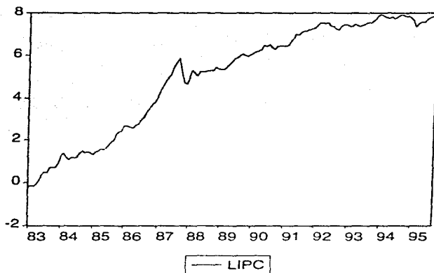
Figura 4.3.: Gráfica del logaritmo natural del I.P.C.
