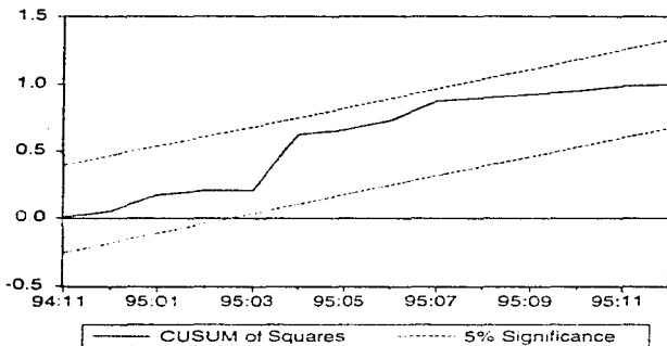
Figura 3.16 . Resultados de la prueba CUSUM 2
