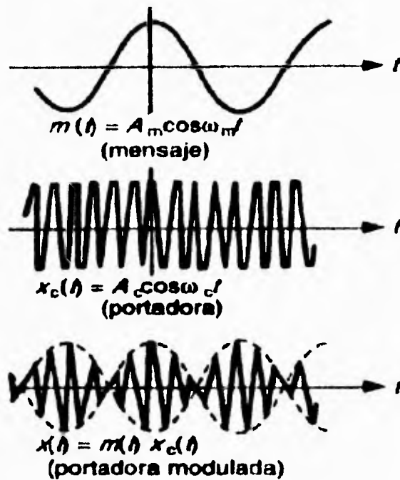
Figura 3.2 Modulación en Amplitud
