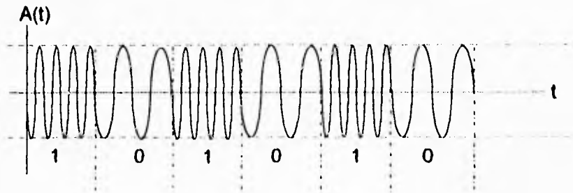
Figura 3.6 Modulación en frecuencia
