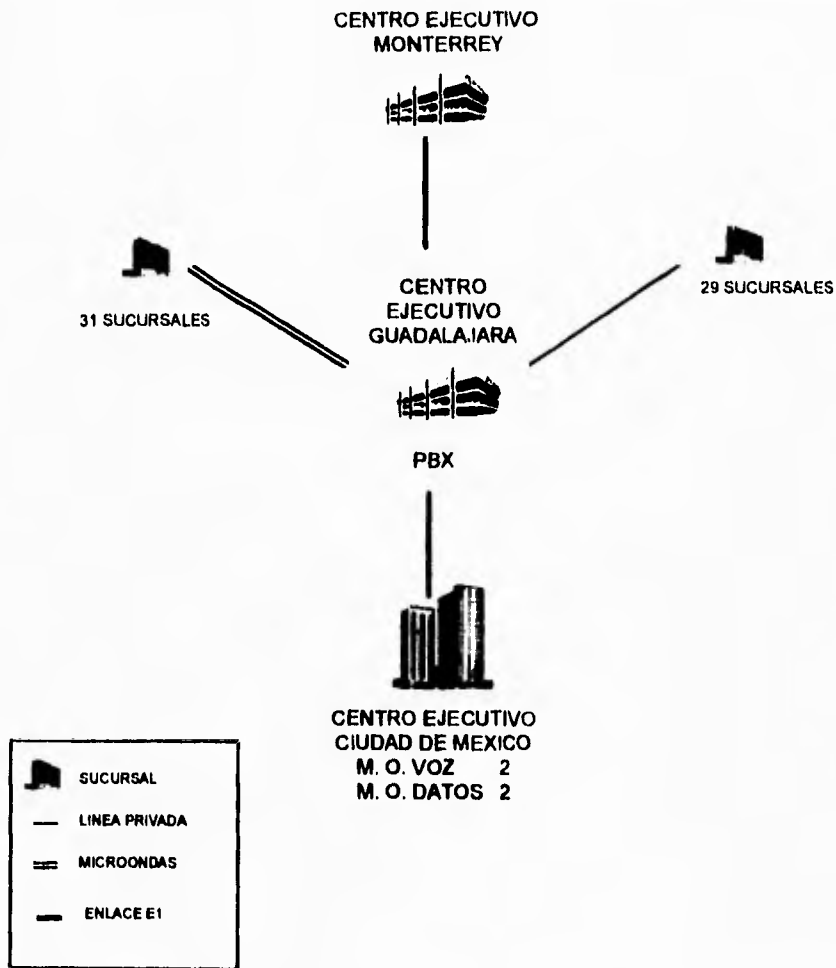
Figura 4.5 Centro ejecutivo Guadalajara
