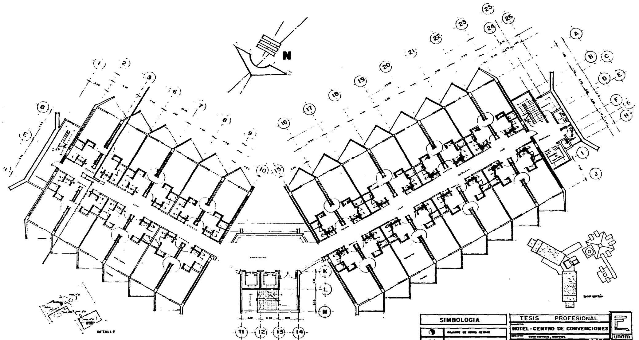
planta tipo / habitacion sencilla ESC. 1/100
