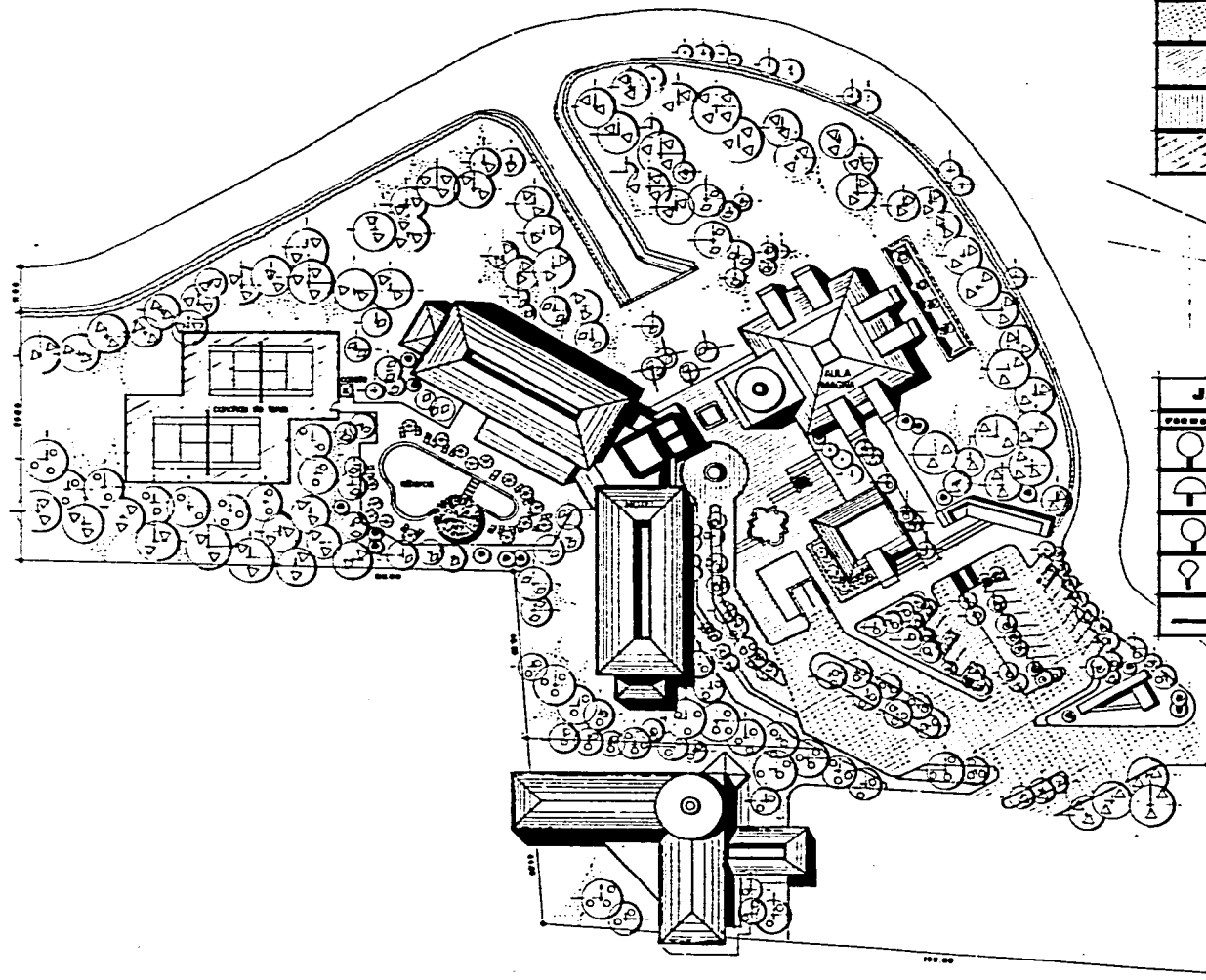
planta de conjunto ESC. 1:500
