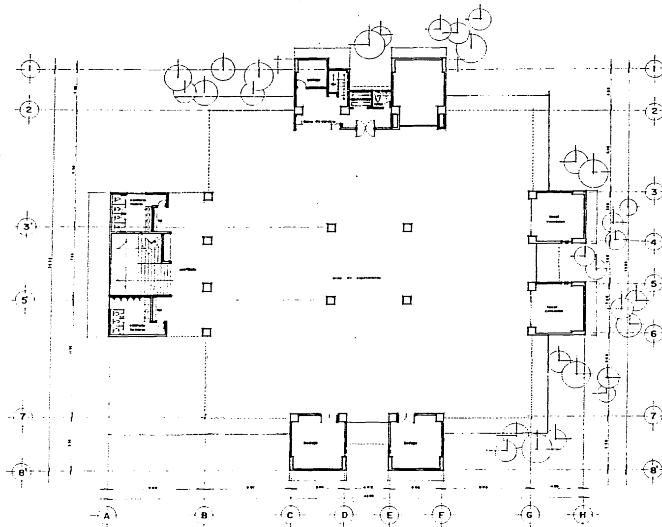
planta area de exposiciones ESC. 1:100
