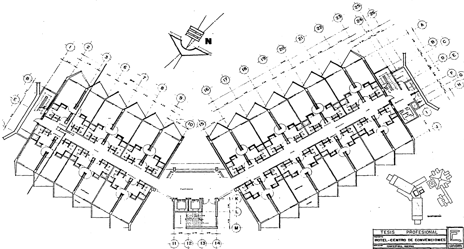
planta tipo / habitación sencilla ESC. 1:100
