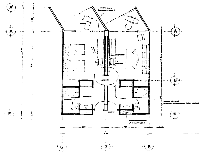
planta tipo habitacion sencilla ESC 1:50
