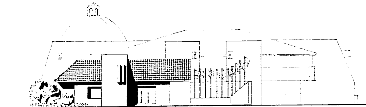
elevación principal administración - aula magna ESC 1:100
