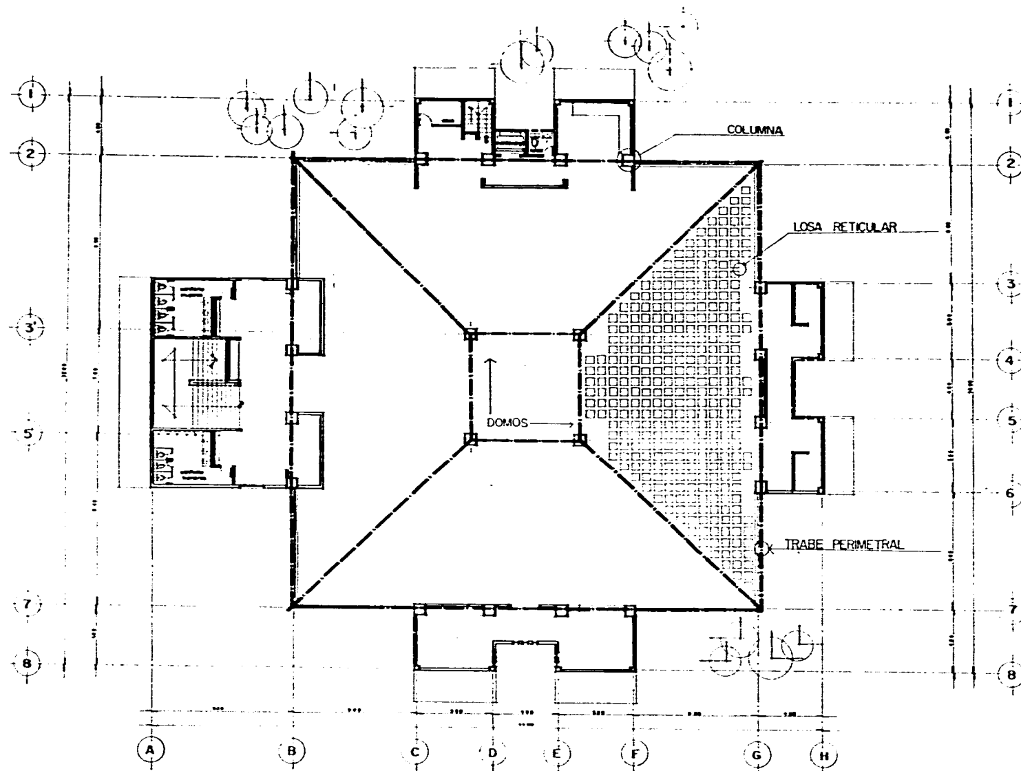
planta aula magna ESC. 1:100
