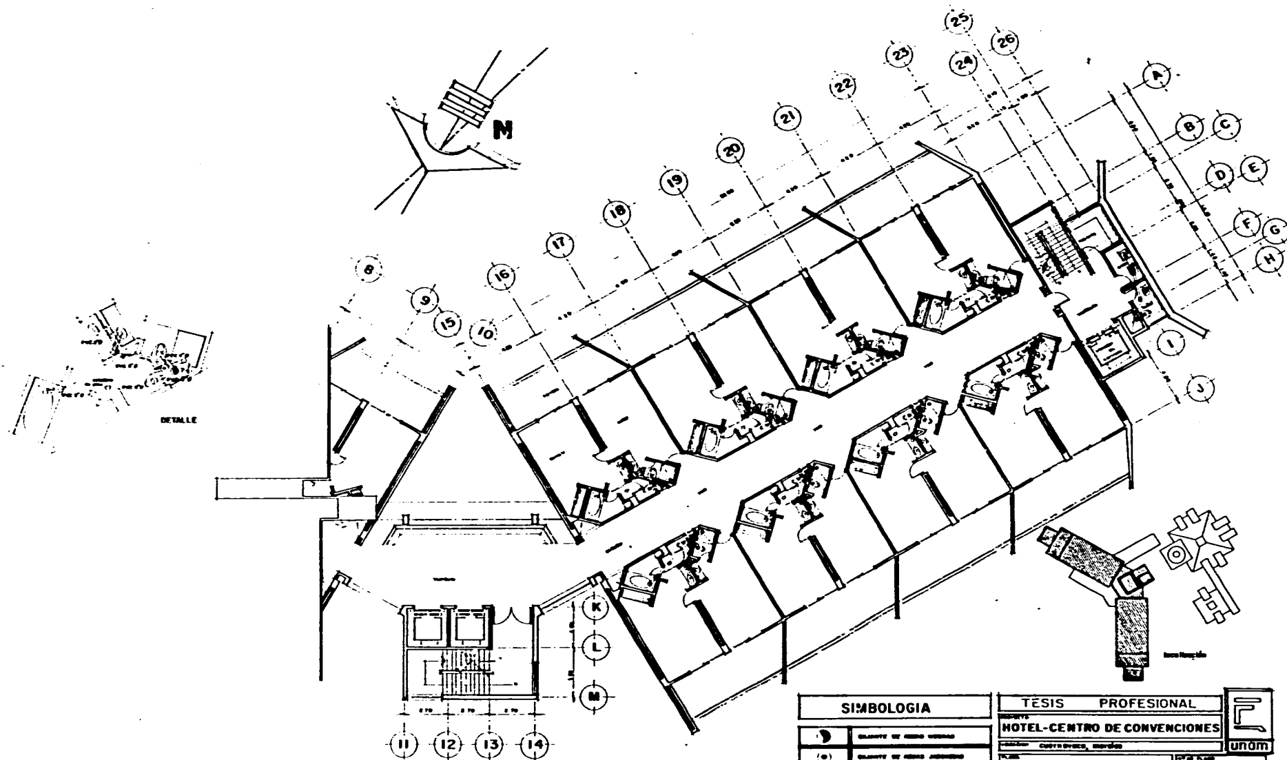
Planta tipo / habitacion suite SC 1:100
