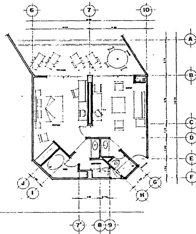
planta tipo habitacion suite ESC 1:50
