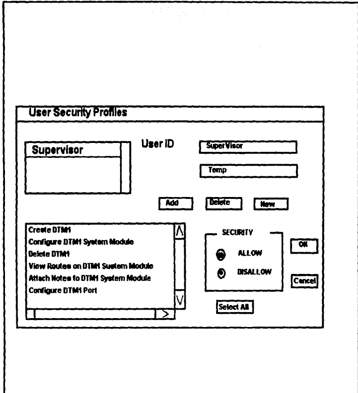
Figura III.3.6-3. Cuadro de archivos de seguridad de usuarios.
