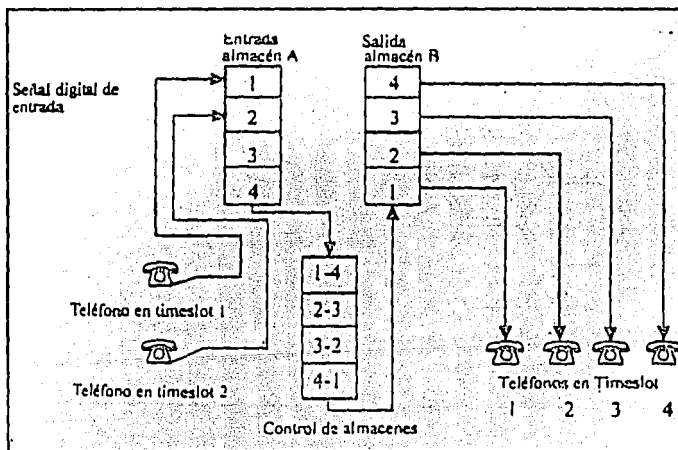
Figura 1.3.2-1 Conmutador de Tiempo, utiliza timeslots para conectar cualquier entrada a cualquier salida.
