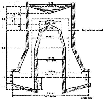
FIGURA 17/G.703
