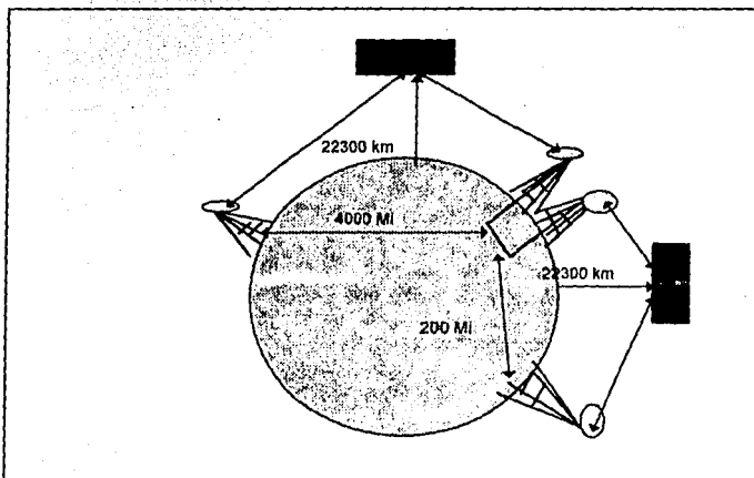
Figura I.1.5-12. Distancias involucradas en una comunicación por satélite.
