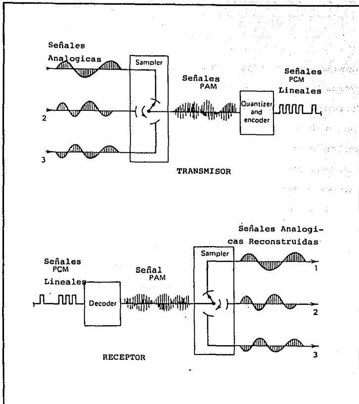
Figura 1.1.3-4. Analogía simplificada de la formación de una onda PAM.
