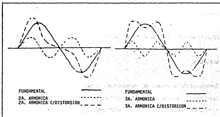
Figura I.2.4-1. Señal distorsionada.
