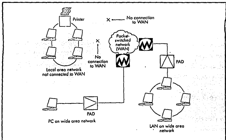
Figura III.2-2. En la parte izquierda se encuentra una LAN mientras la PC que se encuentra en la parte inferior izquierda forma parte de una WAN (Wide Area Network). En la parte derecha se encuentra una LAN conectada a una WAN vía una PC que se denomina "gateway".
