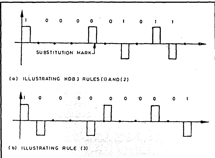
Figura 1.2.5-11. Código de línea HDB3.
