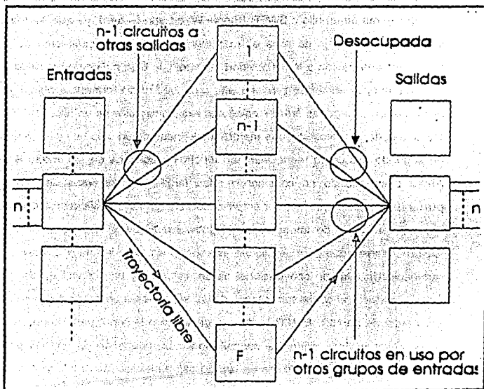
Figura 1.3.2-7 Conmutador con n entradas que tiene n-1 circuitos ocupados. A la salida también hay n-1 circuitos ocupados; para evitar el bloqueo siempre debe existir una trayectoria disponible
