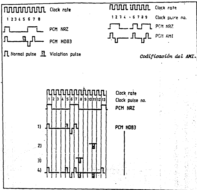
Figura 1.2.5-13. Codificación HDDB3 y AMI.
