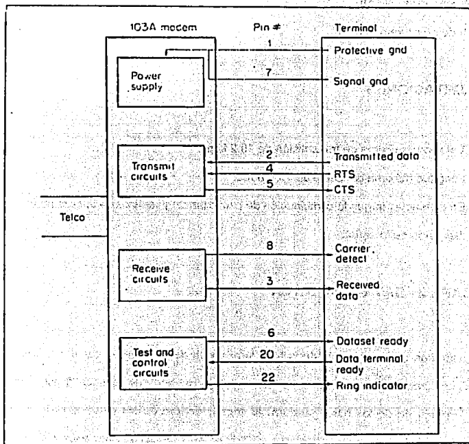
Fig. I.2.6-8 Ejemplo de interfaz DTE-DCE.
