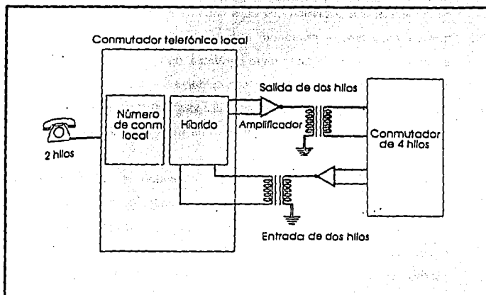
Figura I.3.2-8. La transmisión por cuatro hilos permite amplificación independiente de transmisión y recepción.
