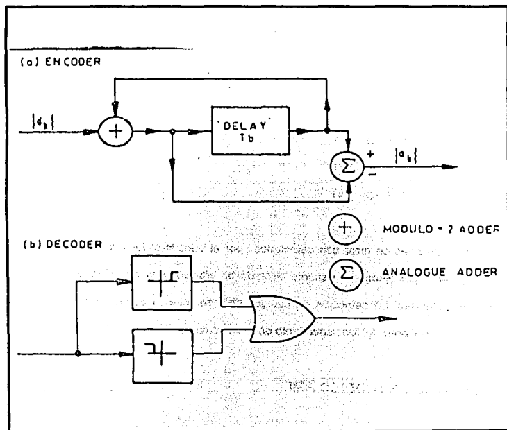
Figura I.2.5-9. Codificación y decodificación para el código de línea AMI.
