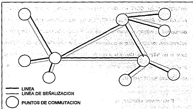
Figura I.1.6-3 Modo de señalización CCIS Asociado.
