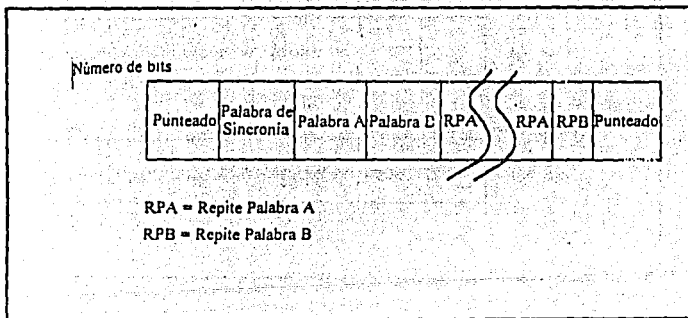
Figura 1.3.3-7. Formato general de un mensaje hacia un móvil.
