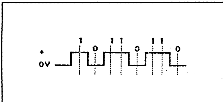
Figura 1.2.5-1. Señalización Unipolar no-retorno a cero. La corriente o voltaje no regresa al valor cero entre bits "unos" adyacentes.
