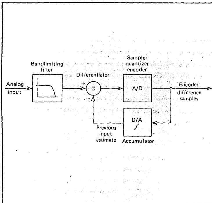
Figura I.1.3-14. Diagrama de bloques funcional del PCM Diferencial.
