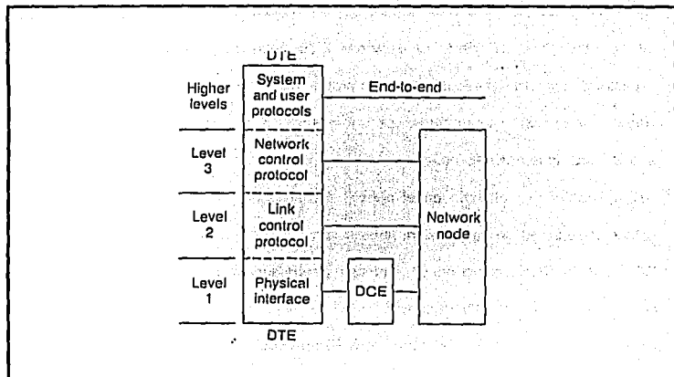
Figura I.1.11-7. Niveles bajos del protocolo de interface para redes.
