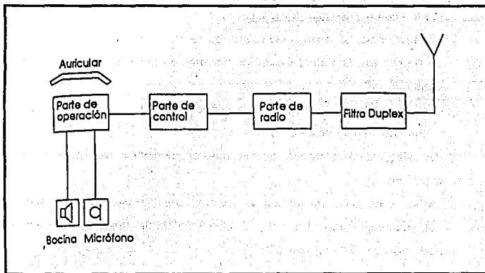
Figura I.3.4-2 Unidades Funcionales de la Estación Móvil
