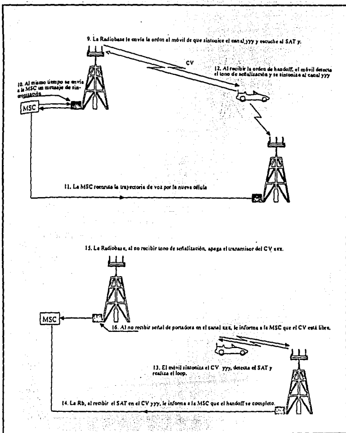
Figura 1.3.3-5. Finalización del Handoff
