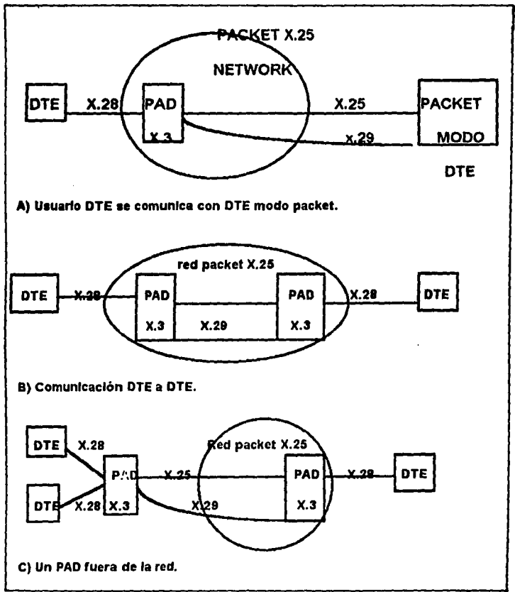
Figura I.1.10-1. PADs y X.25
