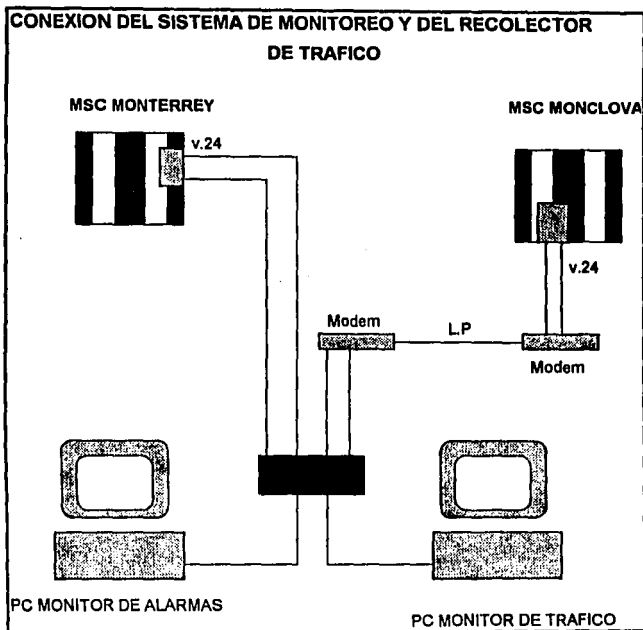
Figura II.2-1 Esquema de Conexión Típico del Monitor de Alarmas y del Recolector del Tráfico.
