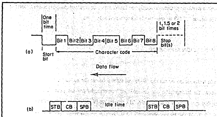
Figura 1.2.1-3 Transmisión asincrónica (a) transmisión de carácter de ocho bits. (b) transmisión de varios caracteres. stb=start bit; cb= bits de carácter; spb=stop bits; tiempo desocupado es el tiempo entre la transmisión de cada carácter.
