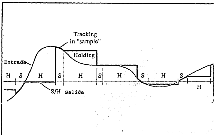
Figura 1.1.2-1. (b) Respuesta en el dominio del tiempo de un circuito S / H Ideal.
