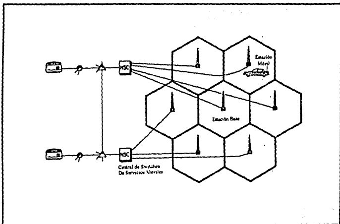
FIGURA I.3.5.1 Estructura de la Red Celular
