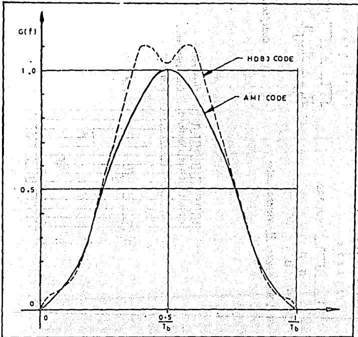
Figura I.2.5-14. Espectro de potencia S_x(f) para los códigos HDB3 y AMI.
