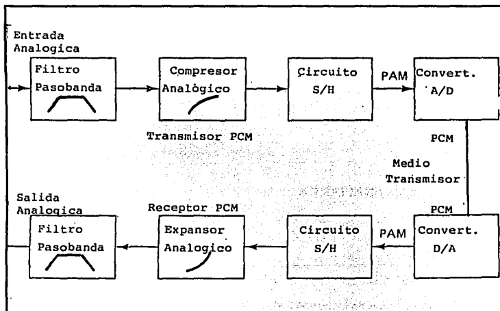
Figura 1.1.3-9. Sistema PCM de compansión analógica.
