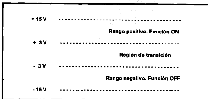
Figura I.2.6-6. Niveles de voltaje de intercambio del circuito.
