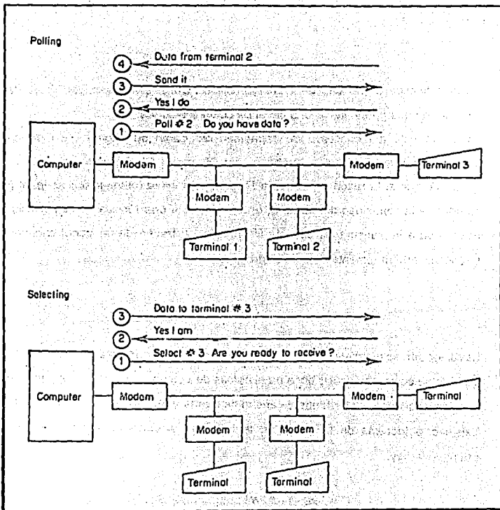
Figura 1.2.1-7 Poll y select. Poll y select es un método que permite a varios dispositivos usar una línea común de una manera ordenada.
