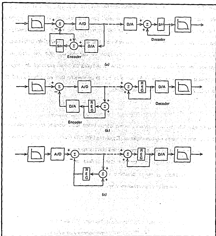
Figura 1.1.3-15. Implementaciones DPCM. (a) Integración analógica.
