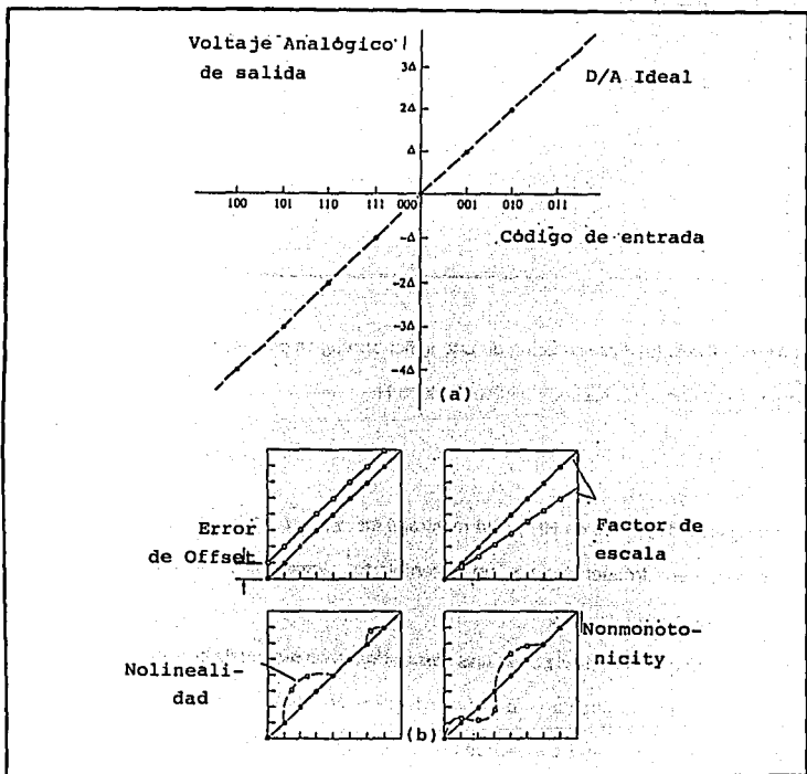
Figura 1.1.2-5. (a) Características ideales de un convertidor D / A y (b) desviaciones típicas del funcionamiento de los convertidores D / A prácticos.
