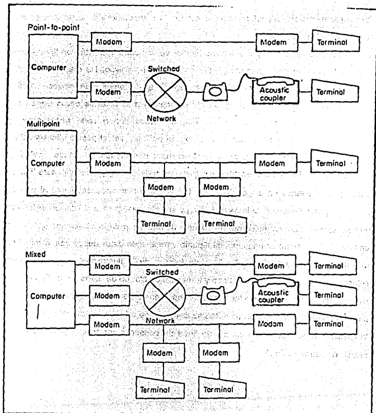
Figura 1.2.1-6 Estructura de línea en redes. Arriba: punto a punto. Centro: multipunto (mullidrop). Abajo: estructura de línea mixta
