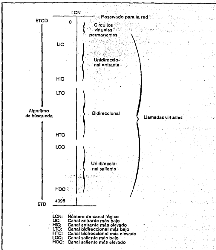
Figura 1.1.11-4. Canales lógicos X.25
