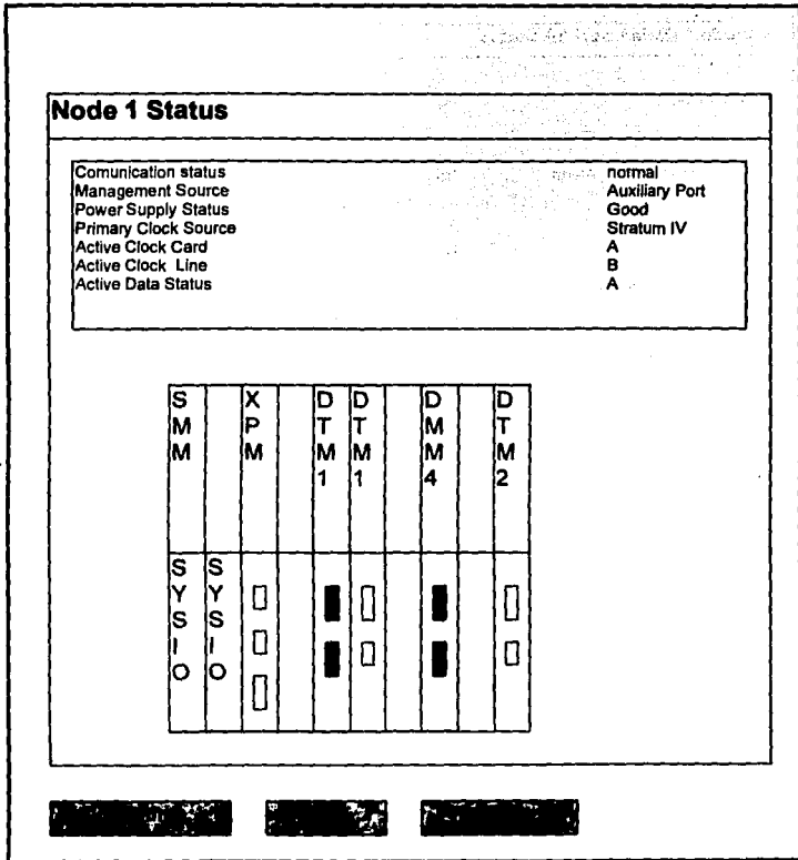
Figura III.3.6-5. Ventana de estados de nodos.
