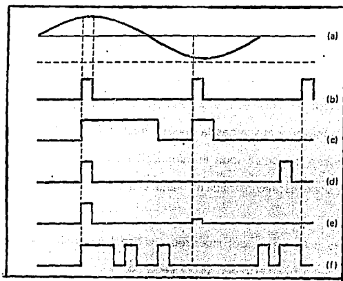
Figura 1.1.3-1. Modulación de pulsos: (a) señal analógica; (b) pulso muestreado; (c) PWM; (d) PPM; (e) PAM; (f) PCM.
