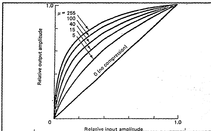
Figura I.1.3-10. Características de la ley \mu de compresión.
