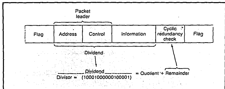
Figura I.1.11-8. Operación del código de redundancia cíclica (CRC)
