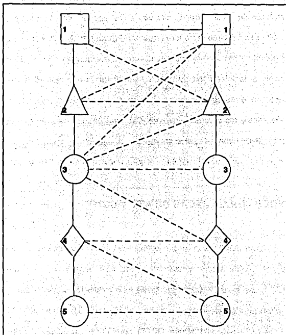
Figura I.1.13-4. La red jerárquica norteamericana (ATT). Note como los rangos más altos se conectan en malla.
