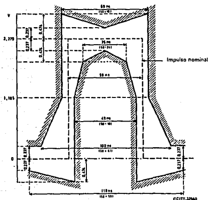
FIGURA 16/G.703 Plantilla para el impulso en el caso de un interfaz a 8448 kbit/s
