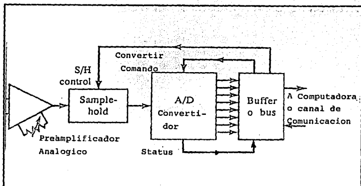
Figura 1.1.2-1. (a) Diagrama a bloques de los elementos básicos de un ADC.
