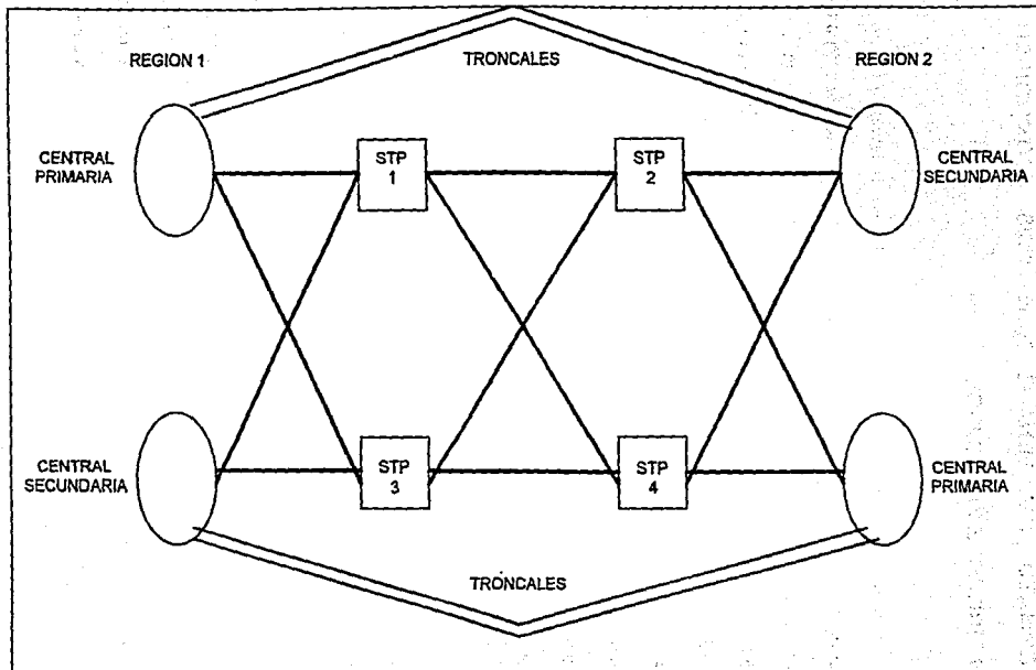
Figura I.1.6-5. Modo No asociado CCIS de acuerdo al concepto de punto de transferencia de señal STP.
