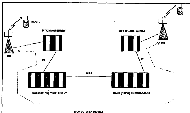
Figura II.1-4. Conexión de los MSC con los CALD
