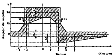
FIGURA 10/G.703
