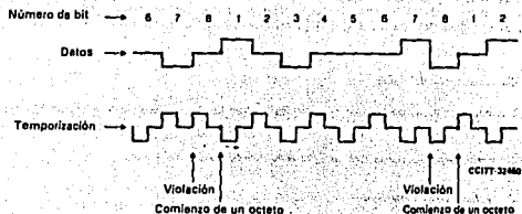
FIGURA 6/G.703
