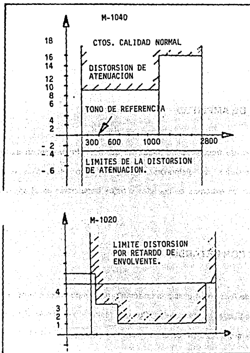
Figura I.2.4-2. Límites de distorsión por atenuación y por retardo de envoltura.
