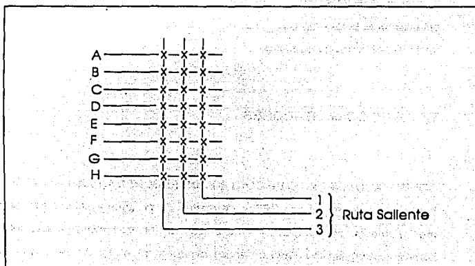
Figura 1.3.2-2. Conmutador de disponibilidad limitada
