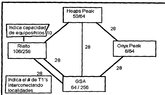
Figura I.1.8-2. Interconexión entre localidades.
