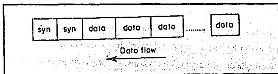
Figura 1.2.1-4 Transmisión síncrona. En la transmisión síncrona, uno o mas caracteres syn se transmiten para establecer el reloj antes de la transmisión de datos.
