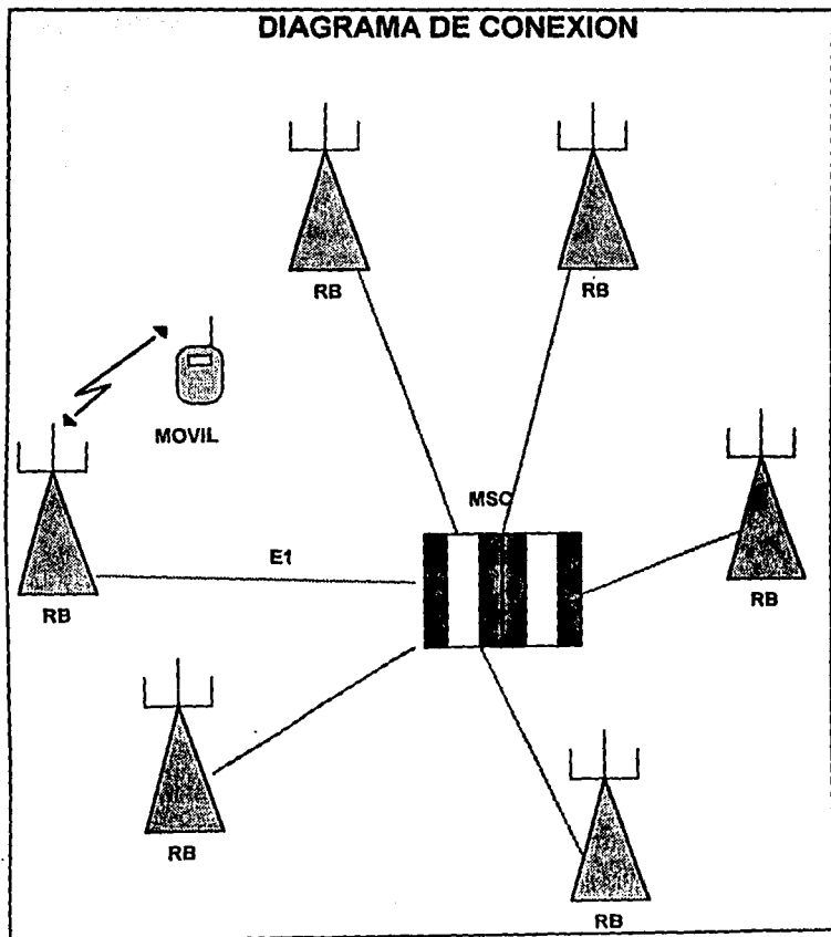
FIGURA II.1-1. Esquema básico de un sistema de telefonía celular.
