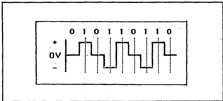
Figura 1.2.5-5. Señalización bipolar no-retorno a cero.
