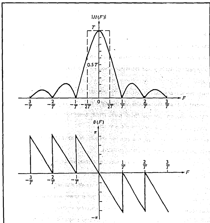
Figura 1.1.2-7. Características de respuesta en frecuencia del S/H.
