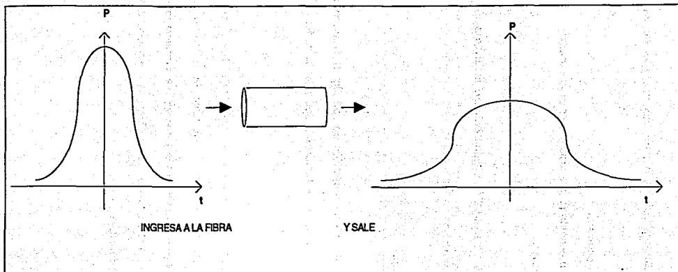
Figura 1.1.5-5. Ensanchamiento del pulso.
