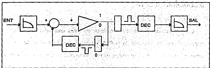
Figura I.1.4-2. Diagrama a bloques funcional de un codificador/decodificador Delta.
