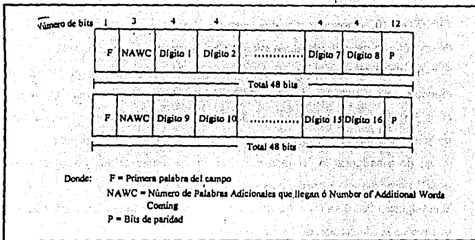
Figura 1.3.3-6 Formato del mensaje que origina el móvil
