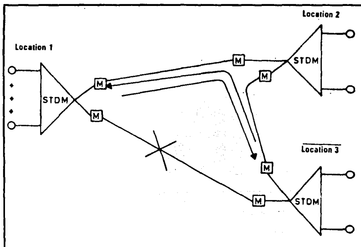
Figura I.1.9-11. Direccionamiento alterno.
