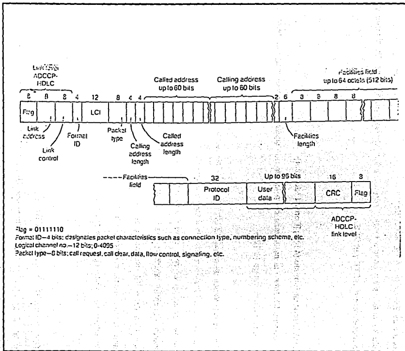
Figura 1.1.11-9. La Trama de requisición de llamada y estructura de paquete para X.25
