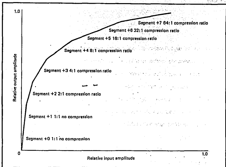
Figura I.1.3-12. Características de compresión \mu 255
