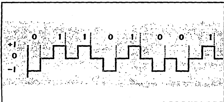
Figura I.2.5-4. Señalización polar retorno a cero.
