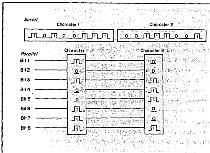
Figura 1.2.1-5 Tipos de transmisión. En la transmisión serial, los bits que componen los caracteres que se van a transmitir son enviados en secuencia a través de la línea. En la transmisión en paralelo, los caracteres son transmitidos serialmente pero los bits que representan el carácter que se va a enviar en paralelo.
