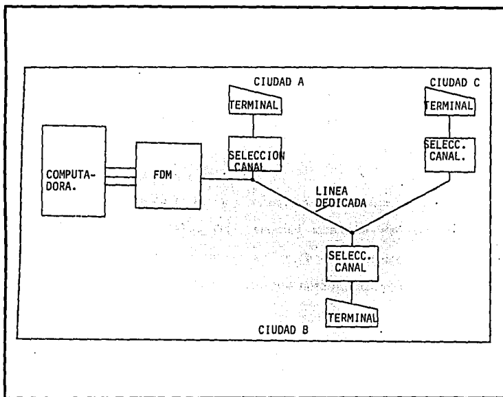
Figura 1.1.9-3. FDM permite la operación de circuitos multipunto.
