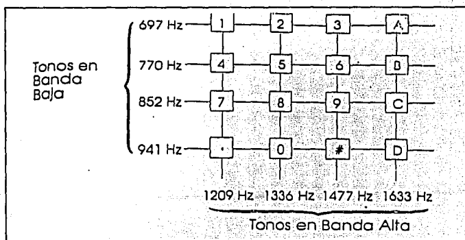
Figura 1.3.2-4 Sistema estándar por marcación por tonos.
