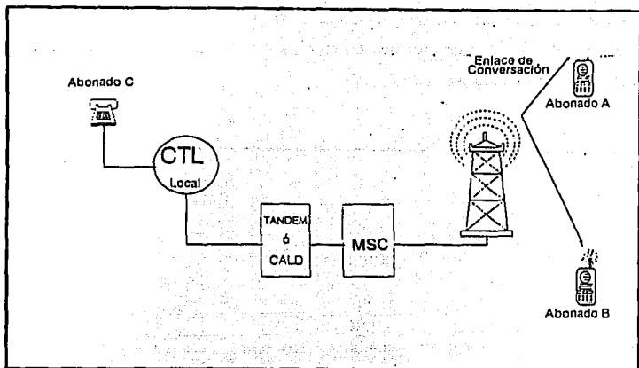
Figura I.3.1-2. Interconexión de la Central Celular con la Red Pública de Telefonía Comutada y el Sistema de Telefonía Celular
