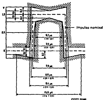
FIGURA 9/C.703
