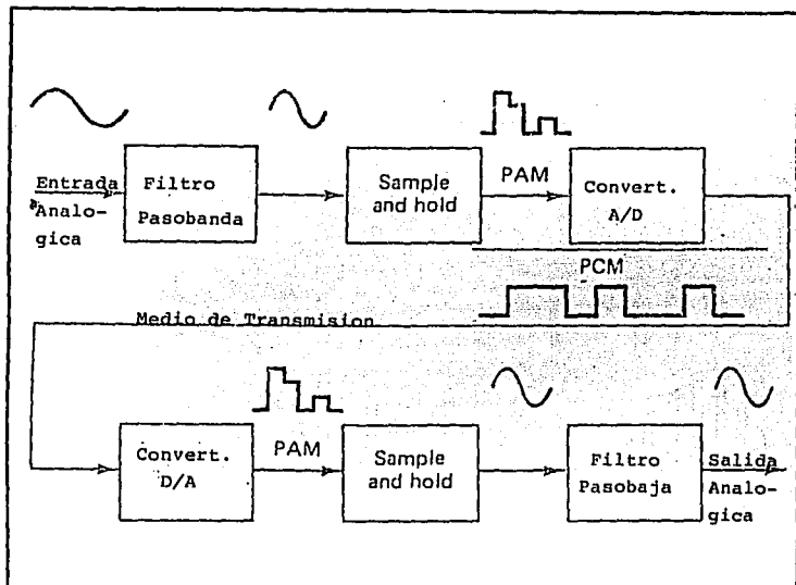
Figura 1.1.3-2. Diagrama a bloques simplificado de un sistema PCM
