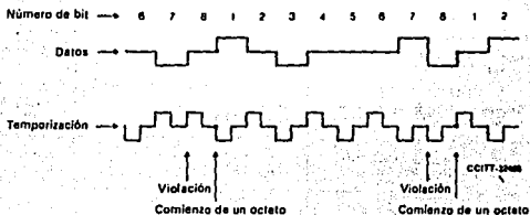
FIGURA 7/G.703
