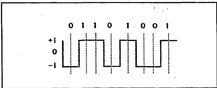
Figura 1.2.5-3. Señalización polar no-retorno a cero.
