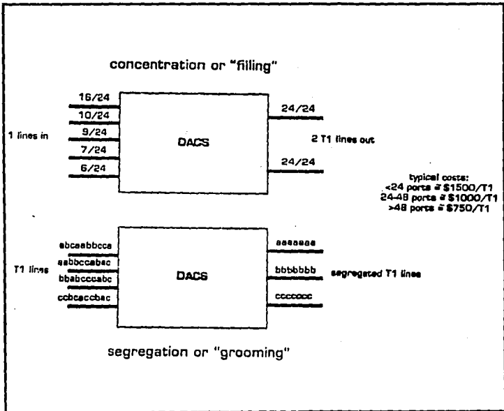
Figura I.1.8-1. Segregación o "grooming".
