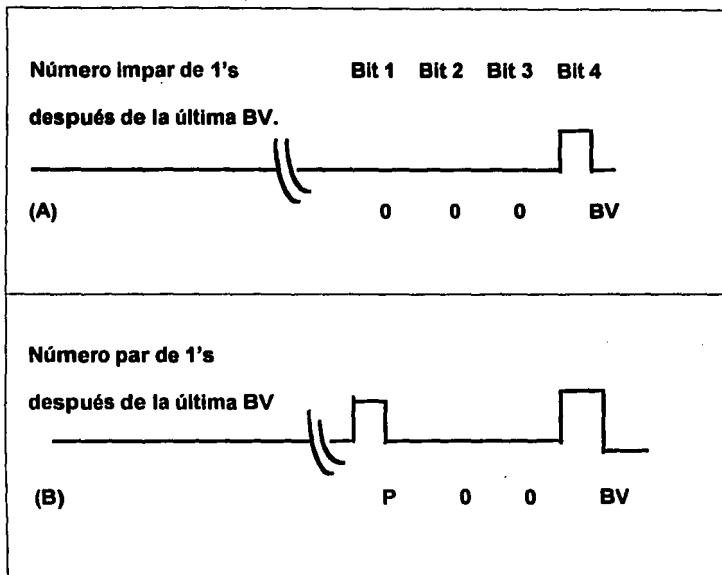
Figura 1.1.7-2. Codificación HDB3: P = polaridad, BV = violación bipolar.
