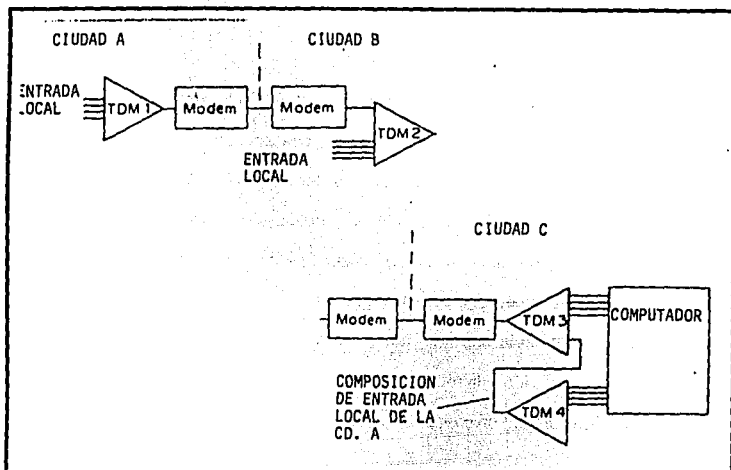
Figura 1.1.9-6. Multiplexaje Multipunto en serie.
