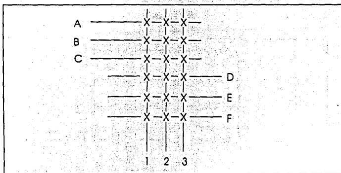
Figura 1.3.2-3 Conmutador con trayectorias internas múltiples entre entradas y salidas
