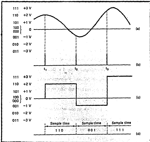
Figura I.1.3-7. (a) Señal analógica de entrada; (b) Pulso de muestreo; (c) señal PAM; (d) código PCM.
