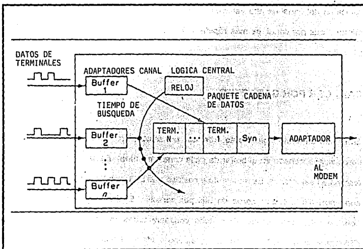
Figura 1.1.9-4. Multiplexaje por división de tiempo.
