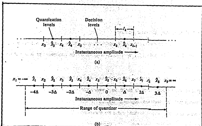
Figura 1.1.2-2. Proceso de cuantización y ejemplo de un cuantificador midrise.
