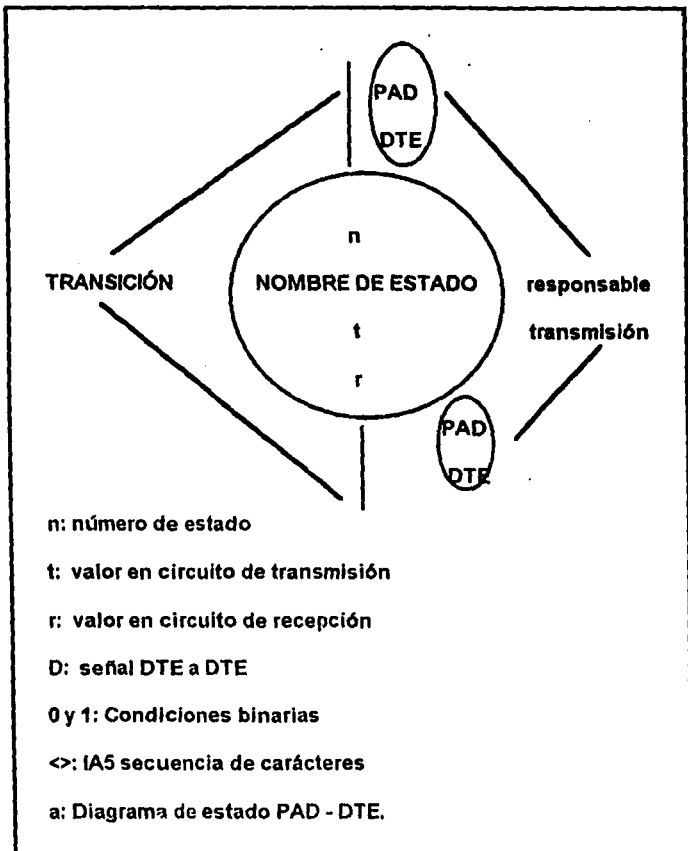
Figura I.1.10-3. Comunicación PAD/DTE.
