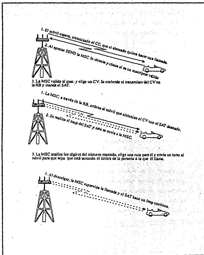
Figura 1.3.3-2. Proceso de llamada desde un móvil
