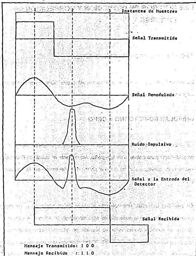
Figura I.2.4-4. Efecto del Ruido Impulsivo.
