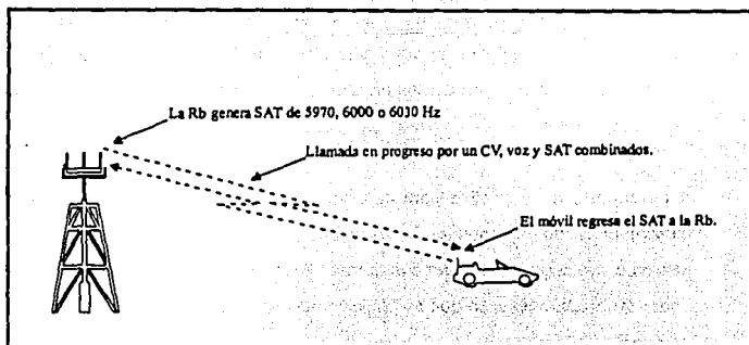
Figura 1.3.3-3 Proceso de Supervisión de llamada
