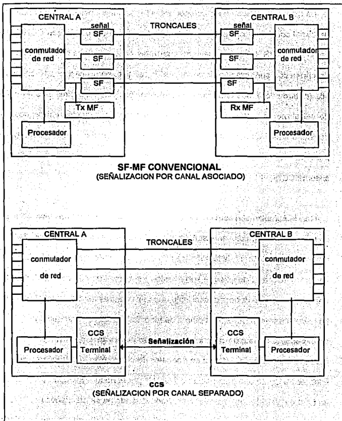
Figura I.1.6-1 Técnica de señalización analógica comparada con la técnica de señalización por canal común (CCS).
