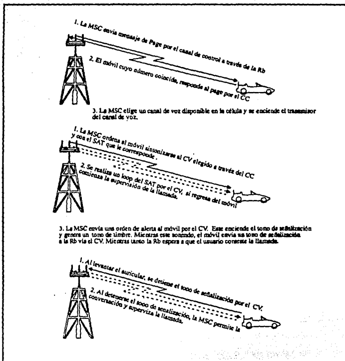
Figura I.3.3-1. Proceso de llamada a un móvil.
