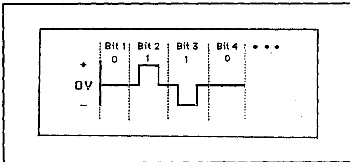
Figura 12.5-7. Señalización bipolar de 50% RTZ (AMI).
