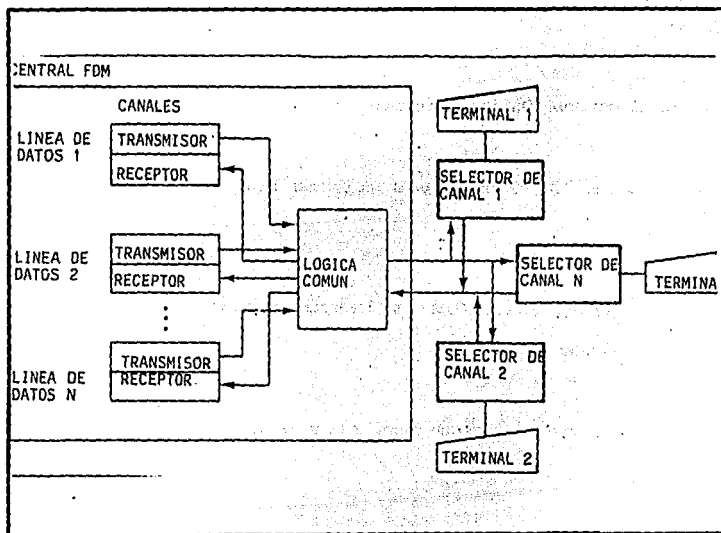
Figura I.1.9.2. Multiplexaje por División de Frecuencia.
