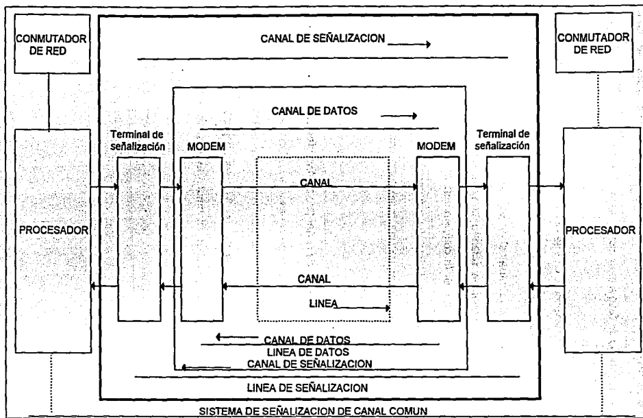
Figura 1.1.6-2 Componentes funcionales básicos del sistema de señalización de canal común.
