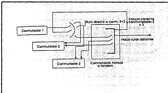
Figura 1.3.2-9. Configuración de un Conmutador de Troncal Simple
