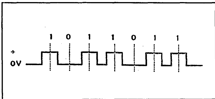
Figura 1.2.5-2. Señalización unipolar retorno a cero. La señal siempre retorna al nivel cero después de cada bit uno.
