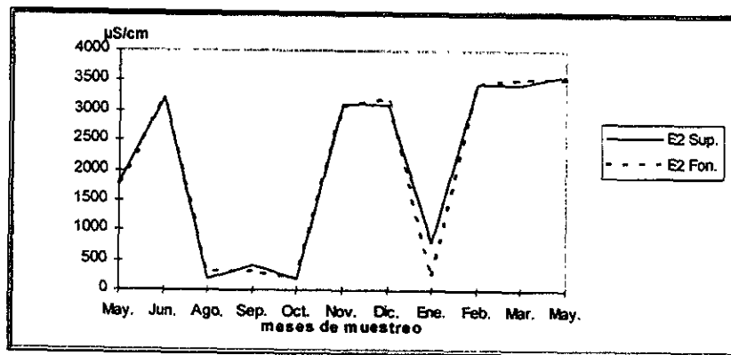
Fig. 20. Variación de la conductividad en el estanque dos.
