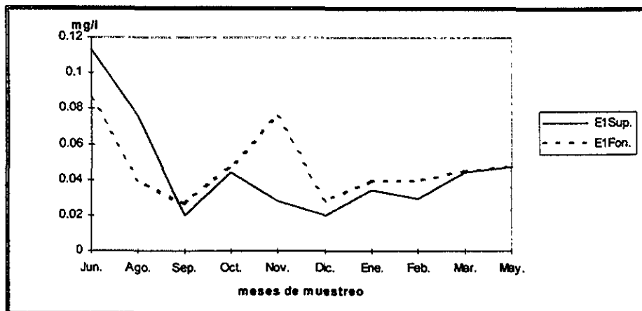
Fig. 27. Variación de ortofosfatos registrado en el estanque uno.
