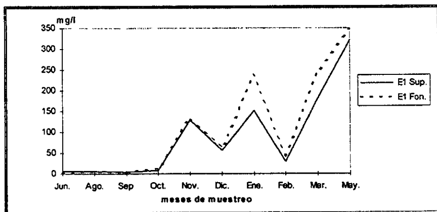
Fig. 12. Variación de la dureza de calcio registrada en el estanque uno.
