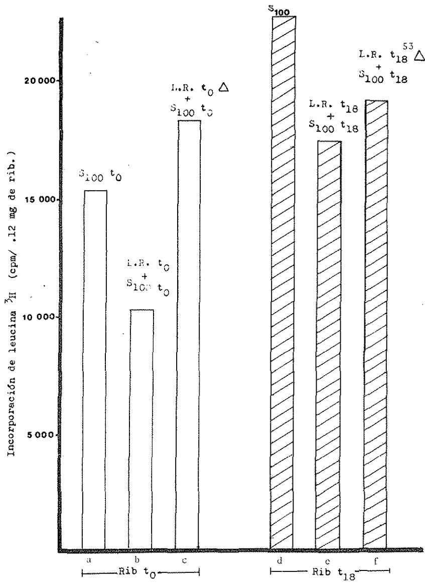
Fig. 10. Inhibición de síntesis de proteínas por la adición de lavado ribosomal. Se midió la incorporación de leucina tritiada in vitro en la fracción insoluble en ácido tricloroacético en presencia del lavado ribosomal, 10 6 u g de prot., 8500 dializado (L.R.), tanto calentado a ebullición (Δ) como sin llevar a cabo este tratamiento.
