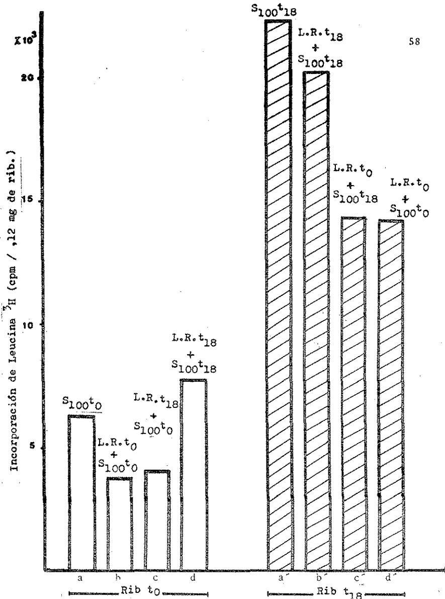
Fig. 13. Inhibición de la síntesis de proteínas por la adición de lavados ribosomales. 100 ug de ribosomas aislados de tejido fresco o envejecido fueron incubados con una mezcla de reacción para síntesis de proteínas en presencia del sobrenadante celular y en algunos casos con 100 ug del lavado ribosomal K 500 (L.R.) dializado.
