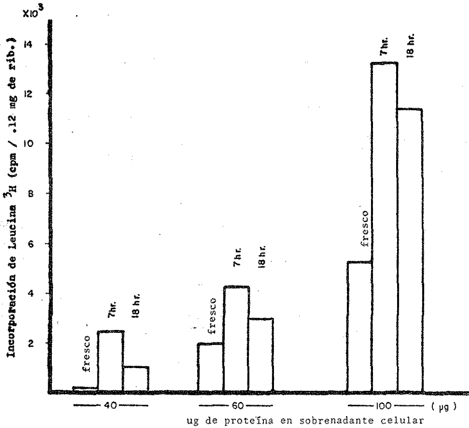
Fig. 8. Incorporación in vitro de leucina ^3\text{H} por ribosomas de tejido fresco de papa en presencia de sobrenadante celular obtenido de tejido fresco, de 7.0 h y de 18.0 h de incubación.
