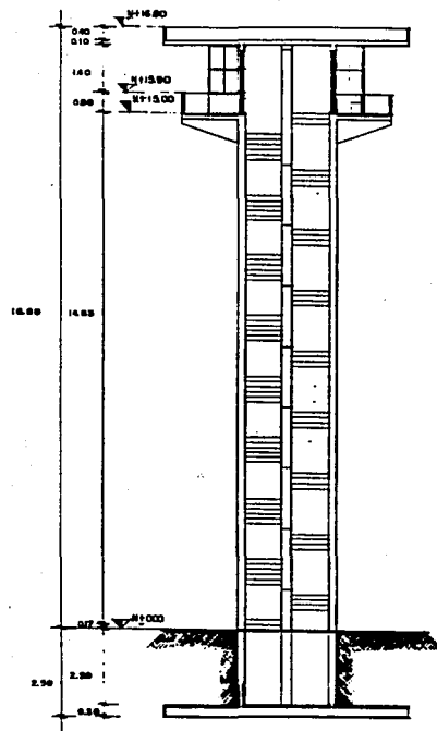
CORTE A-A' ESC. 1:75
