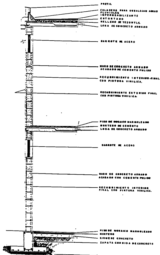
CORTE Y-Y POR FACHADA DE LAS CELDAS
