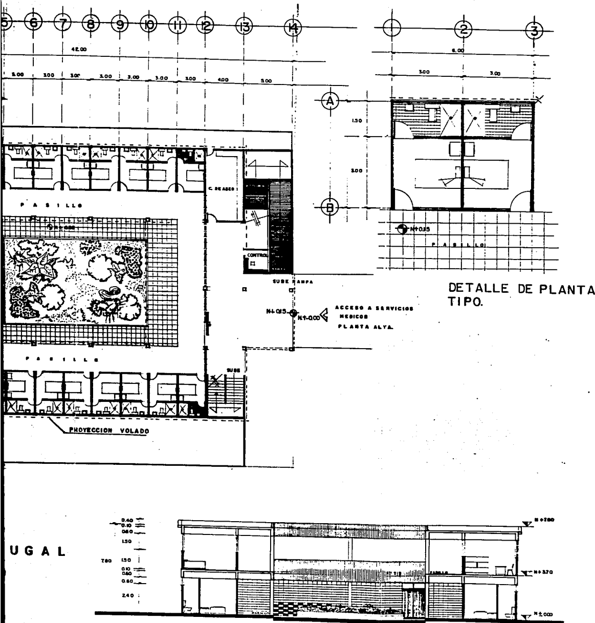
CORTE A-A'
