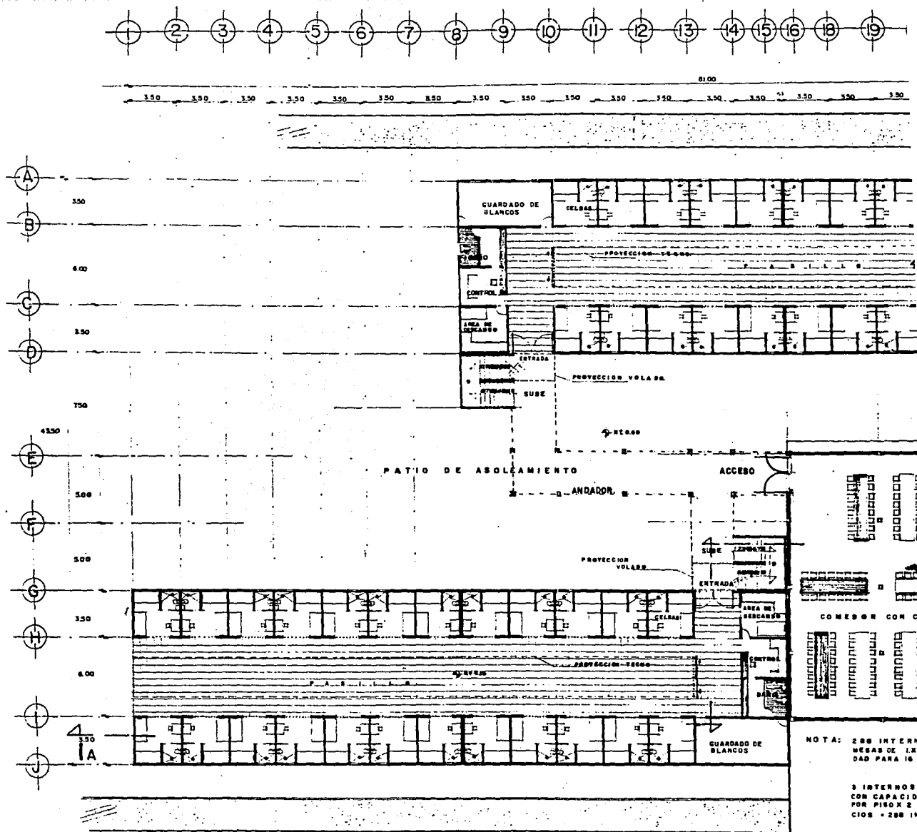
PLANTA DORMITORIOS
