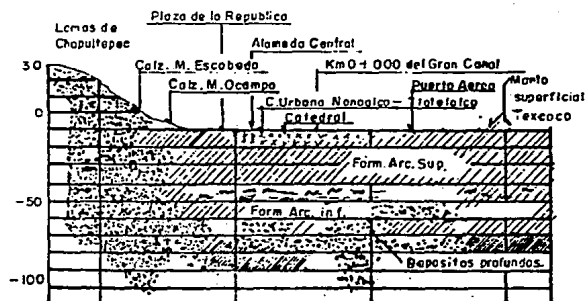
CORTE W-E (Por el Monumento a Colón)
