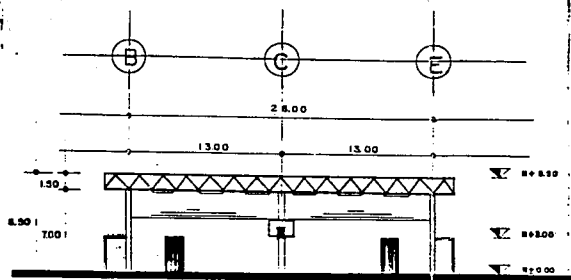
CORTE A-A ESC. 1:200
