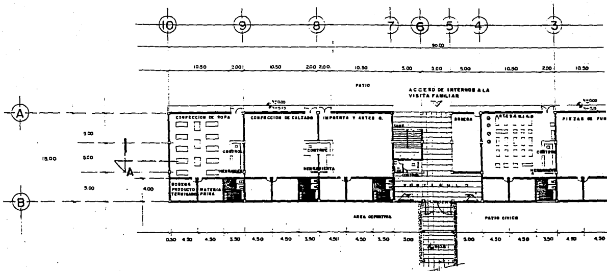
TALLERES F ESC: 1:200
