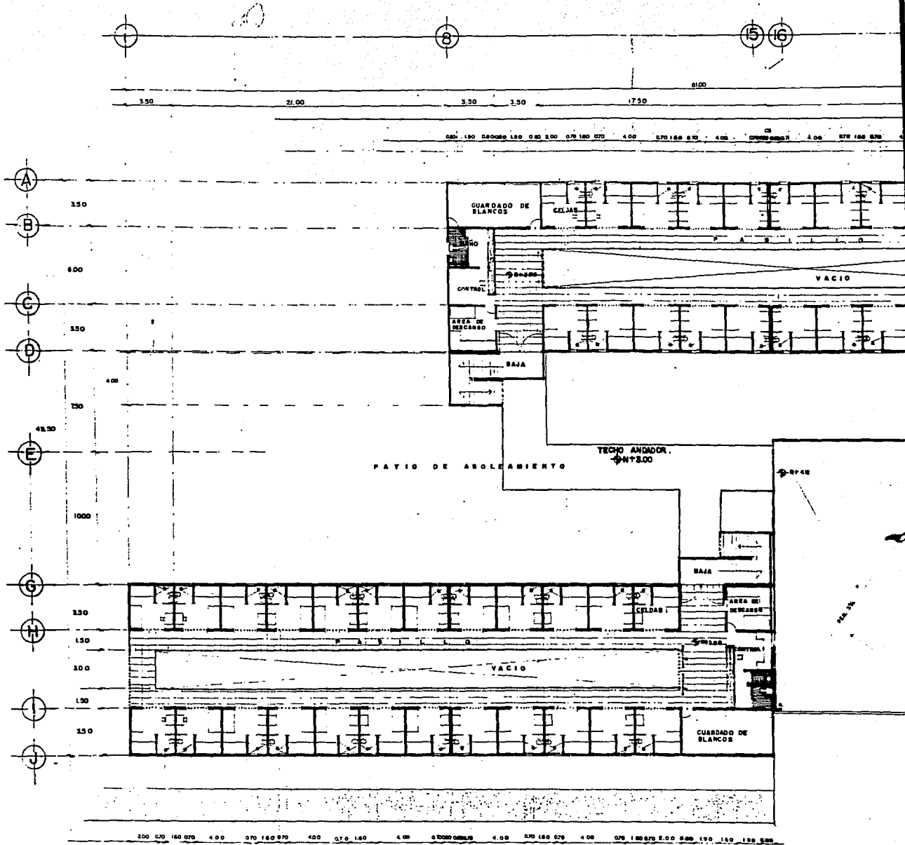
PLANTA ALTA DORMITORIOS
