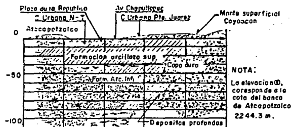
CORTE N-S (Por el Monumento a Colón)
