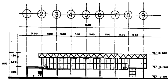
CORTE A-A ESC. 1:200
