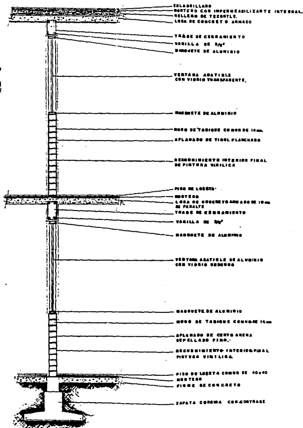
CORTE X-X POR FACHADA DE VISITA CONYUGAL
