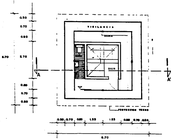
PLANTA ESC. 1:50
