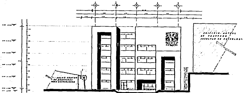
FACHADA PRINCIPAL NORTE (LA UNIVERSIDAD)
