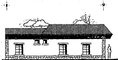
fachada noroeste.
