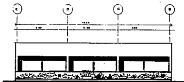
FACHADA ESTE.
