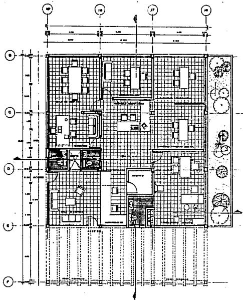
PLANTA ARQUITECTONICA.
