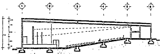
CORTE Y-Y'
