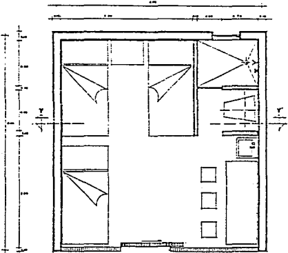
DORMITORIO TIPO
