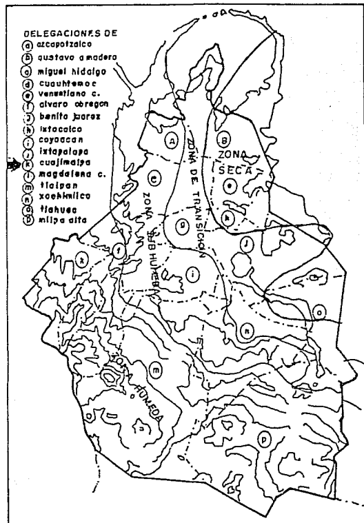
ZONIFICACION CLIMATICA DEL DISTRITO FEDERAL
