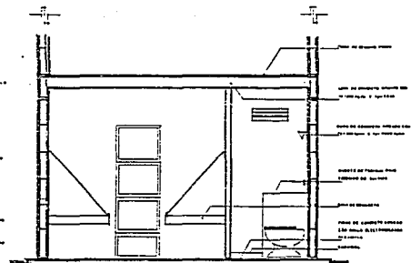
CORTE Y-Y'
