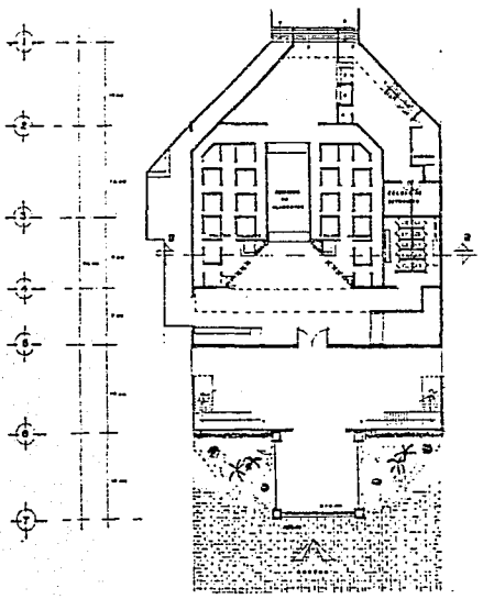
PLANTA ADUANA
