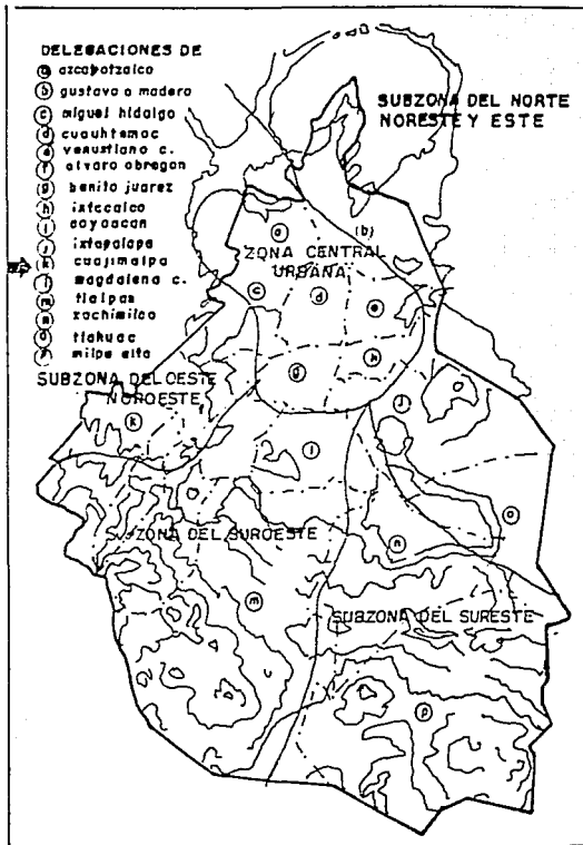
ZONIFICACION MESOCLIMATICA DEL DISTRITO FEDERAL
