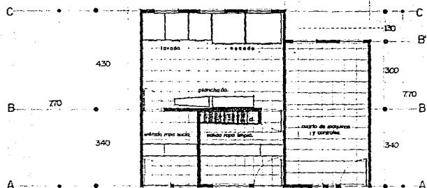
planta arquitectónica lavandería y cto. de máquinas.
