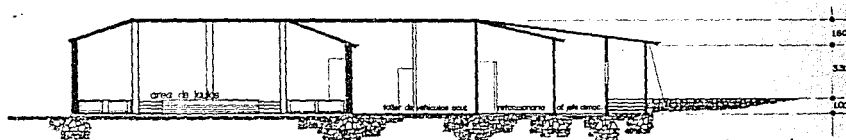
corte a-a transversal.
