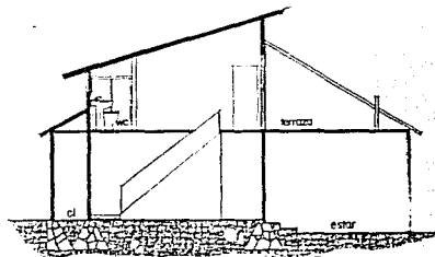
corte a-a
