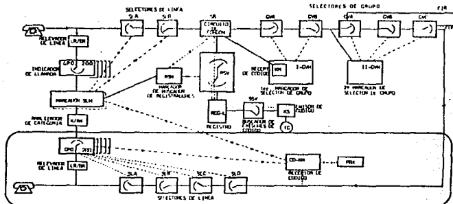
FIGURA 6 MECANISMOS TERMINALES DE LA TRANSPORTACION DE LA LLAMADA
