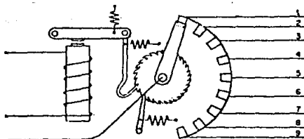
FIGURA 2 SELECTOR PASO POR PASO CON AVANCE INDIRECTO
