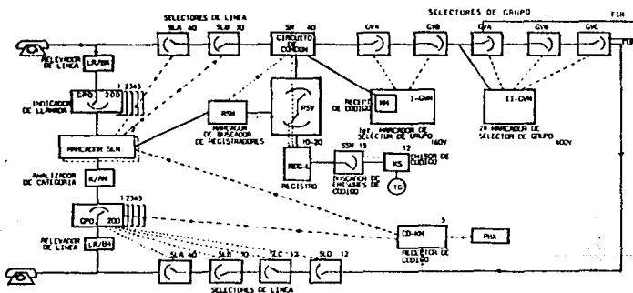
FIGURA 7 CUANTIFICACION DEL SISTEMA ELECTROMECANICO DE CONMUTACION TIPO ARF-102
