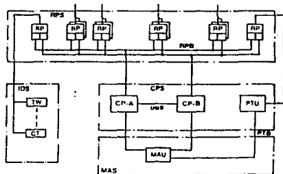
FIGURA 10 MECANISMOS BASICOS DE CONTROL DEL AUTOMATA TIPO AXE-1 (Hardware) (Diagrama a bloques)
