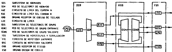
FIGURA 9 SISTEMA AUTOMATICO DIGITAL EN UNA CENTRAL TIPO AXE-1 (Diagrama a bloques del hardware)
