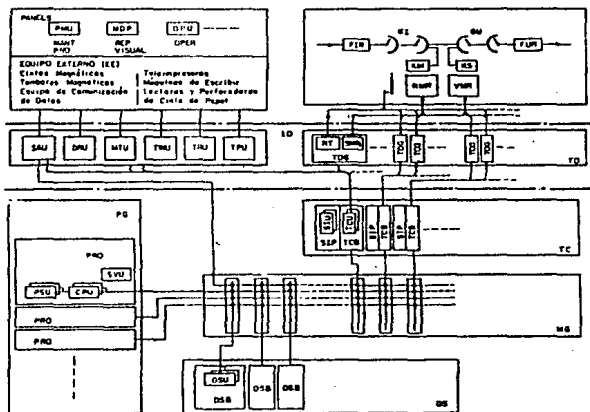
FIGURA 8 SISTEMA AUTOMÁTICO DE MAQUINARIA PARA LARGA DISTANCIA TIPO AKE-13
