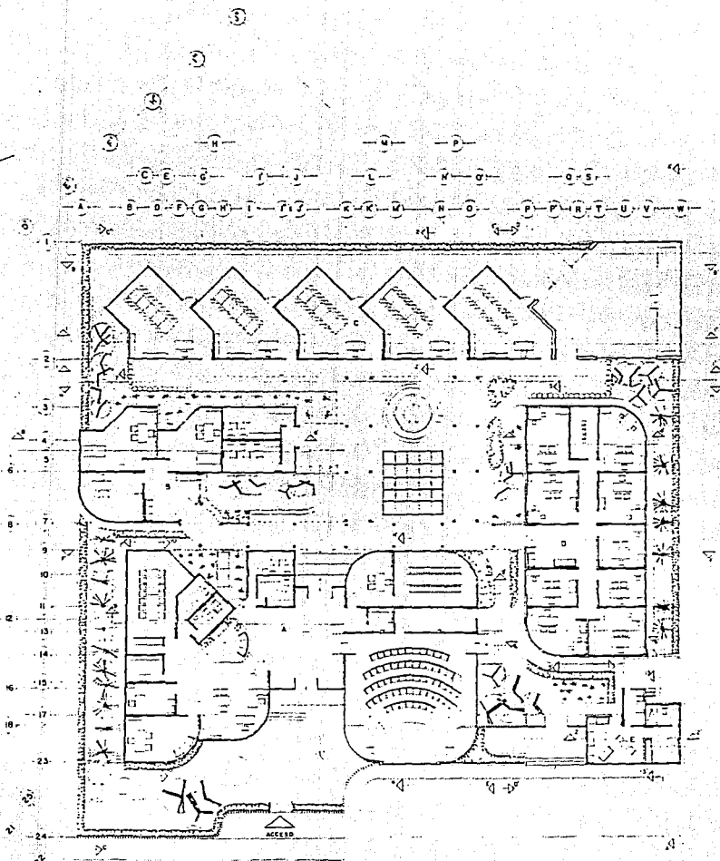
PLANTA ARQUITECTONICA
