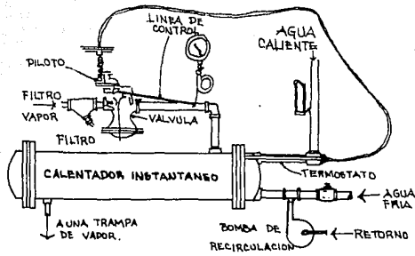
CONTROL DE AGUA CALIENTE PARA CALENTADOR INSTANTANEO
