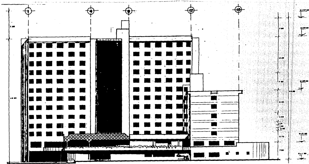
FACHADA SUR E S C . 1 1 0 0
