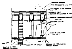
DETALLE ANGLAR FALSO PLAFON 1 1 2
