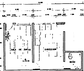
PLANTA DIRECCION MEDICA E.S.C. 1 1 9 0 0
