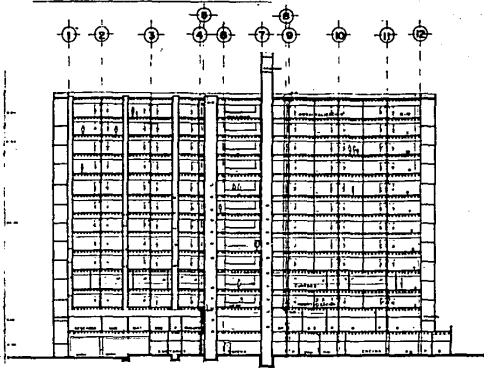
CORTE X - X' LONGITUDINAL E.S.C. 1 : 2 0 0
