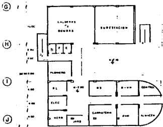
PLANTA SOTANO E.S.C. 1 2 0 0 0
