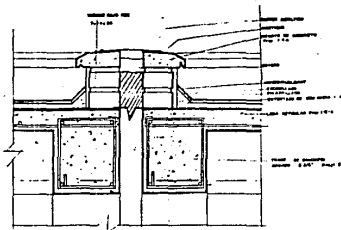
DETALLE JUNTA AZOTEA 1 1 8
