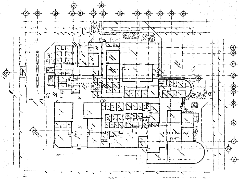
PLANTA ARQUITECTONICA BAJA
