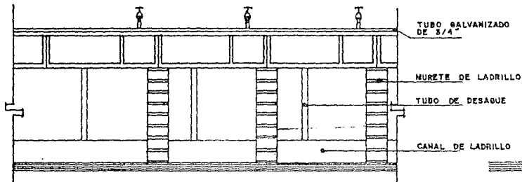
ALZADO
