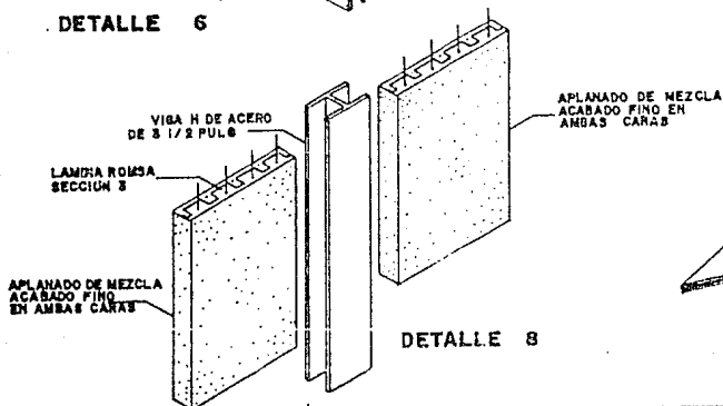
DETALLE 6
