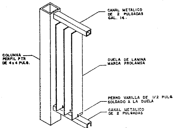
DETALLE 6
