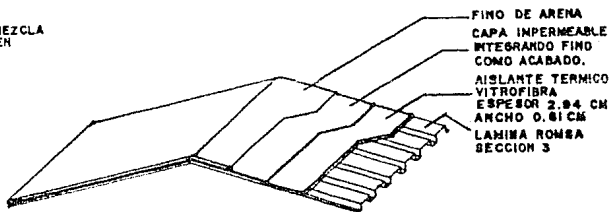
DETALLE 9
