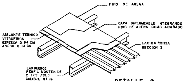
DETALLE 2
