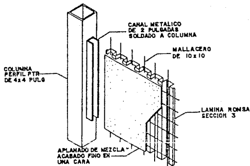
DETALLE 7
