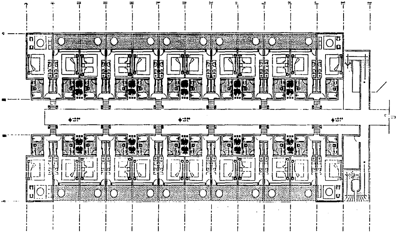
PLANTA ALTA ESCUELA N.º 1
