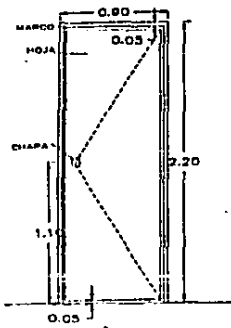
PUERTA TIPO MEDIDAS 0.75 UNA A. R. O. CURVED
