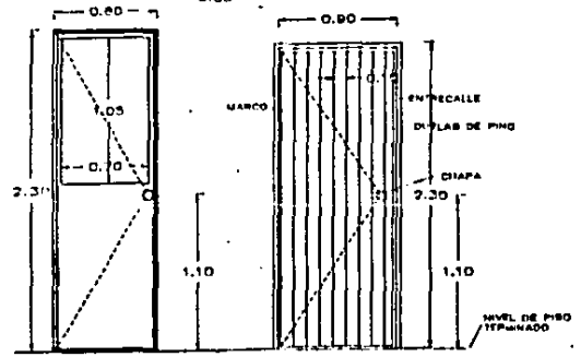
PUERTA DE ACCESO
