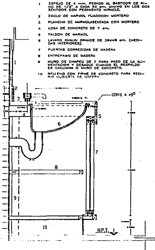
UNIDAD DEL LAVADO ( SECCION TRANSVERSAL )
