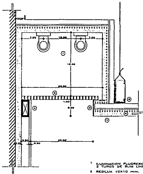
CAJILLO LUMINOSO SOBRE PLAFON ( SECCION TRANSVERSAL )
