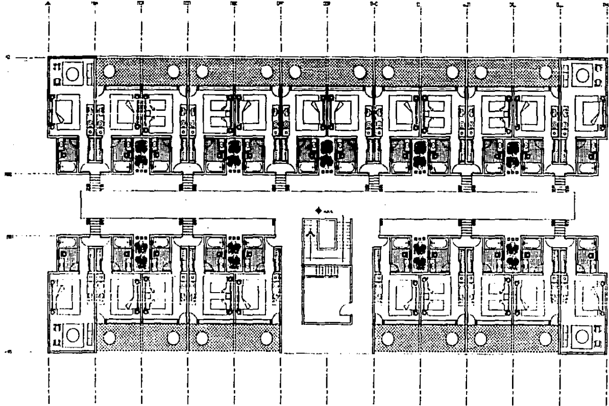
PLANTA ALTA RECONSTRUCCION D
