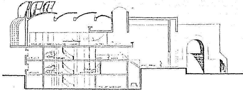
CORTE J-J'
