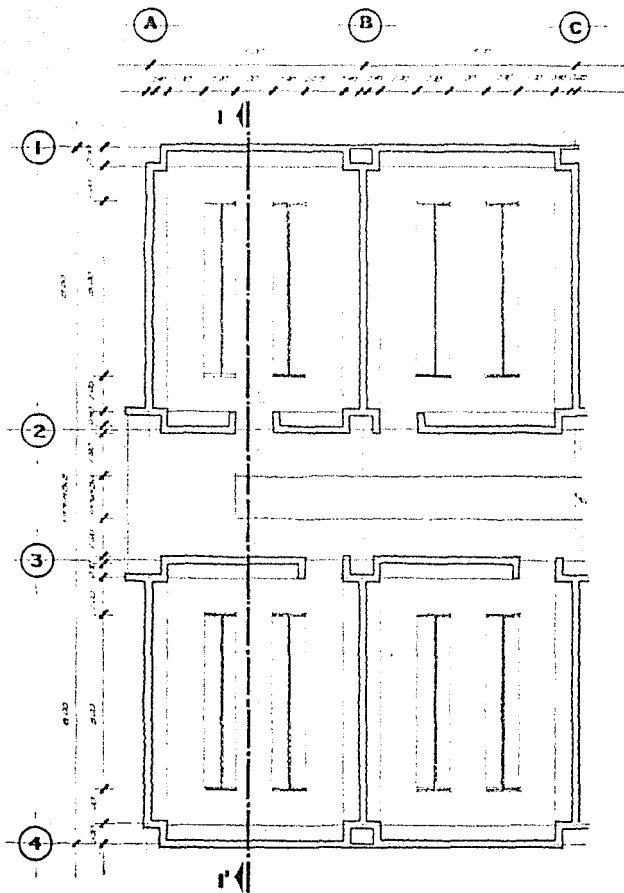
MODULO DE ACERVO DISTRIBUCION DE LA ESTANTERIA
