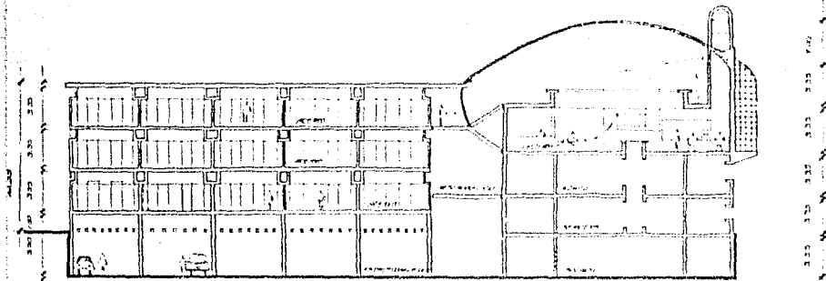
CORTE L-L'
