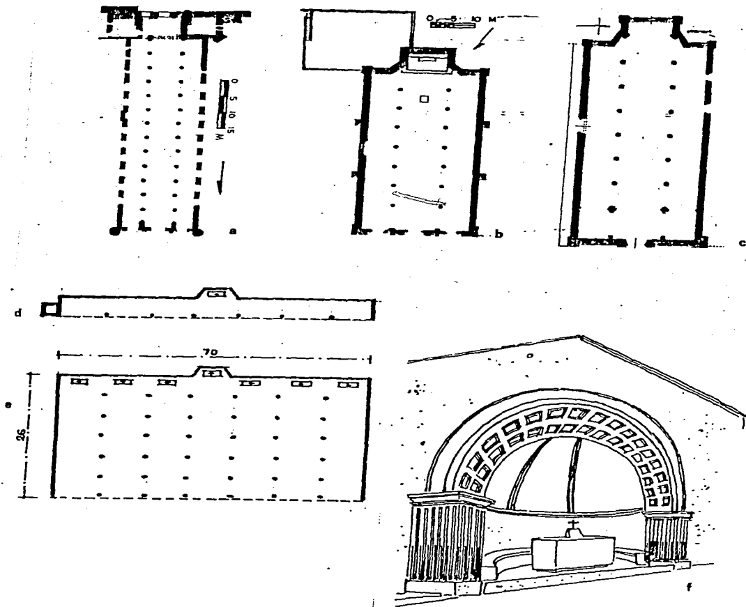
Fig. 19. Templos de plantas basilicales de tres naves muy largas y la techumbre de madera (a, b y c). Capillas abiertas (d, e, f). a) Cuicilapan, 1555; b) Tecali, 1570; c) Zacatlán, 1550-1560; d) Iglesia de San José de Los Naturales, seg. Mc Andrew, en 1539; e) La misma iglesia en 1563; f) Capilla abierta de Tarrimbaro.
