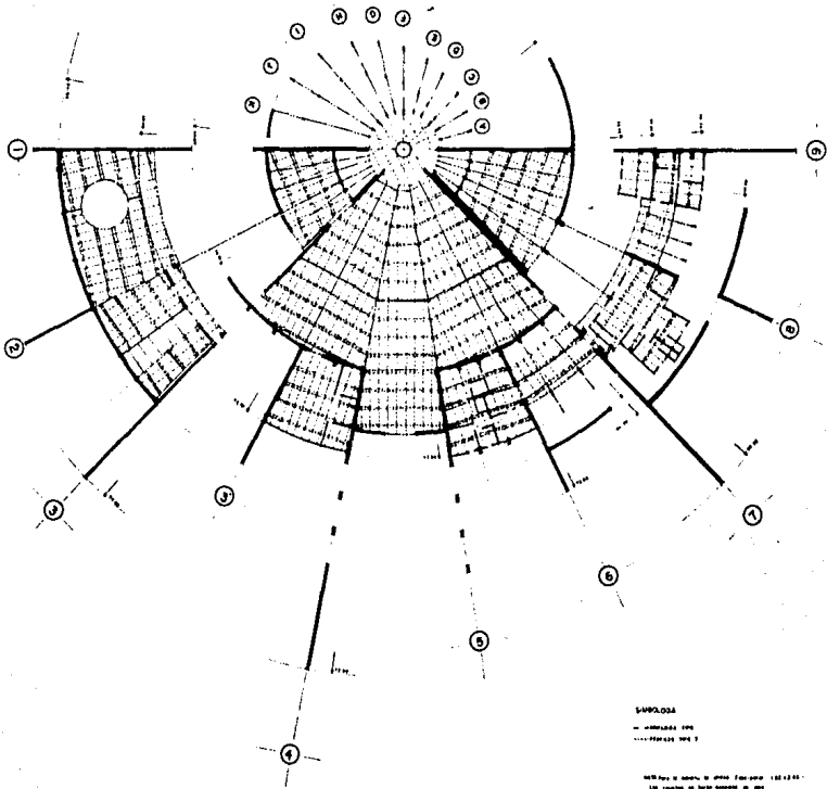
PLANTA ESTRUCTURAL ESC 1:200
