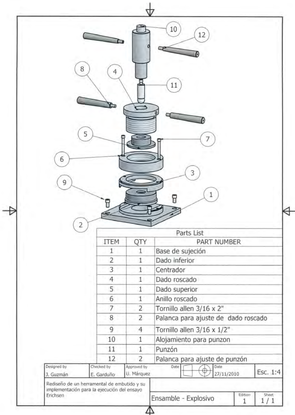
Fig. 3.22. Plano, explosivo.
