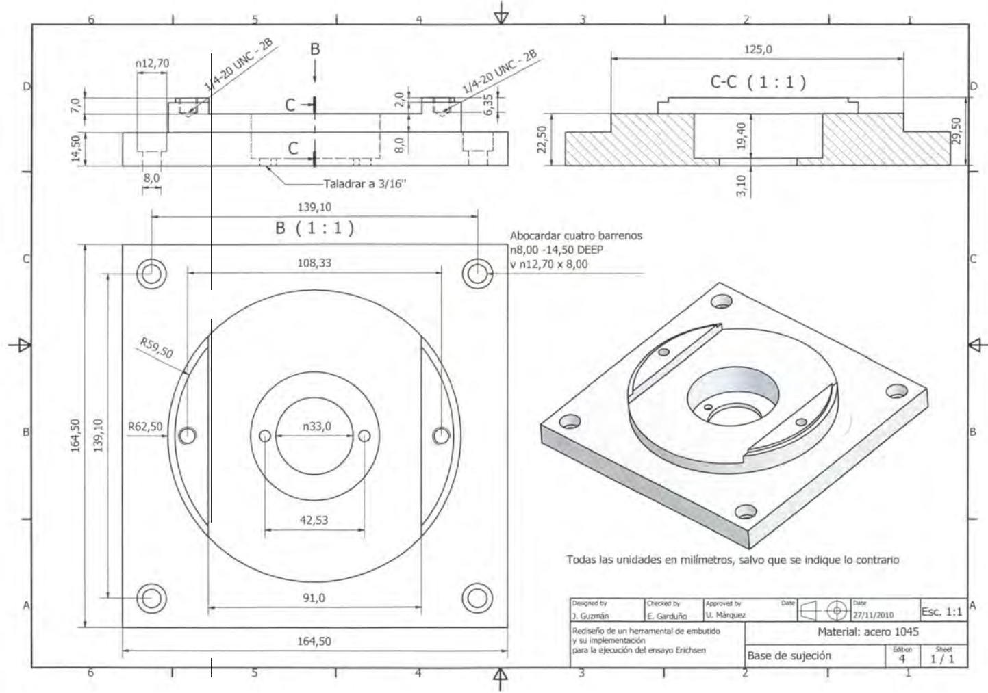
Fig. 3.12. Plano. base de sujeción.
