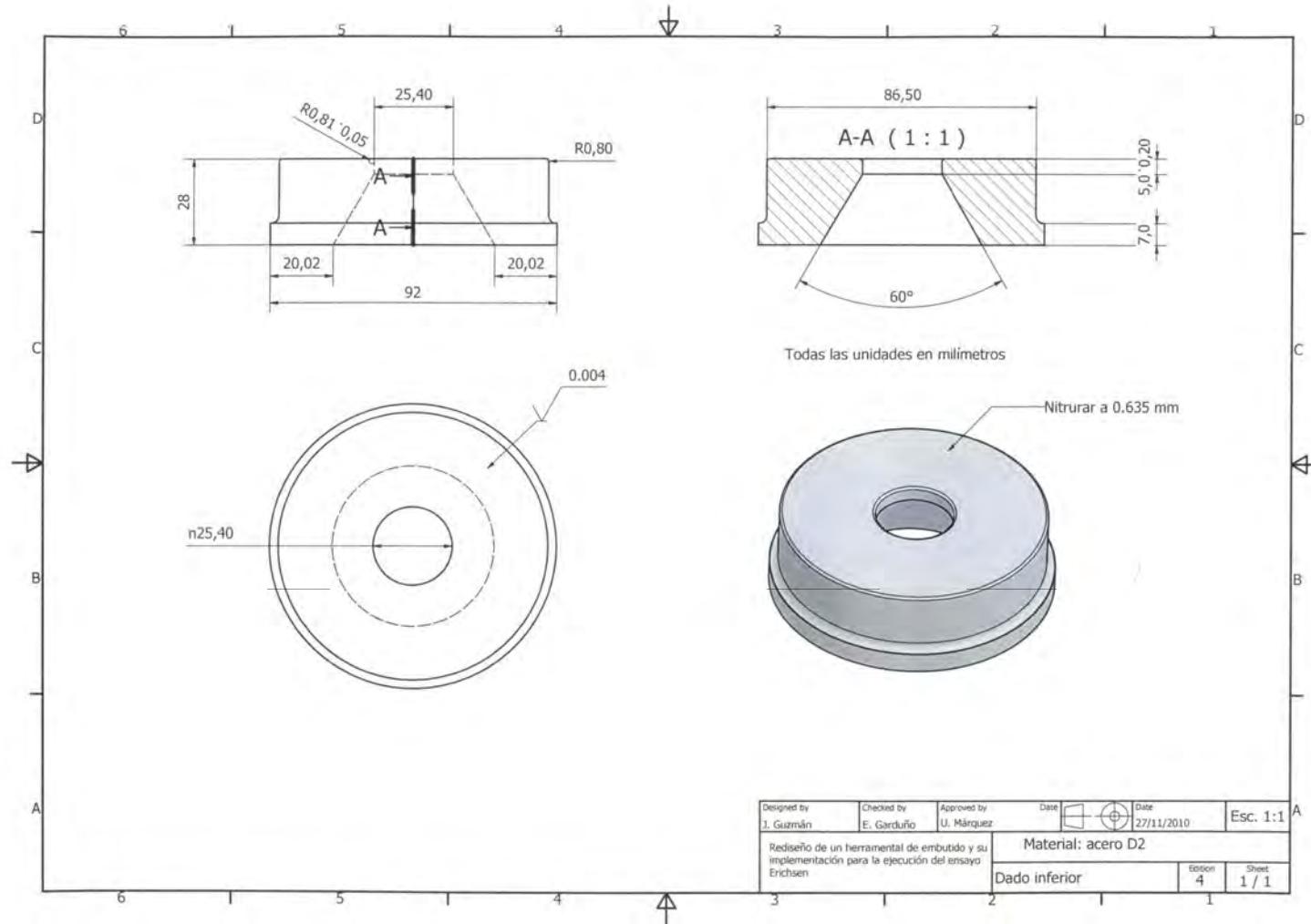
Fig. 3.13. Plano, dado inferior.
