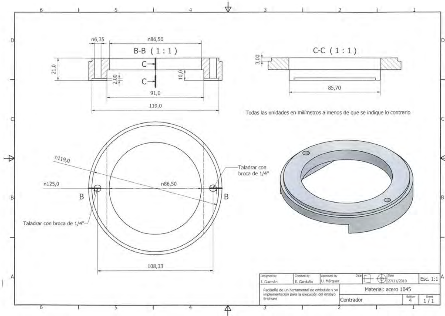
Fig. 3.14. Plano, centrador.
