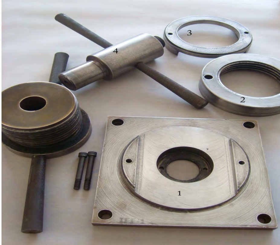
Fig. 3.11. Partes remanufacturadas del herramental: 1) Base de sujeción, 2) Anillo roscado, 3) Centrador y 4) Alojamiento para punzón
