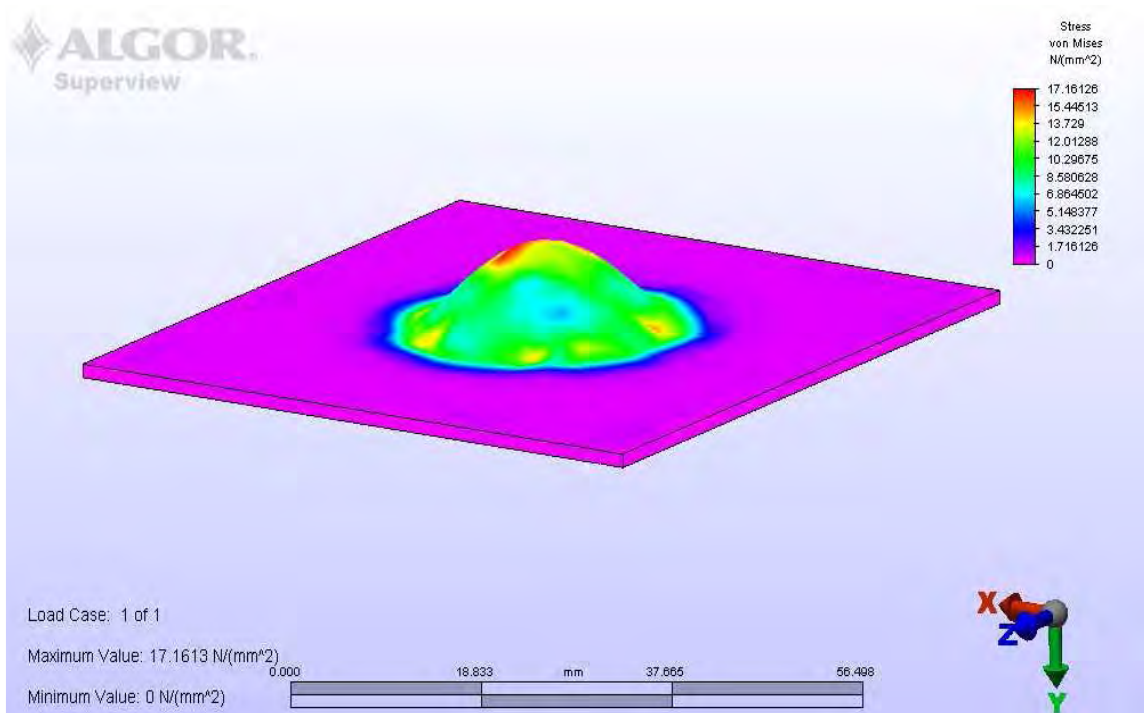
Fig. 4.8. Mapa de colores de los esfuerzos resultantes en la lámina de acero calibre 18.
