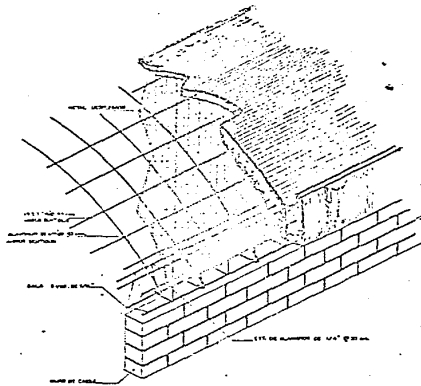
ISOMETRICO BOVEDA
