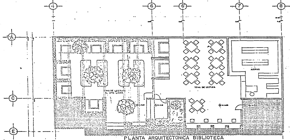
PLANTA ARQUITECTONICA BIBLIOTECA
