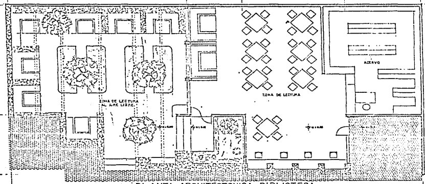
PLANTA ARQUITECTONICA BIBLIOTECA
