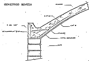
CORTE BOVEDA
