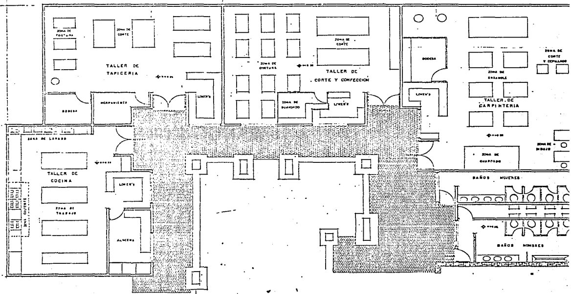
PLANTA ARQUITECTONICA TALLERES
