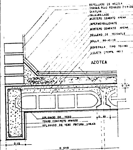
DETALLE - 1
