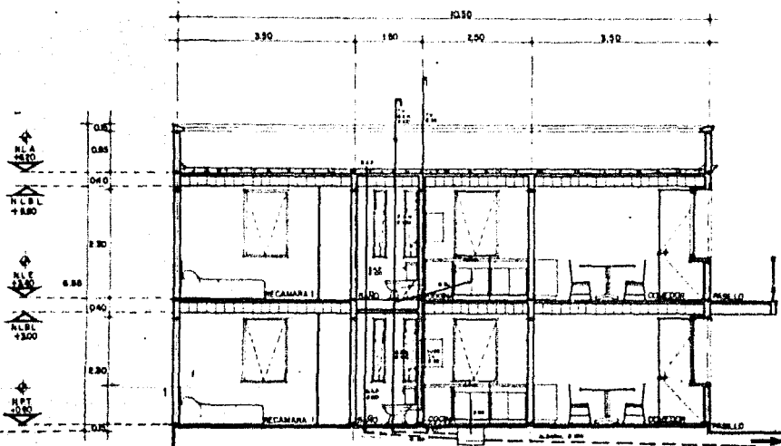
CORTE Y-Y' escala 1:50
