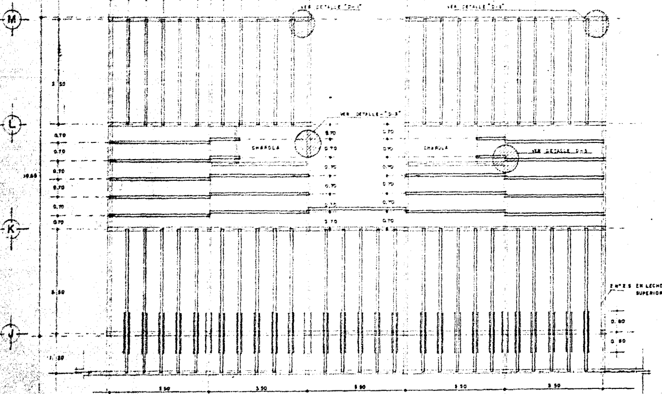
LOSA DE ENTREPISO.
