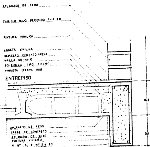
DETALLE - 2
