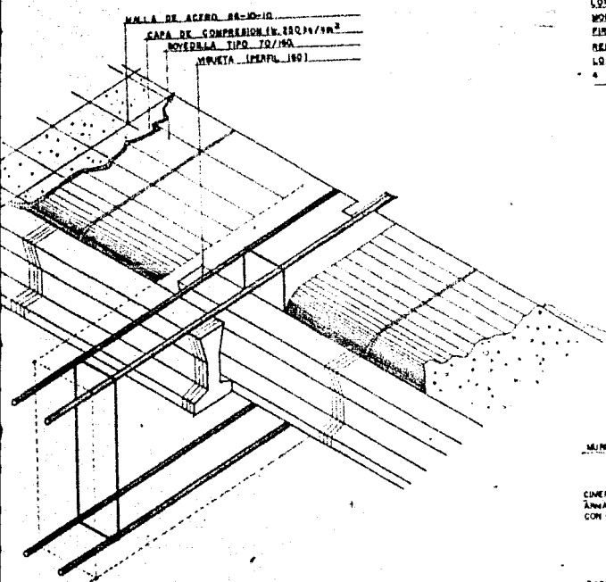
DETALLE - 1
