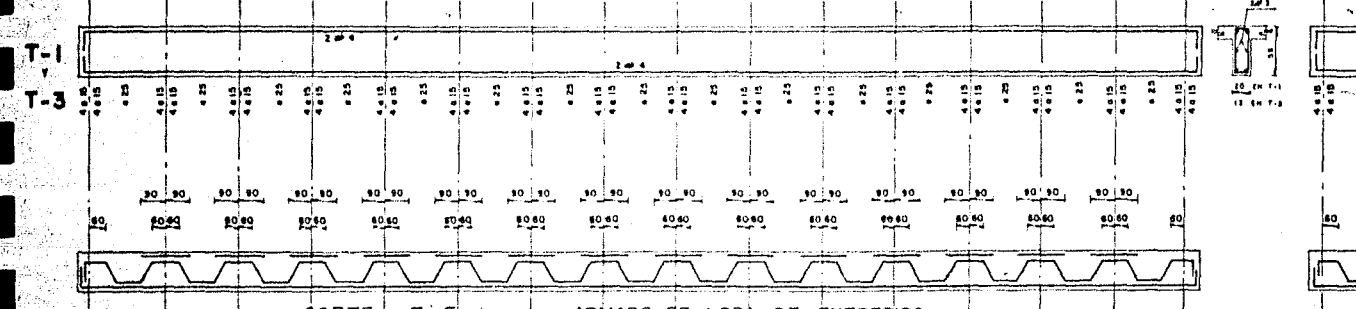
CORTE E-E ARMADO DE LOSA DE ENTREPISO
