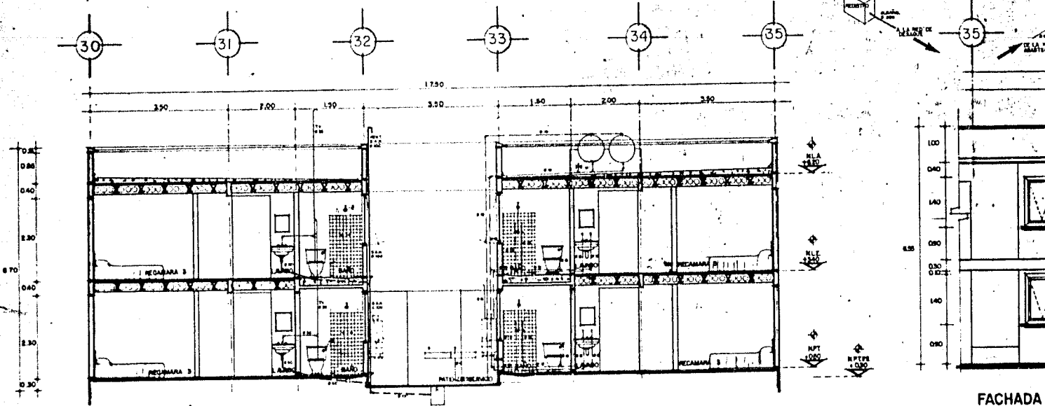
CORTA X-X' escala 1:50
