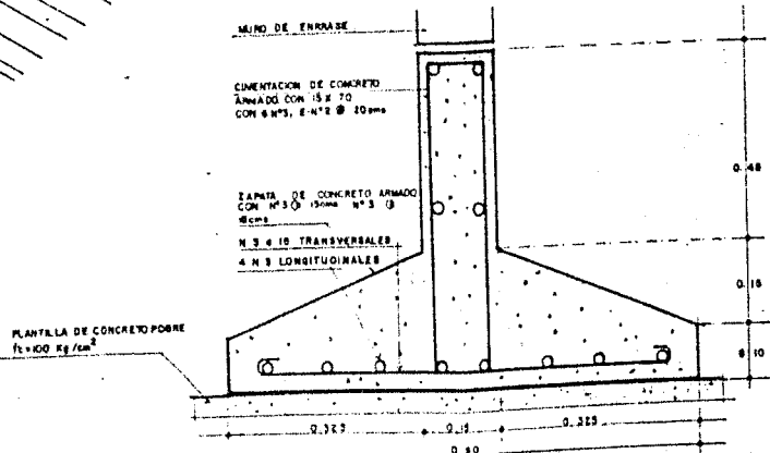
DETALLE - 4
