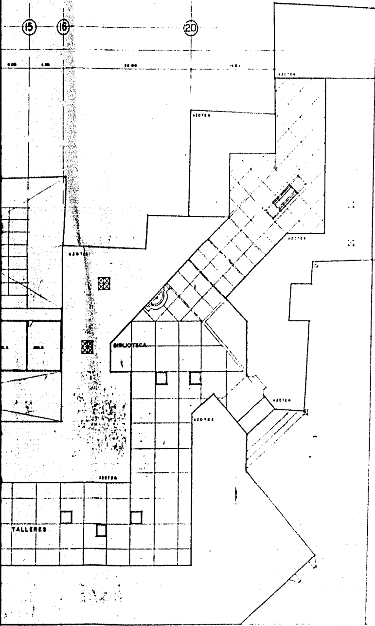
PLANTA ALTA
