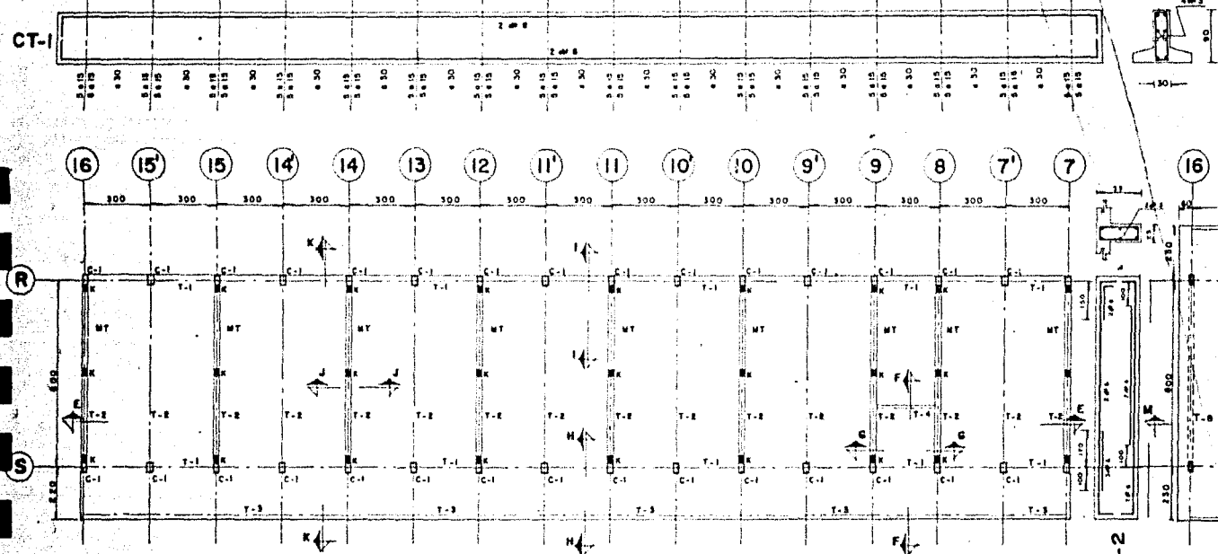
PLANTA DE ENTREPISO
