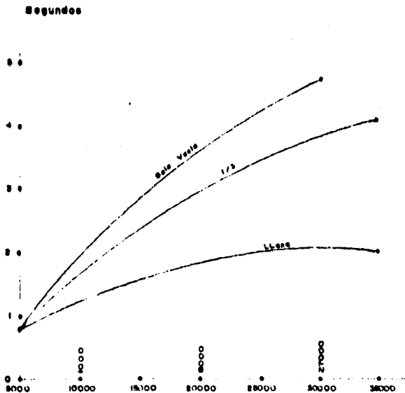
DURACION PROPORCIONADA DE LA RESONANCIA EN LOCALES PARA MUSICA Y CONVERSACION.
