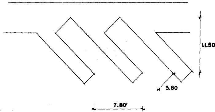
MEDIDAS MINIMAS PARA EL APARCAMIENTO DE AUTOBUSES A 45°
