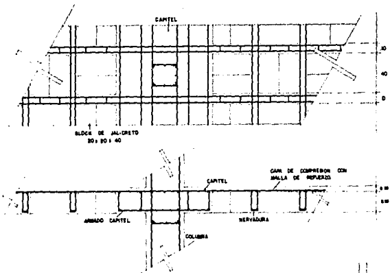
LOSA DE CONCRETO aligerada con block hueco de jal-creto
