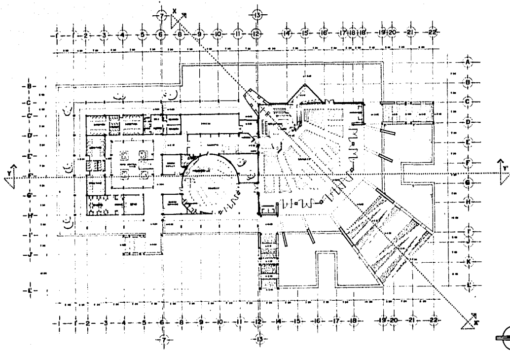
PLANTA ARQUITECTONICA NIVEL 2
