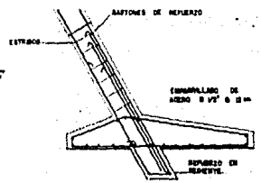
ZAPATA HORIZONTAL con carga inclinada
