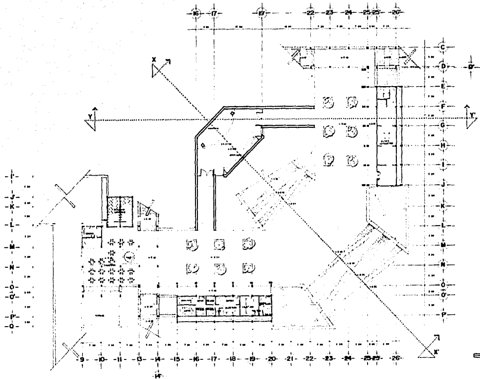
PLANTA ARQUITECTONICA NIVEL 3
