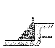
MURO DE CONTENCION (de piedra de la region)
