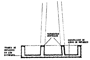
LOSA DE GIMENTACION
