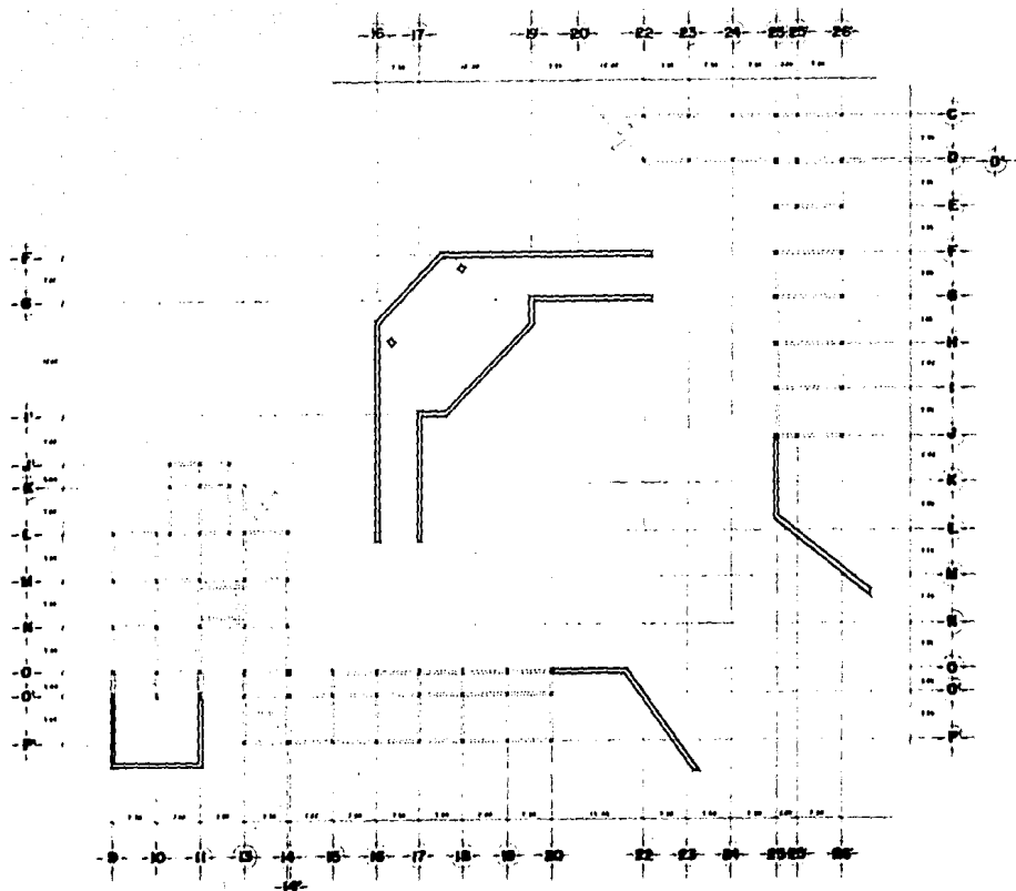
PLANTA ESTRUCTURAL NIVEL 3
