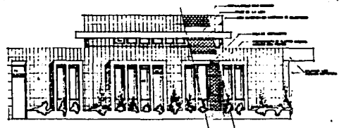
ALZADO SUR Esc. 1:50
