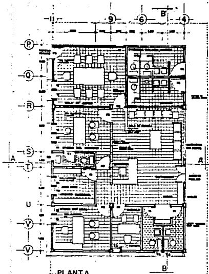
PLANTA ZONA ADMINISTRATIVA PARROQUIAL Esc. 1:500
