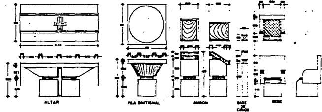
DISEÑO DE MUEBLES Esc. 1:20
