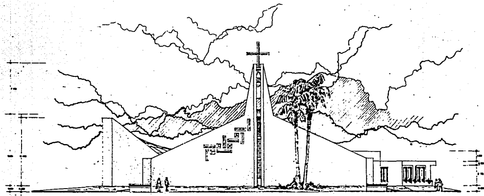
PLANO DE ALZADOS ESC: 1:100
