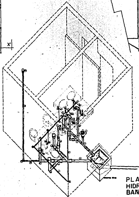
ISOMETRICO
