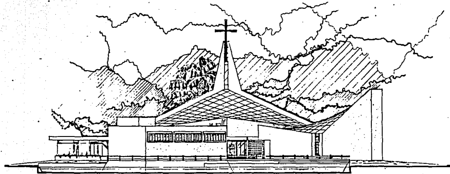
ALZADO NORESTE
