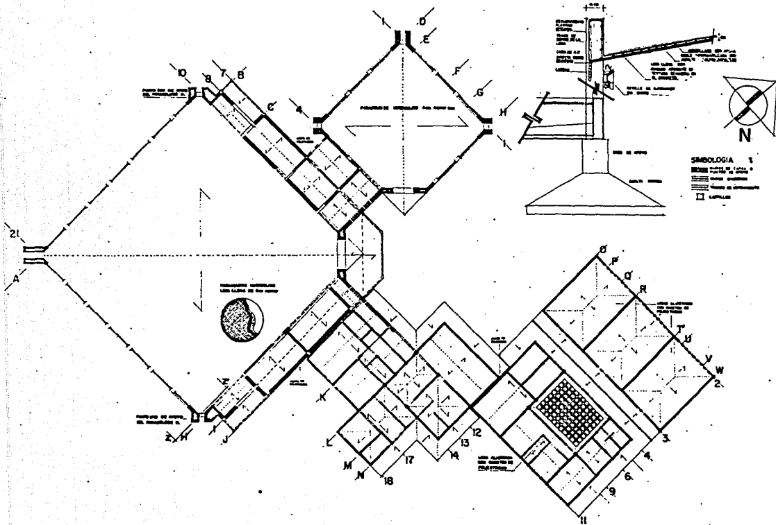
PLANO DE ESTRUCTURA Esc. 1:100
