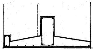
DETALLE LOSA DE CIMENTACION
