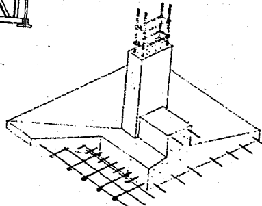
ARCLAJE DE COLUMNA EN LOSA DE CIMENTACION
