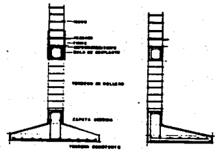
DETALLE ZAPATA CORRIDA
