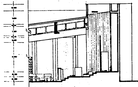
CORTE B-B'
