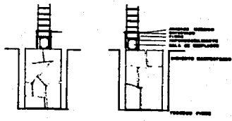
DETALLE CIMENTO MAMPOSTADO
