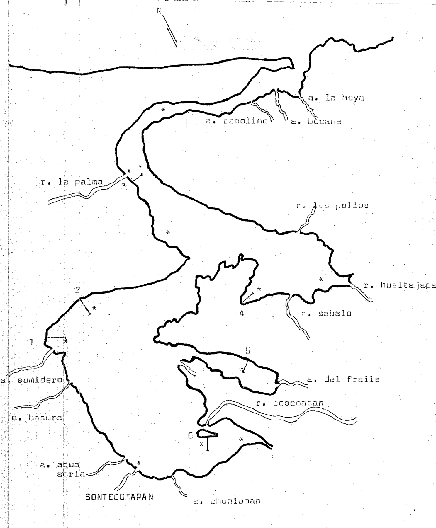
Fig. 1. Mapa general de la Laguna de Sontecomapan (modificado de Vázquez-Yanes et al, 1972). Las estaciones permanentes de muestreo y observación de los "manchones" de Ruppia maritima están marcadas con números. El agua se colectó en las zonas señaladas con asteriscos (*)
