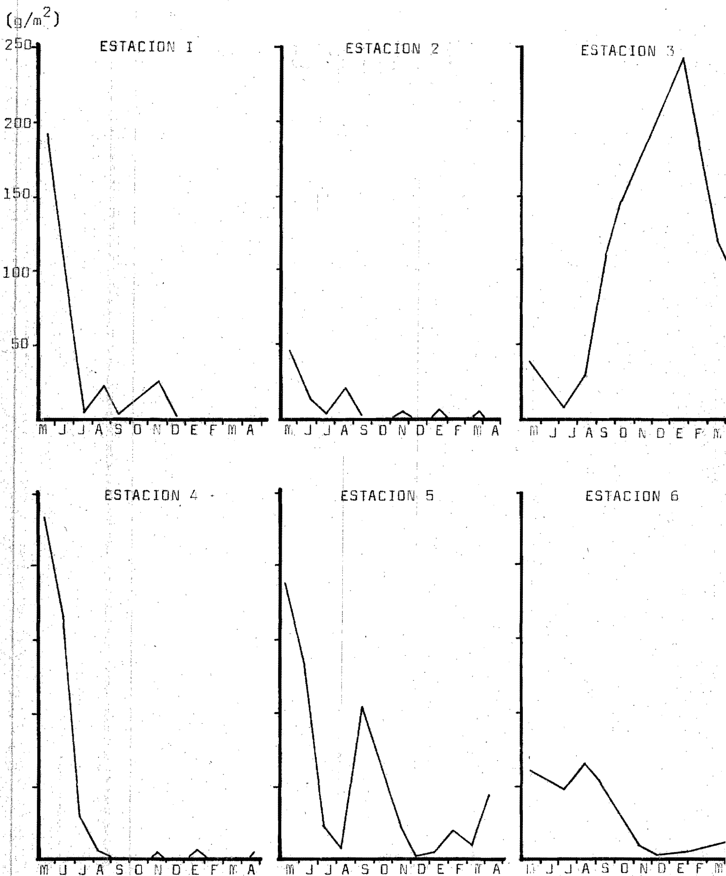
Fig. 9. Valores de productividad obtenidos para las seis estaciones de muestreo de los "manchones" de Ruppia . Los valores están dados en peso seco por metro cuadrado.
