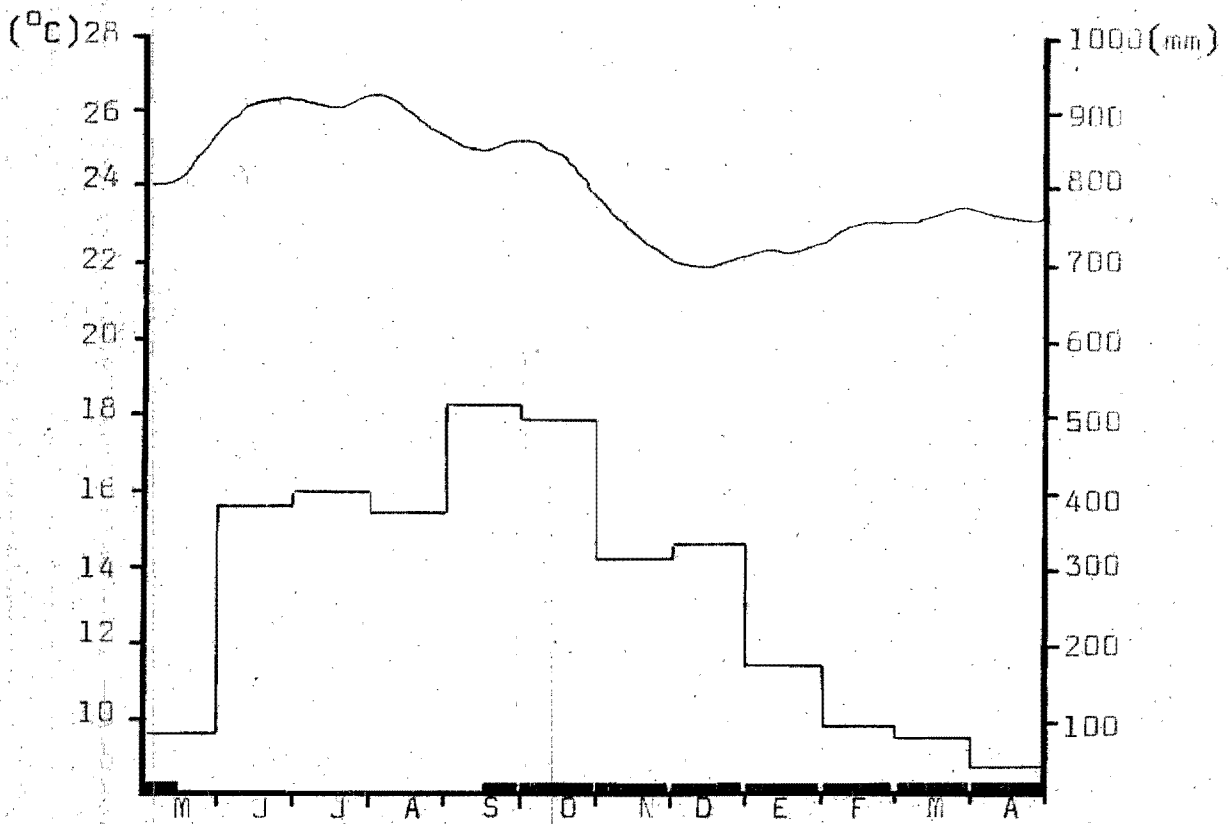
Fig. 2. Climograma de la Estación Meteorológica del Faro de Zapotitlán, Ver. En la parte inferior, las barras oscuras marcan la época de "nortes".
