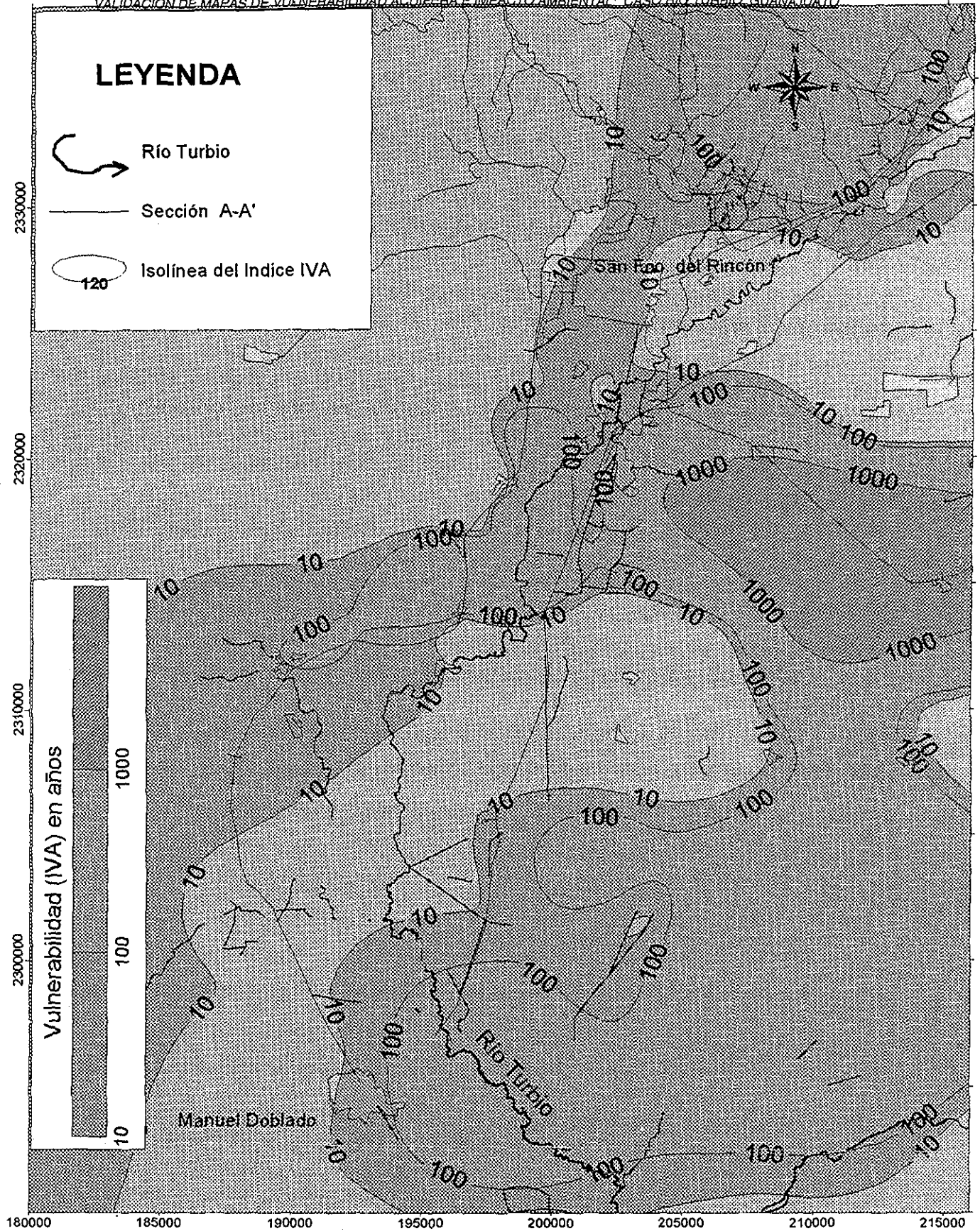
Figura 6.3 - Mapa del Índice de Vulnerabilidad de Acuíferos (AVI) en años en el Valle del Río Turbio. Valores mayores a 1000 años se ubican al oriente del valle en donde se encuentran paquetes arcillosos. Los valores menores a 10 años se asocian a rocas fracturadas y paquetes con conglomeráticos.
