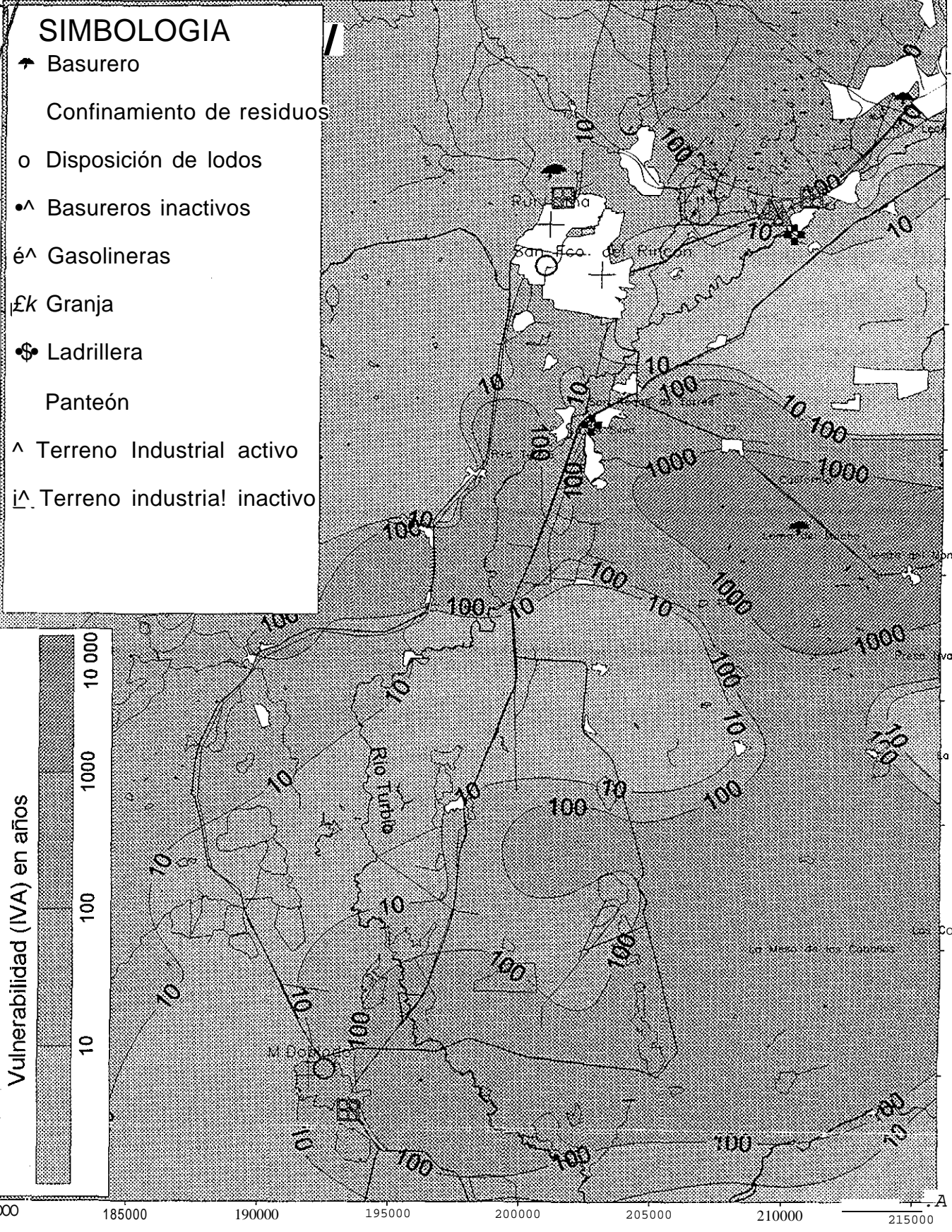
Figura 7,2- Mapa de riesgo al acuífero, basado en el método de vulnerabilidad AVI. La principal fuente contaminante lo constituye el Río Turbio, en su trayecto atraviesa zonas de alta vulnerabilidad
