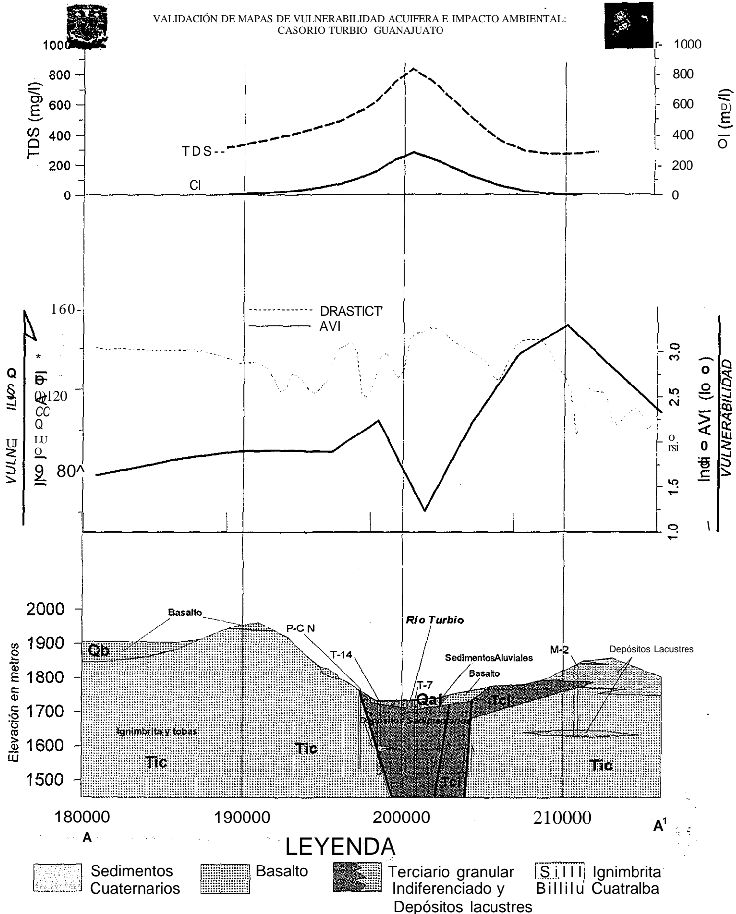
Figura 6,6- Comparación entre las secciones geológica, de vulnerabilidad, e hidrogeoquímicas en el Valle del Río Turbio,
