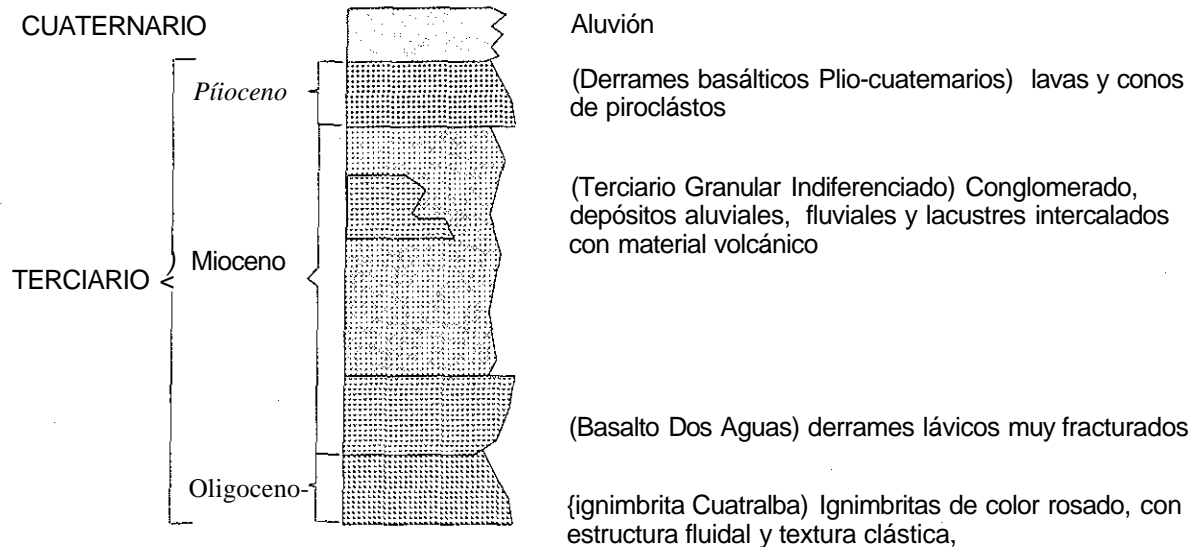
Figura 4.1.- Columna estratigráfica en el Valle del Río Turbio
