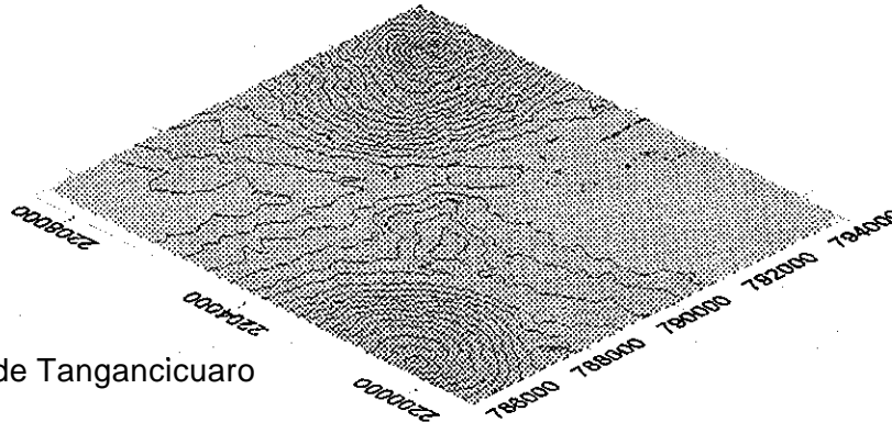
Figura 3 1 Comparación entre mapas morfométricos, topografía y vulnerabilidad de acuíferos (DRASTIC) en el área de Tangancicuaro
