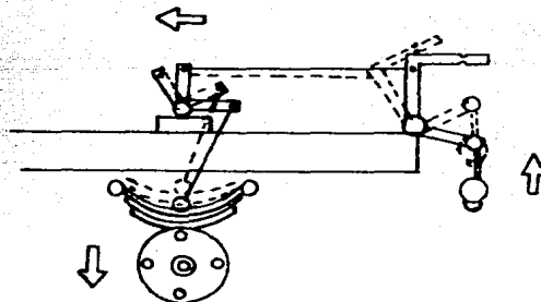
MECANISMO PARA MANTENER UNIFORME LA ALTURA DE LA BARRA DE RIEGO.
