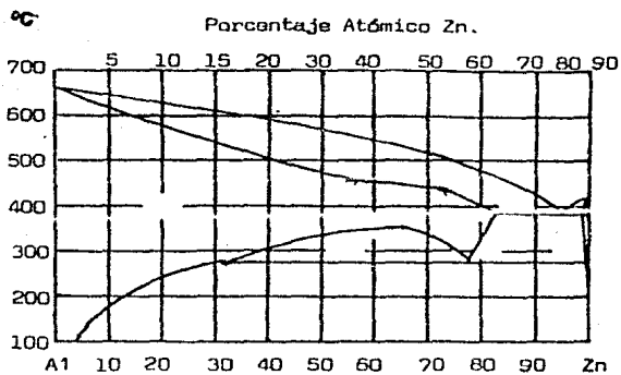
Fig. 37 Diagrama de Equilibrio Al-Zn.
