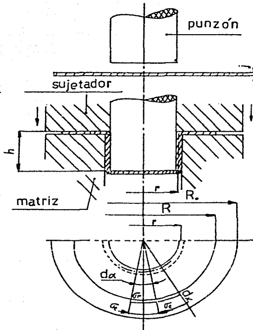
Fig. 48.- Gráfico en el cual se considera un elemento de chapa sometido a la acción de las fuerzas exteriores producidas durante el embutido.
