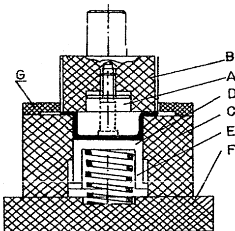
Fig. 46.- Esquema de una estampa sencilla para embutir.
