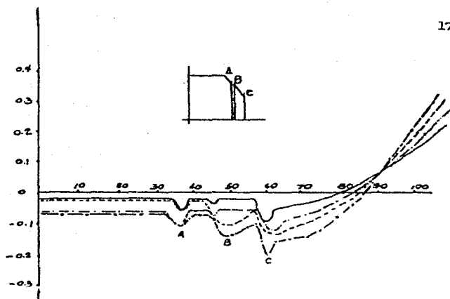
Fig. 60. Efecto de la fuerza del sujetador de cospel, P_1 , en la distribución de esfuerzos en el espesor, en la 1a. y 2a. etapa de empuje. ——— 1a. etapa P_1 = 54.12 \text{ KN} -.-.-. 1a. etapa P_1 = 82.24 \text{ KN} ——— 2a. etapa P_2 = 32.42 \text{ KN} -o-o- 2a. etapa P_2 = 32.42 \text{ KN} .
