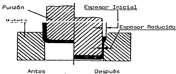
Fig. 62.- Método de embutido para utensilios de fondo grueso.
