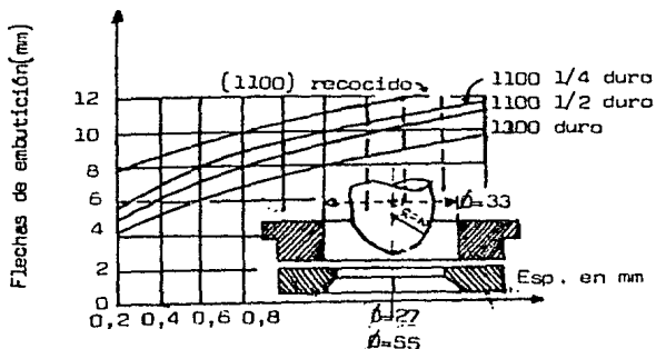
Fig. 34 Flechas de embutición Erichsen para el (1100) en distintos espesores. Recocido-1/4 duro-1/2 duro (obtenidos por acritud parcial sobre metal recocido).
