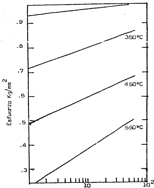
Fig. 31 Efecto de la velocidad de deformación sobre la tensión necesaria para comprimir Al hasta una reducción de 40% en alto ( \epsilon = -0.51 ), a varias temperaturas.
