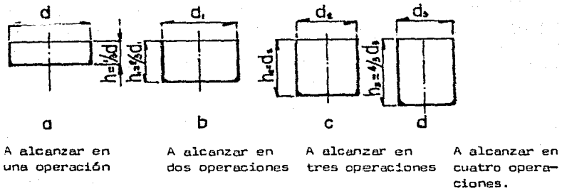
Fig. 51.- Número de las operaciones necesarias con relación a la profundidad del embutido (para piezas de grandes dimensiones)
