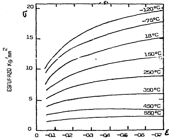
Fig. 30 Curvas tensión-deformación para el Al a varias temperaturas, obtenidas con un plastómetro a leva, a velocidad de deformación de 4.38/seg.
