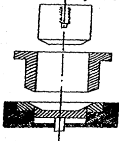
Fig. 57.- Matriz de embutido, punzón, sujetador interior y botador.
