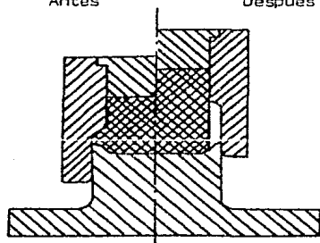
Fig. 64.- Formación de rebordes en la pared en embutido de recipientes.
