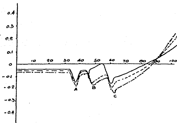
Fig. 61 Efecto de la fuerza P_2 de la camisa del punzón en la distribución de esfuerzos en el espesor en la segunda etapa.
