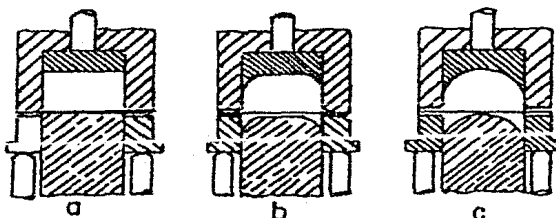
Fig. 53.- Embutido en una etapa (a) Punzón con perfil de radio pequeño; (b) Punzón con perfil de radio grande. (c)-Punzón de cabeza hemisférica.
