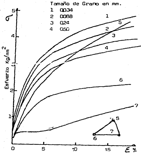
Fig. 28 Efecto del tamaño de grano sobre las curvas de tracción de Al puro.
