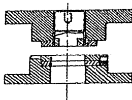
Fig. 56.- Matriz Plana de embutido por empuje, con punzón y sujetador exterior, pero sin los cortantes.
