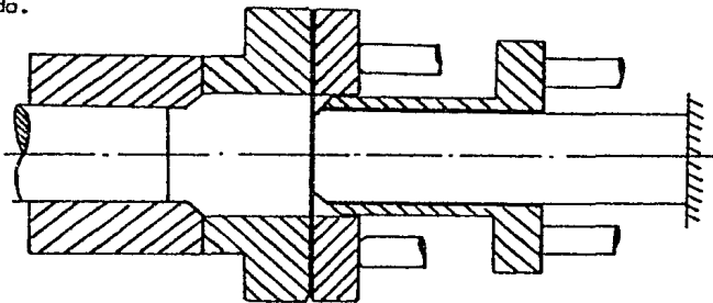
Fig. 59.- Diagrama esquemático de la herramienta.
