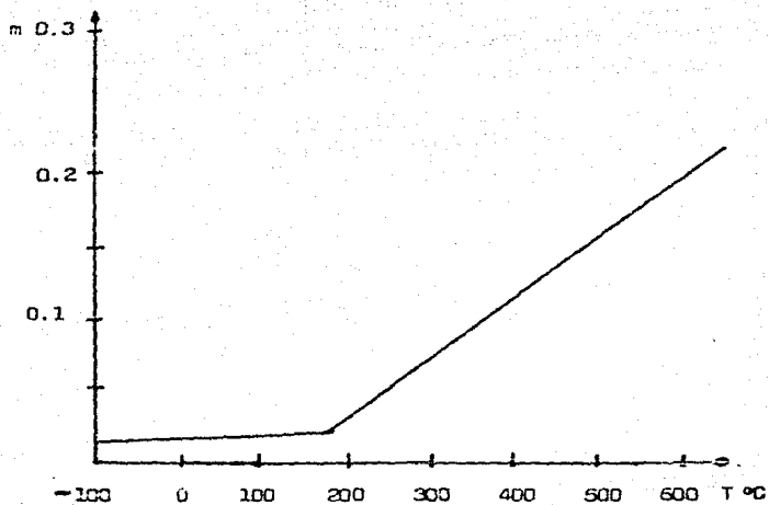
Fig. 29 Variación del coeficiente de sensibilidad a la velocidad de deformación con la temperatura.
