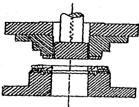
Fig. 55.- Matriz de embutido con punzón, sujetador exterior y filos cortantes.
