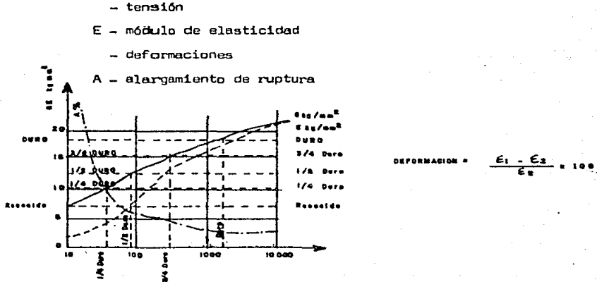
Fig. 32 Curva de acritud del aluminio (1100) por trefilado o laminación en frío.
