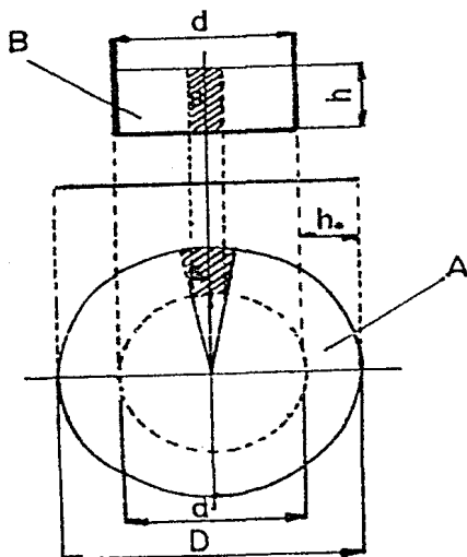
Fig. 47.- Demostración práctica de la deformación que ha experimentado el material de un recipiente embutido.
