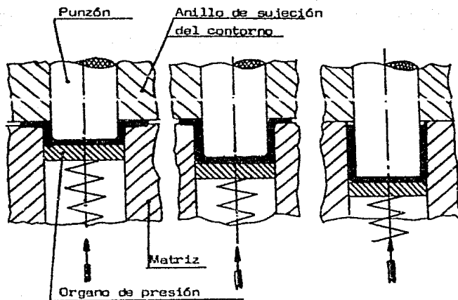
Fig. 43.- Algunas fases durante la operación de embutido.
