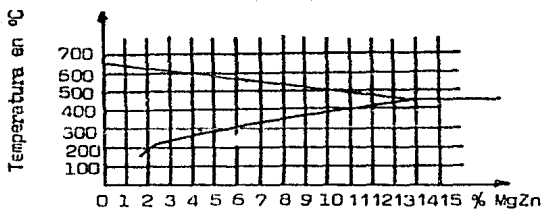
Fig. 38 Diagrama de Equilibrio Al-MgZn.
