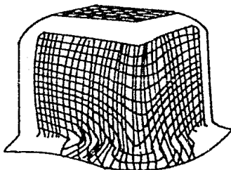
Fig. 42.— Demostración gráfica del alargamiento de las fibras en las paredes de un recipiente embutido.
