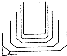
Fig. 54.- Pasos Típicos en embutido, reembutado y dimensionamiento.
