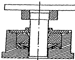
Fig. 58.- Matriz para dimensionamiento de acción simple.
