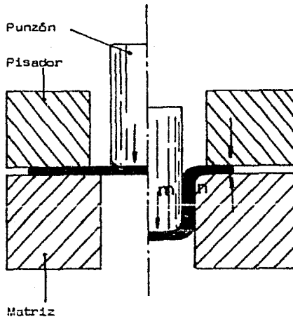
Fig. 44.- Embutido con pisador plano.
