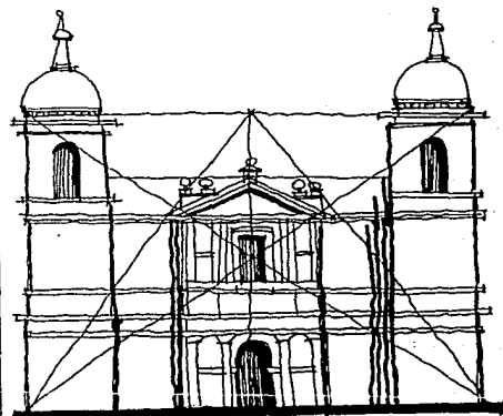
Fachada Principal de la catedral de Valladolid. Proyecto de Juan de la Herrera. (Estudio de Proporciones).
