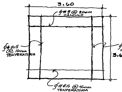
PLANTA-
