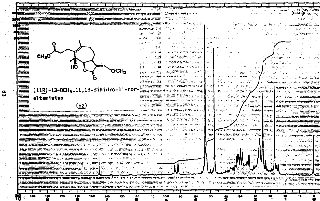
espectro 7
