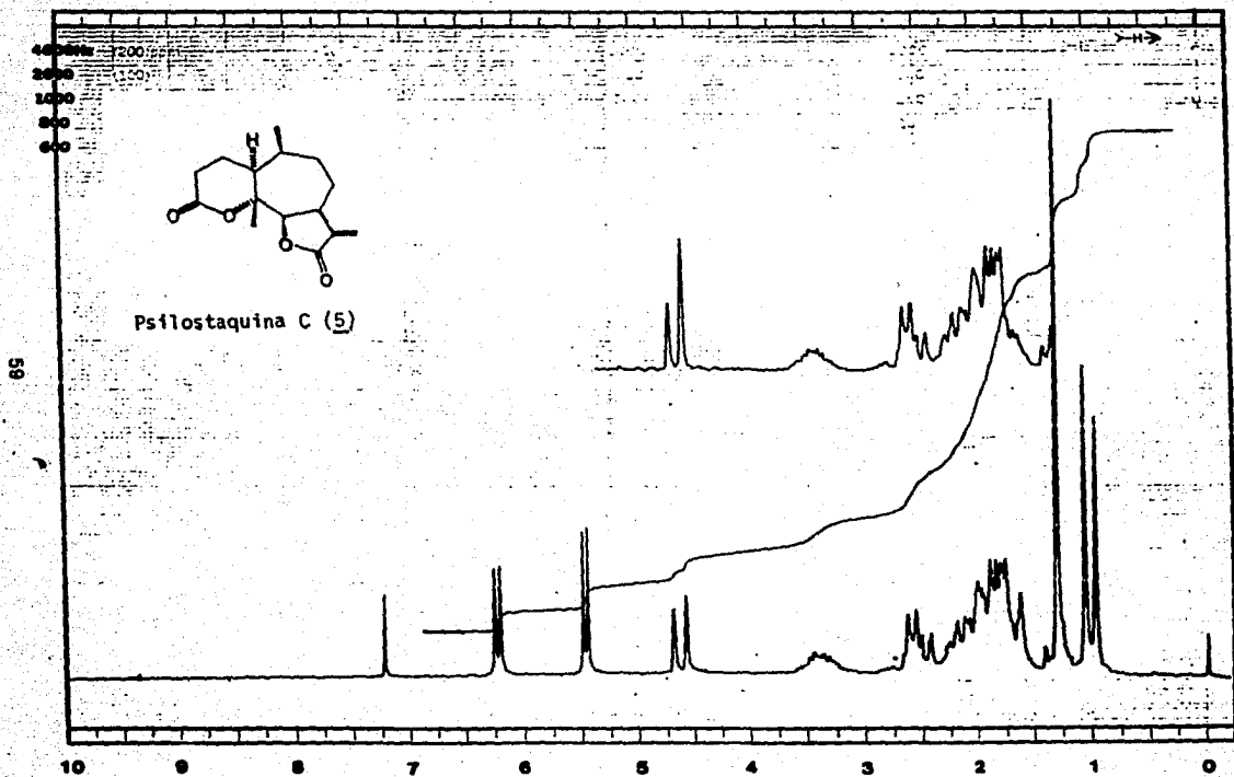
espectro 3
