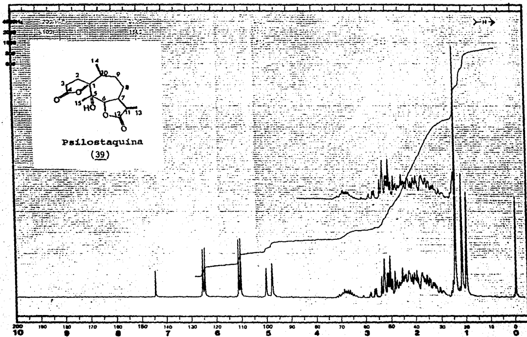
espectro 1
