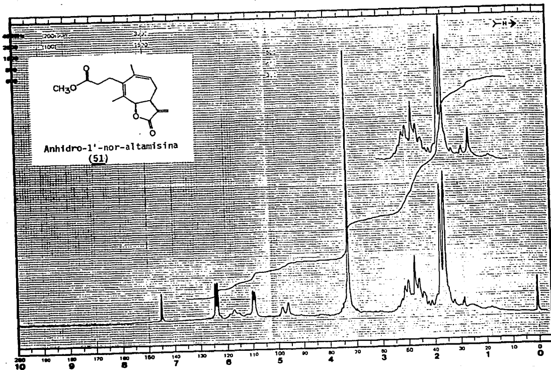
espectro 6
