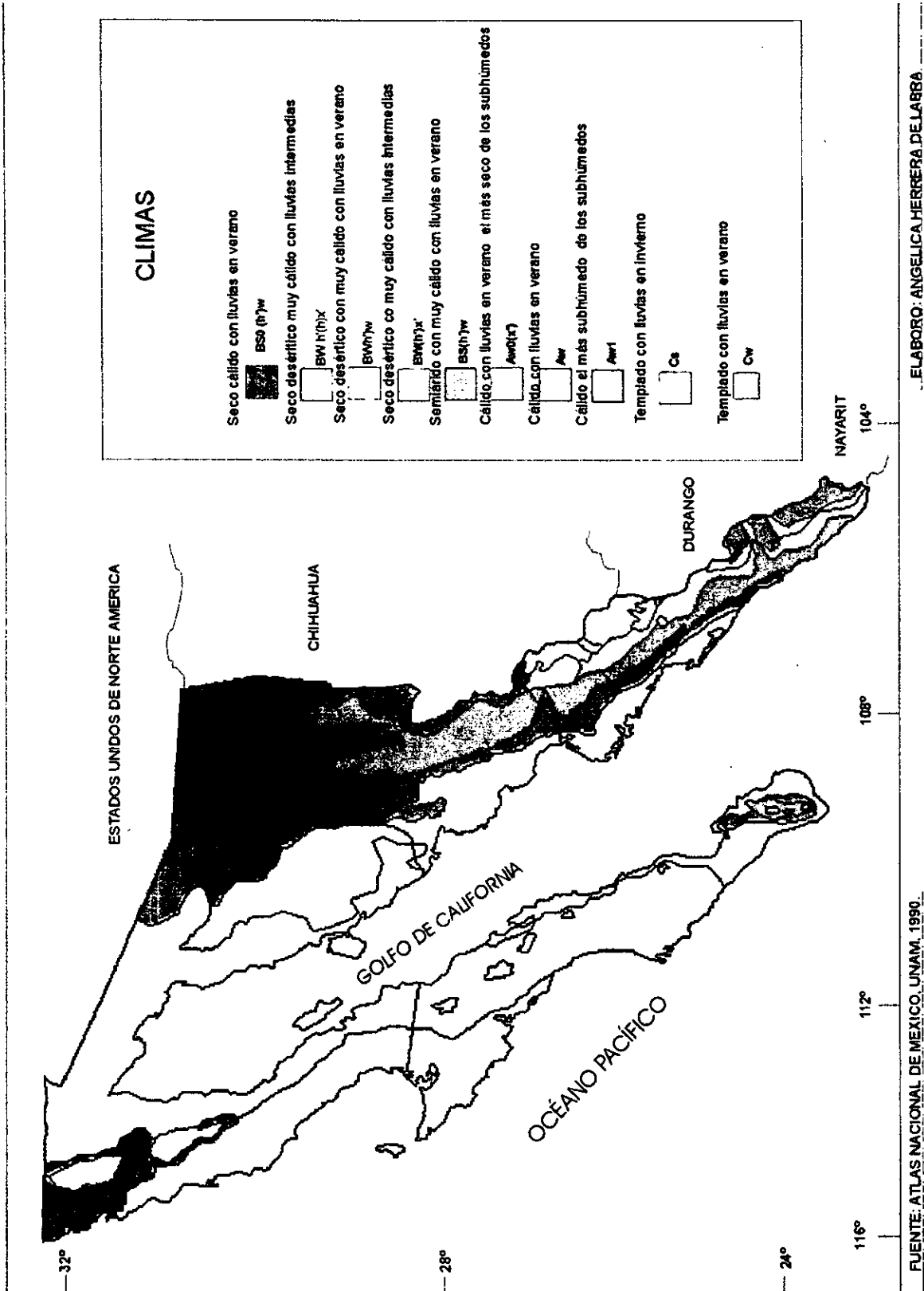
FIGURA 1.5 DISTRIBUCION CLIMATICA DE LA REGION COSTERA DEL NOROESTE DE MEXICO
