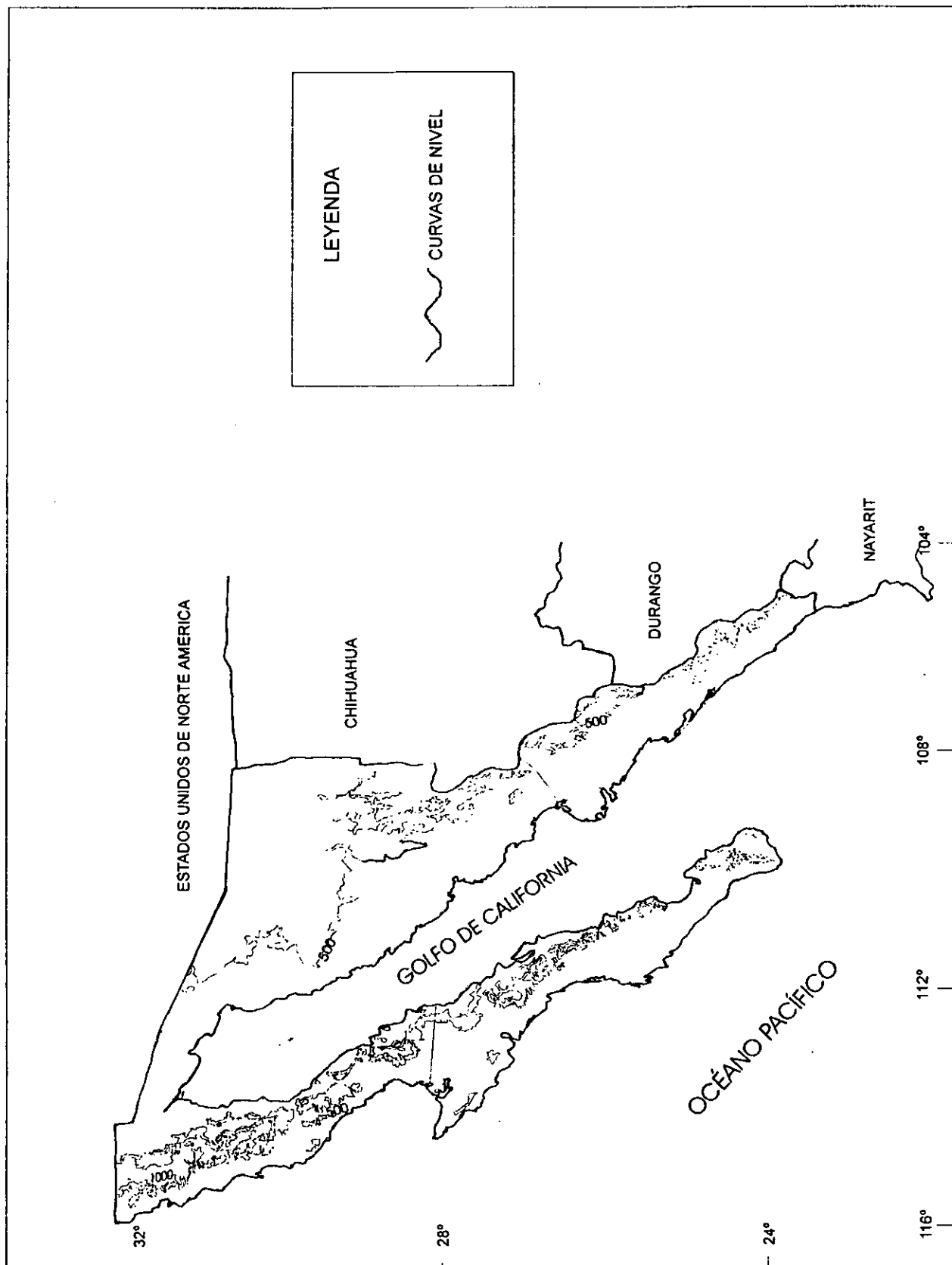
FIGURA 1.4 TOPOGRAFÍA DE LA REGIÓN COSTERA DEL NOROESTE DE MÉXICO
