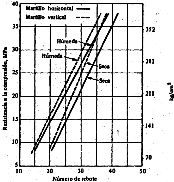
FIG. IV. 6 RELACION ENTRE LA RESISTENCIA A LA COMPRESION DE LOS CILINDROS Y EL NUMERO DE REBOTE, PARA LECTURAS DE MARTILLO EN POSICION HORIZONTAL Y VERTICAL, SOBRE UNA SUPERFICIE DE CONCRETO HUMEDA Y SECA.
