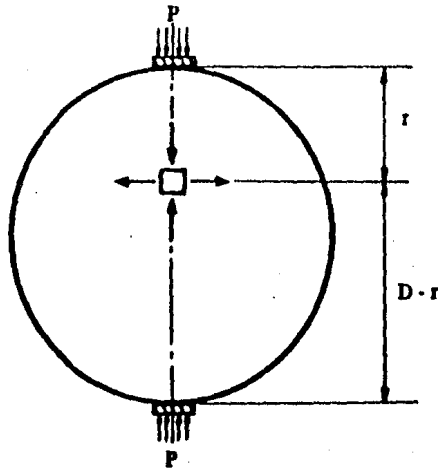
FIG. IV. 3 PRUEBA BRASILEÑA DE TENSION
