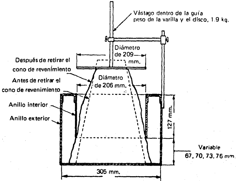
FIG. III. 4. APARATO PARA LA PRUEBA DE REMOLDEO.
