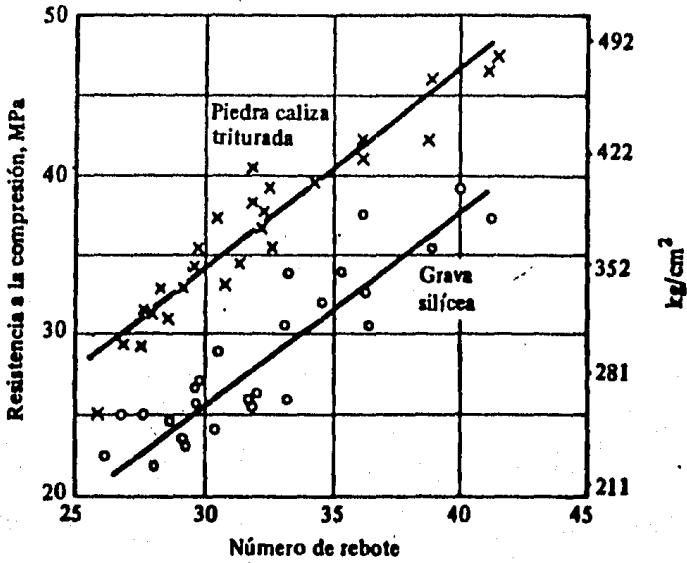
FIG. IV. 7 RELACION ENTRE LA RESISTENCIA A LA COMPRESION Y EL NUMERO DE REBOTE.
