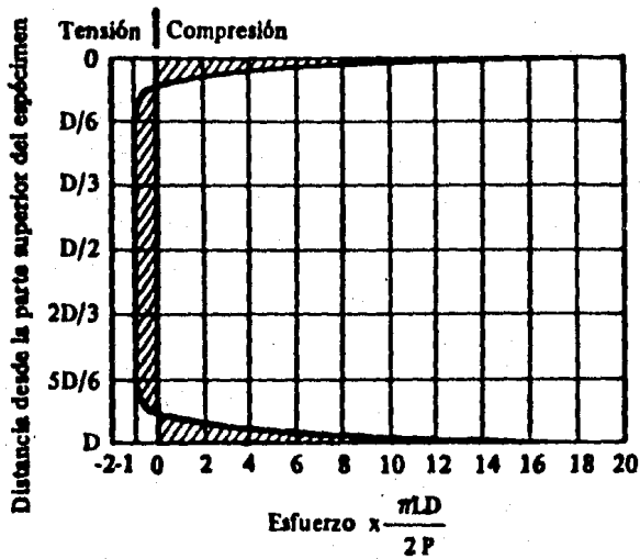
FIG. IV. 3 DISTRIBUCION DEL ESFUERZO HORIZONTAL EN UN CILINDRO CARGADO SOBRE UN ANCHO IGUAL A 1/12 DEL DIAMETRO
