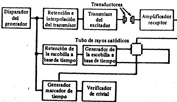
FIG. IV. 9 ESQUEMA DEL APARATO DE PULSO ULTRASONICO.
