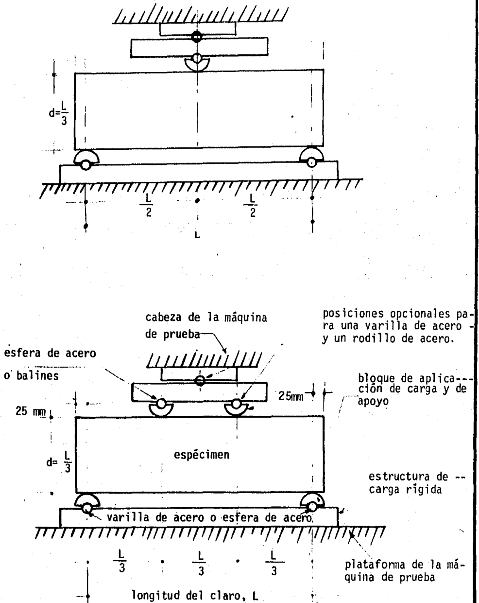
FIG. IV.1 EQUIPO PARA ENSAYAR A FLEXION POR EL METODO DE CARGA EN LOS TERCIOS Y AL CENTRO DEL CLARO
