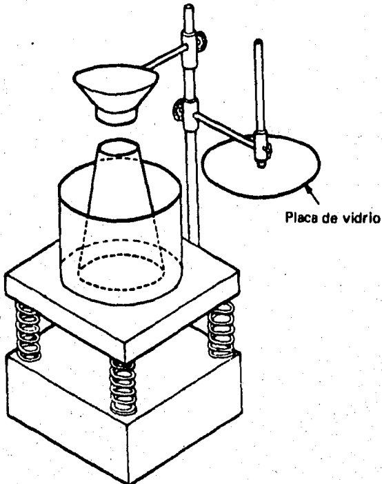
FIG. III. 4. APARATO PARA LA PRUEBA DE REMOLDEO.
