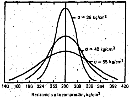
FIG. V. 2 CURVAS NORMALES DE FRECUENCIA.
