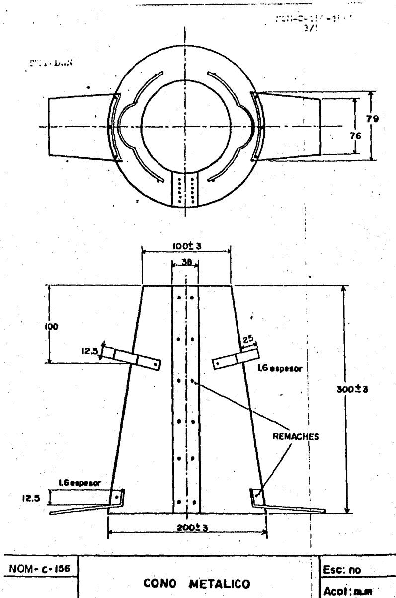
FIG. III.1 EQUIPO PARA LA OBTENCIÓN DEL REVENIMIENTO
