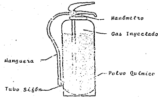
EXTINGUIDOR DE POLVO QUIMICO
