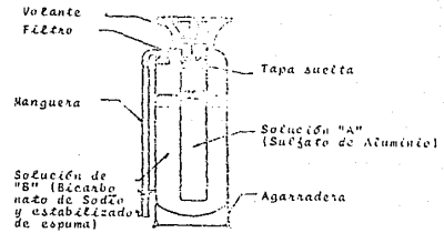
EXTINGUIDOR DE ESPUMA QUIMICA
