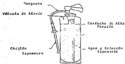
EXTINGUIDOR DE ESPUMA MECANICA
