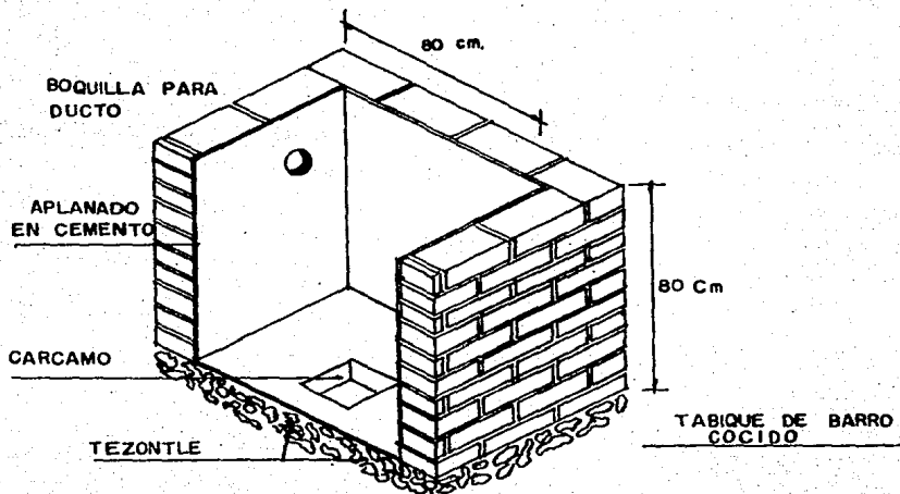
CORTE A-A EN PERSPECTIVA
