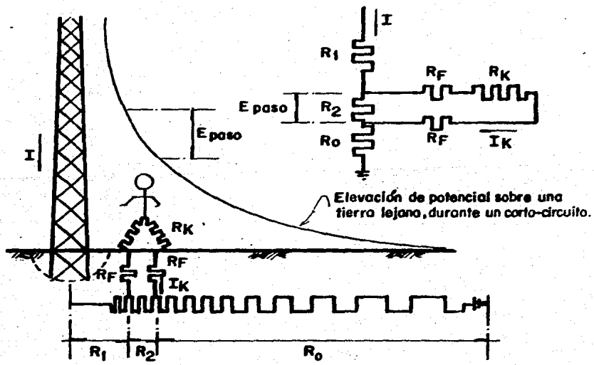
Tensiones de paso, cerca de una estructura conectada a tierra .
