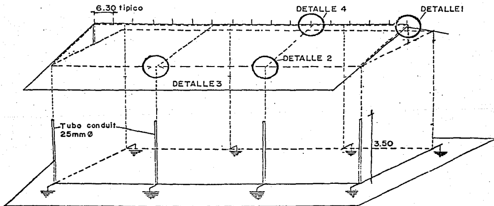
DISTRIBUCION DE MALLA DE PARARRAYOS EN LAS NAVES
