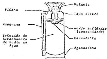
EXTINGUIDOR DE SODA-ACIDO
