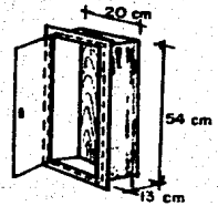
REGISTRO DE DISTRIBUCION ALIMENTACION O DE PASO
