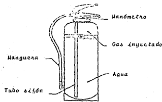
EXTINGUIDOR DE AGUA
