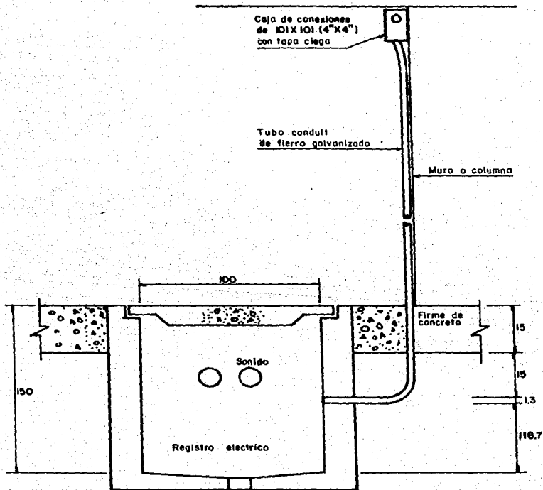
DETALLE DE SALIDA DEL DUCTO DEL VOCEO DEL REGISTRO ELECTRICO
