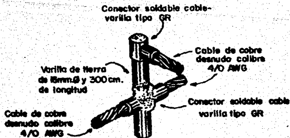
DETALLE 4 (b)
