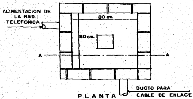
REGISTRO DE BANQUETA
