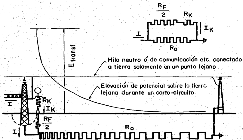
Ejemplo del peligro librado a potenciales transferidos .
