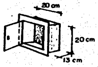
REGISTRO DE DISTRIBUCION
