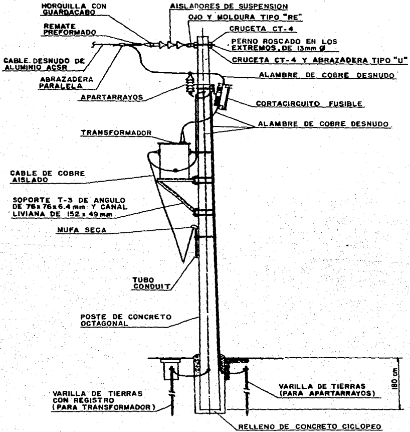
SUBESTACION TIPO POSTE
