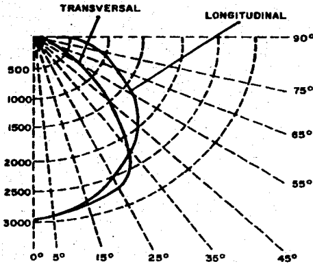
CURVA DE DISTRIBUCION EN CANDLE POWER
