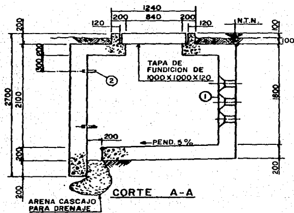
REGISTRO PARA ALTA TENSION
