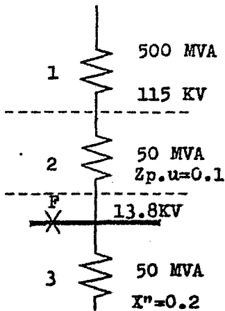
DIAGRAMA DE IMPEDANCIAS
