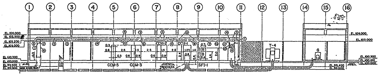
ELEVACION CORTE "A-A"
