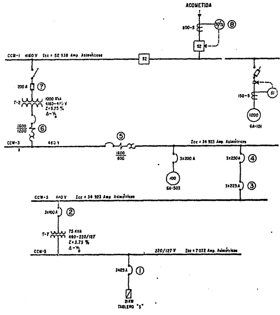
DIAGRAMA UNIFILAR SIMPLIFICADO DE LA TRAYECTORIA SELECCIONADA
