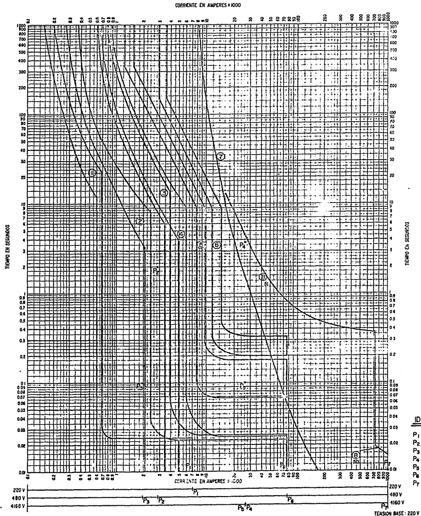
CURVAS DE DISPARO
