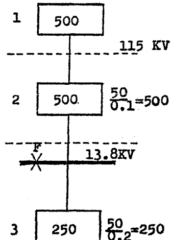
DIAGRAMA DE LOS MVA'S
