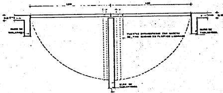
DETALLE DE ABATIMIENTO DE PUERTAS EN ACCESO A C.M.F. 1/5
